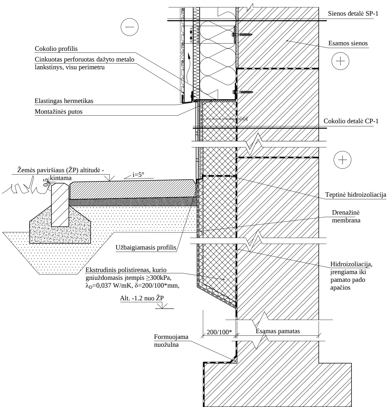
PRINCIPINĖ COKOLIO DETALĖ CD-1/CD-1* M 1:10
