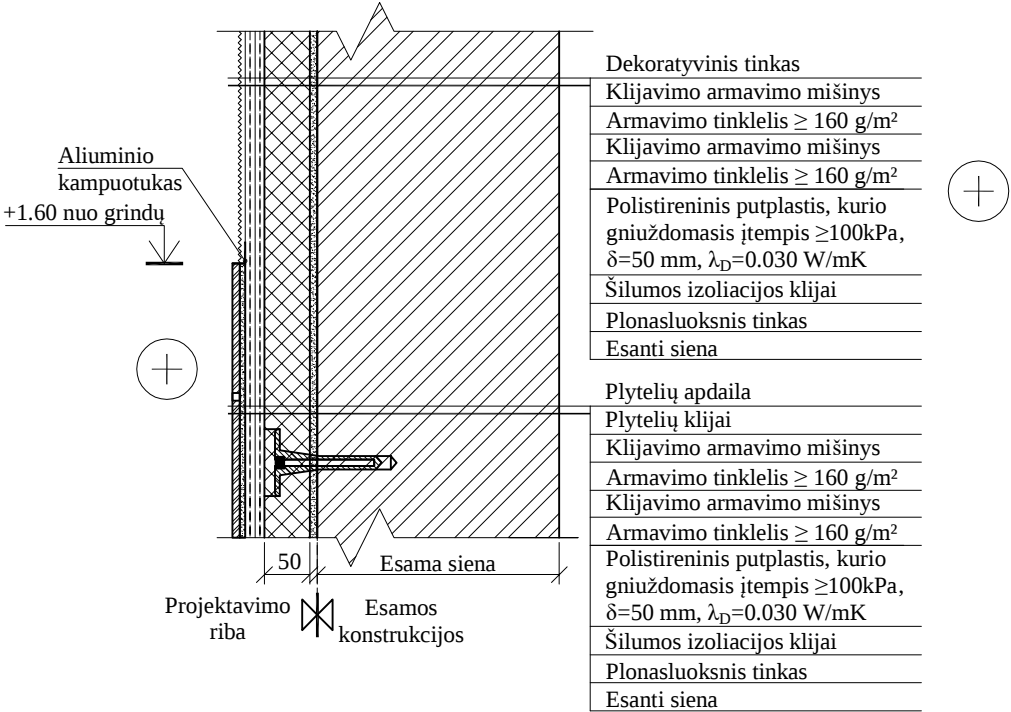
SIENOS DETALĖ SP-5 M 1:10
