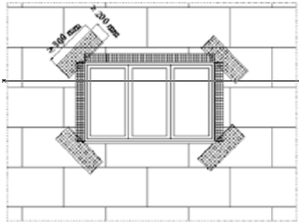
ANGOKRAŠČIŲ KAMPŲ ARMAVIMAS
