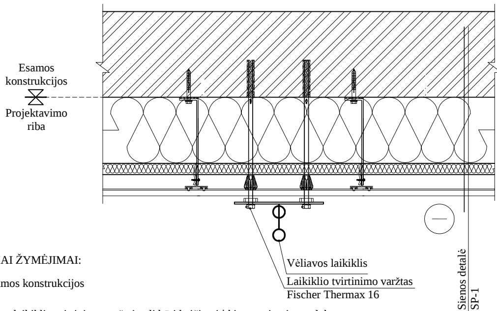
PJŪVIS 1-1 M 1:10
