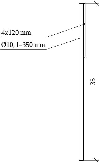
METALO JUOSTA POZ.1 M1:5
