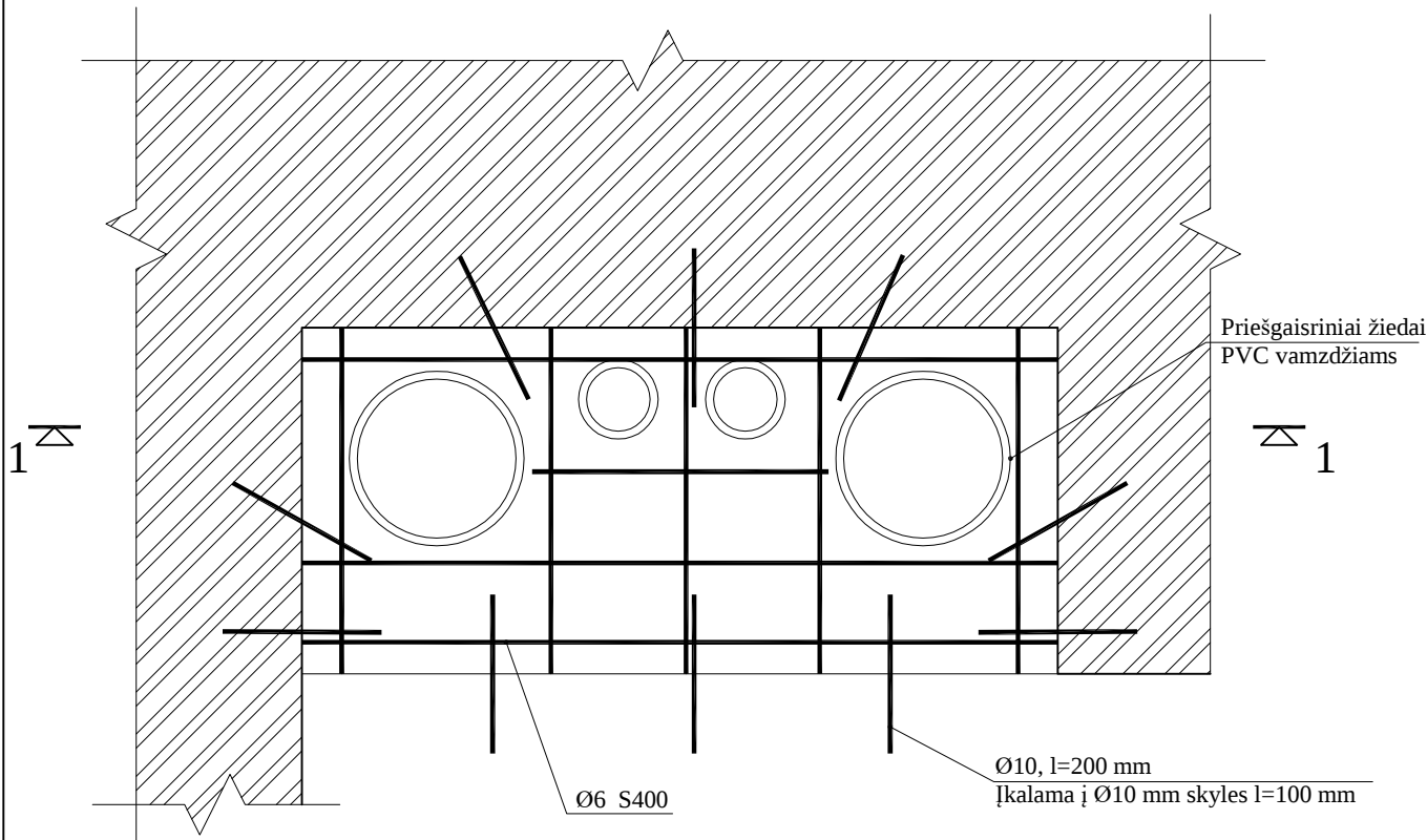
PJŪVIS 1-1
