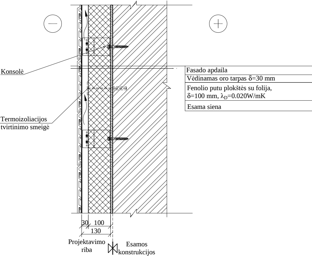
SIENOS DETALĖ SP-2 M 1:10
