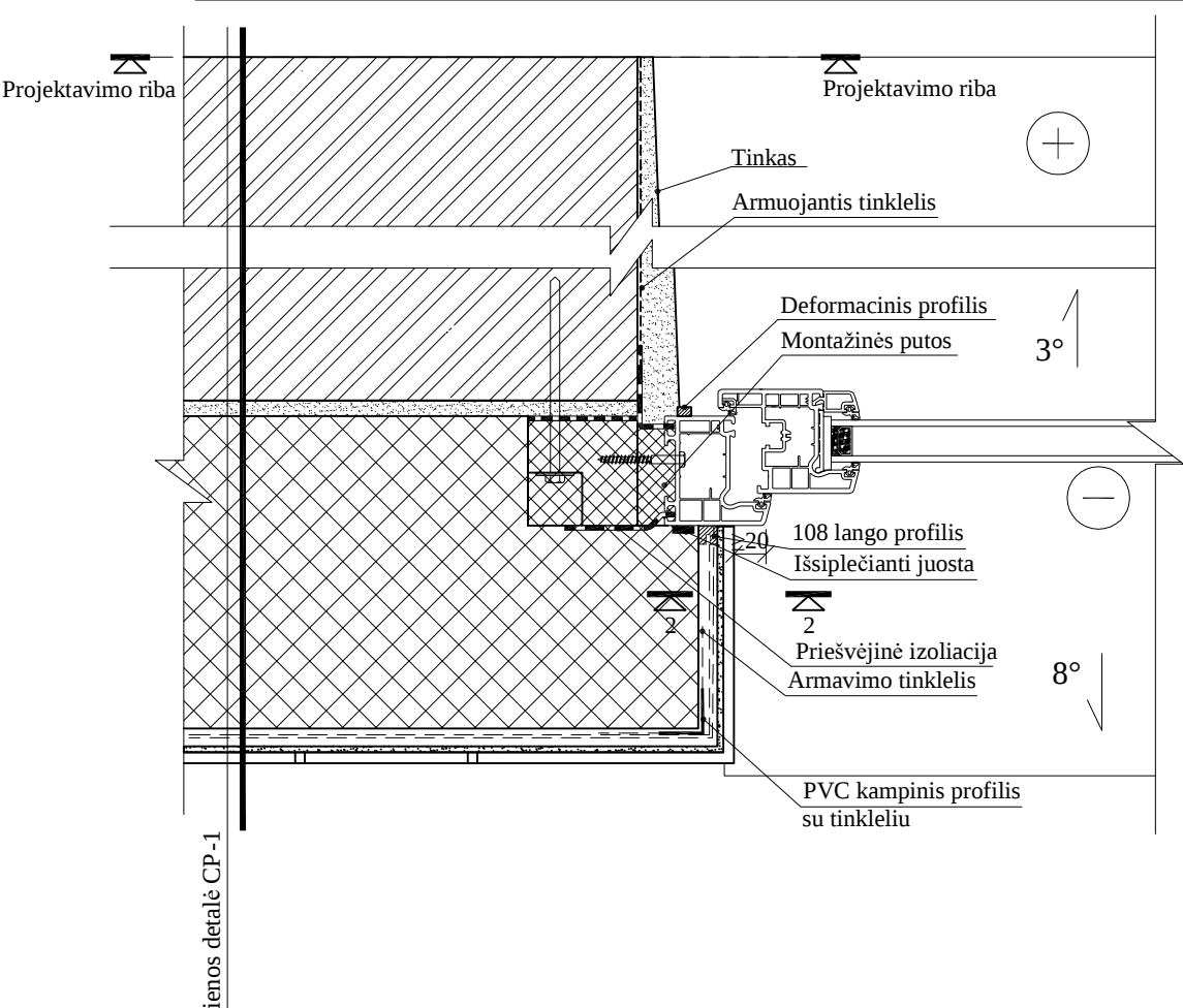
RŪSIO LANGO ŠONINIO ANGOKRAŠČIO ĮRENGIMO DETALĖ M 1:5
