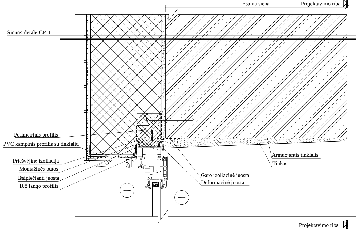
RŪSIO LANGO APATINIO ANGOKRAŠČIO ĮRENGIMO DETALĖ M 1:5
