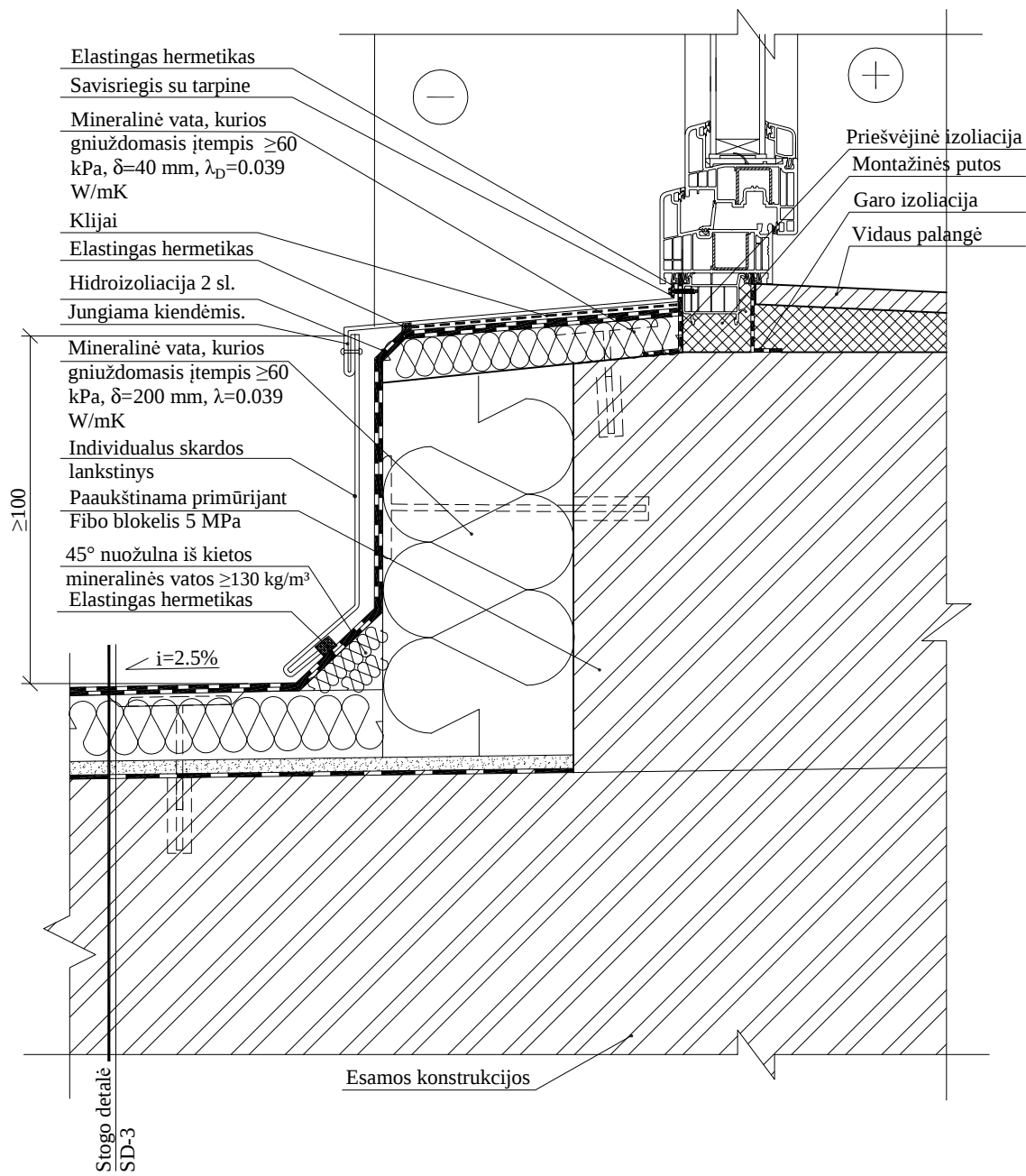
STOGELIO SU LAIPTINĖS LANGO ANGOKRAŠČIU SUJUNGIMO DETALĖ M 1:5
