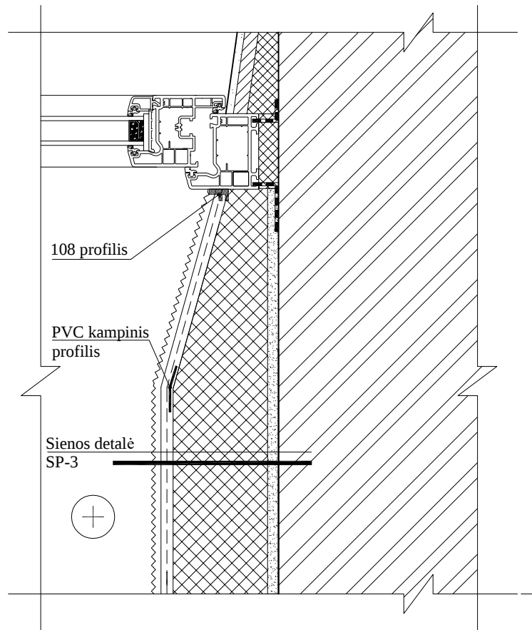
BALKONŲ VIDAUS STKLINIMŲ ANGOKRŠAČIŲ APŠILTINIMO DETALĖ M 1:5
