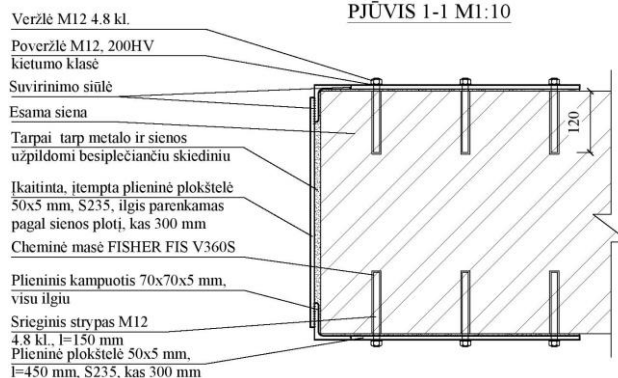
PJŪVIS 1-1 M1:10
