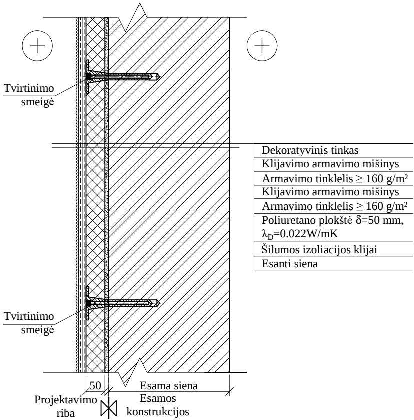
SIENŲ DETALĖ SP-4 M 1:10
