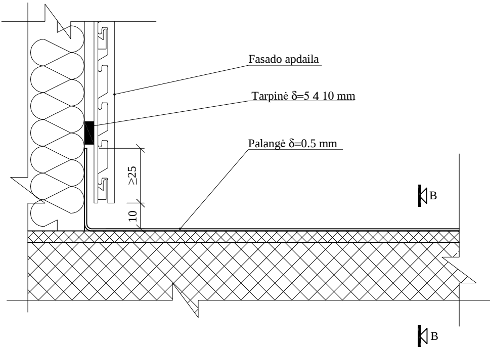
PJŪVIS "A-A" M 1:2
