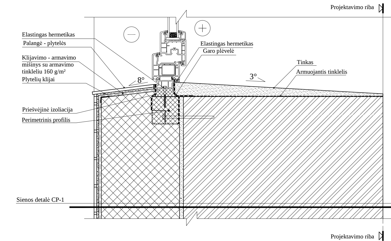
RŪSIO LANGO APATINIO ANGOKRAŠČIO ĮRENGIMO DETALĖ M 1:5
