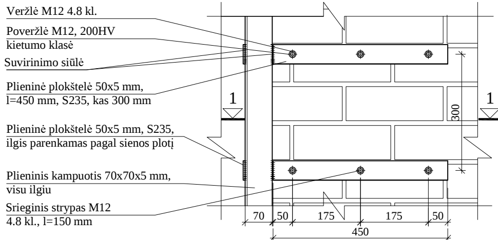
PJŪVIS 1-1 M1:10
