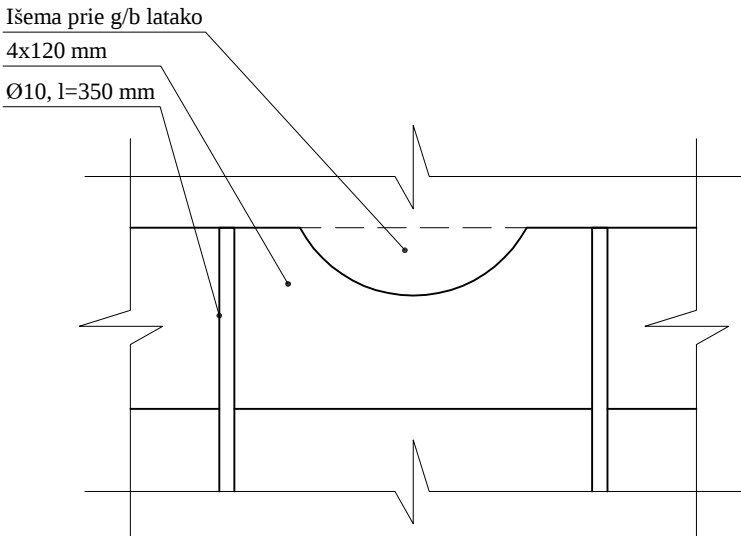
PJŪVIS 1-1 M1:5
