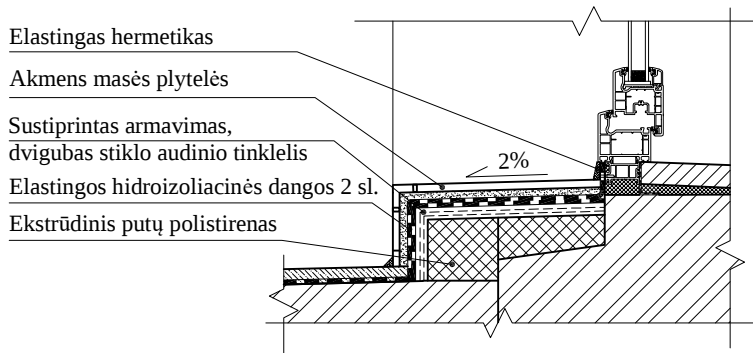
BALKONO DURŲ APATINIO ANGOKRAŠČIO DETALĖ M 1:10
