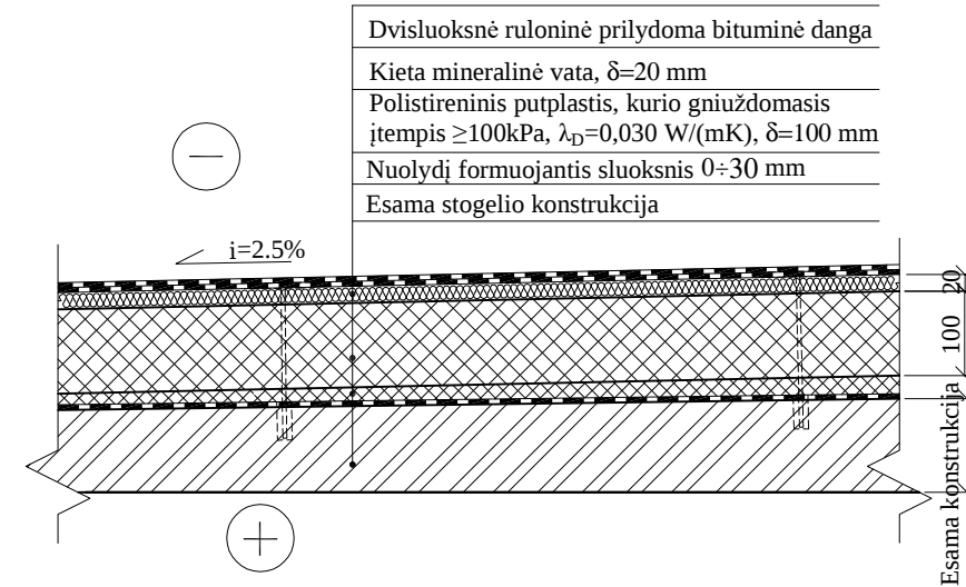
VIRŠUTINIO AUKŠTO BALKONŲ STOGELIŲ APŠILTINIMO DETALĖ SD-2 M 1:10
