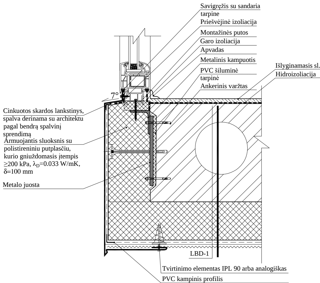
LODŽIŲ STIKLINIMO ĮRENGIMO DETALĖ M 1:5
