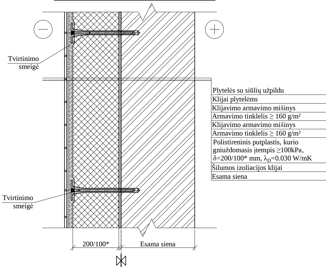
COKOLIO DETALĖ CP-1/CP-1* M 1:10
