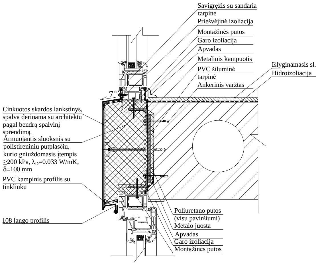
LODŽIŲ STIKLINIMO ĮRENGIMO DETALĖ M 1:5
