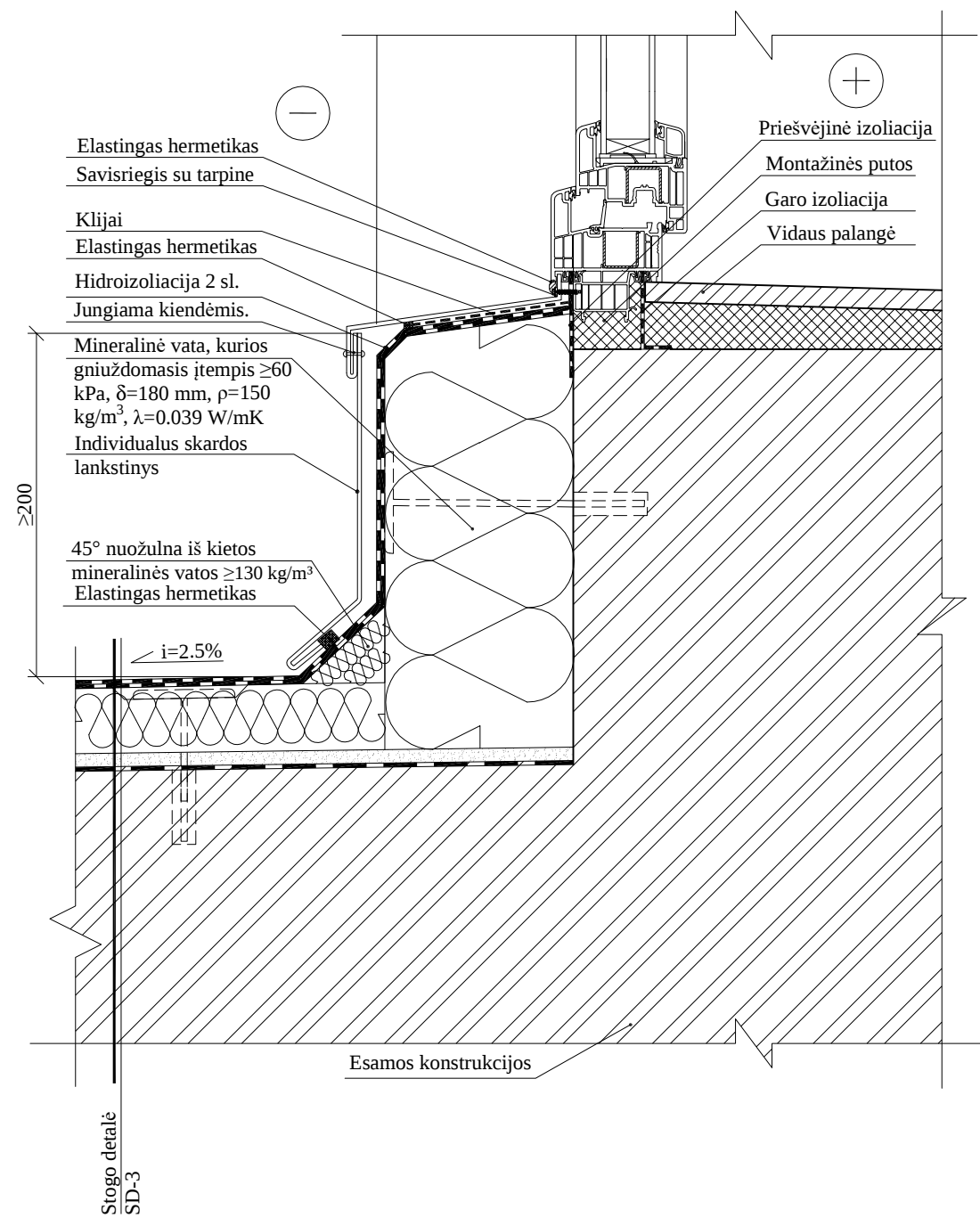
STOGELIO SU LAIPTINĖS LANGO ANGOKRAŠČIU SUJUNGIMO DETALĖ M 1:5
