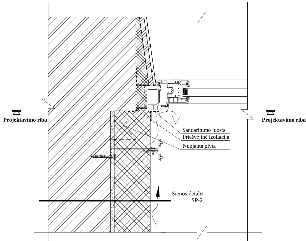
LAIPTINIŲ LANGŲ ŠONINIO ANGOKRAŠČIO ĮRENGIMO DETALĖ M 1:5
