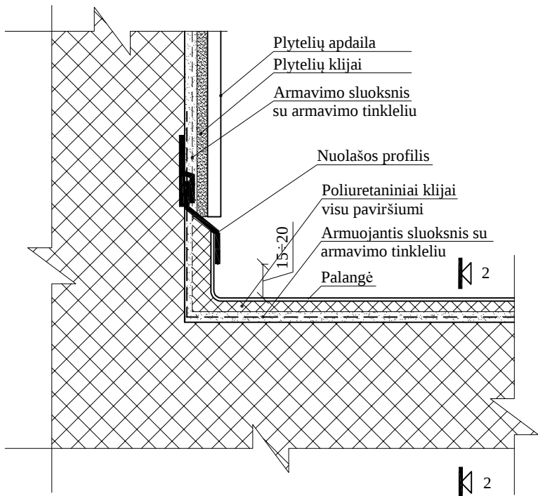
PJŪVIS "2-2" M 1:2
