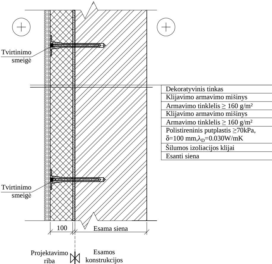
SIENŲ DETALĖ SP-3 M 1:10
