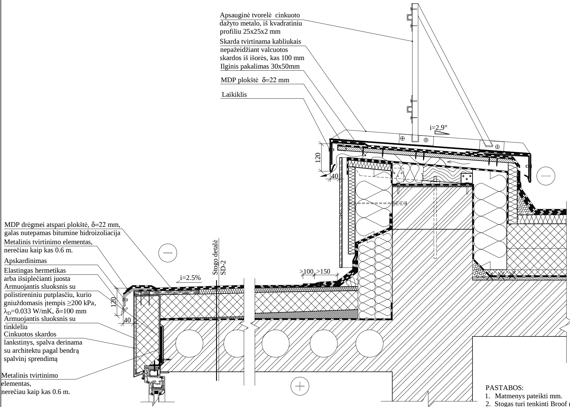
LODŽIJŲ STOGELIO SU PARAPETU SUJUNGIMO DETALĖ M 1: 10
