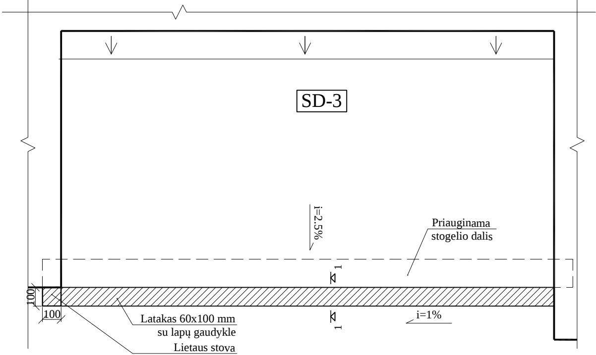
ĮĖJIMO STOGELIO PLANAS M 1:20
