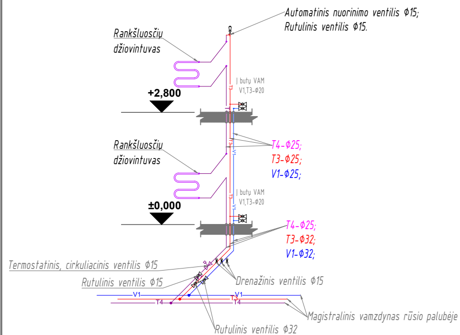
V1; T3; T4 SISTEMŲ TIPINIS STOVAS ST.-1 ... ST.-6.
