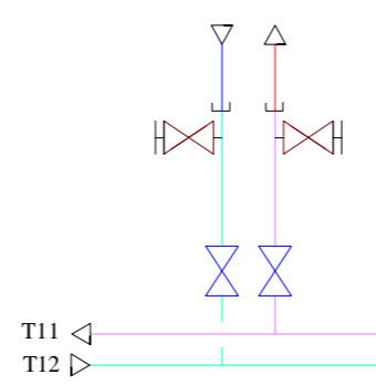
Stovų 29, 32, 35, 38, 41 ir 44 balansavimo uždarymo mazgas
