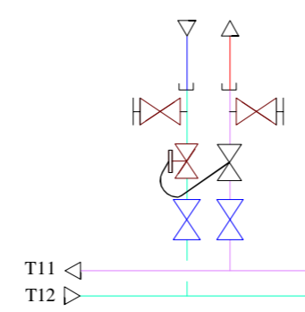
Stovų, išskyrus 29, 32, 35, 38, 41 ir 44 balansavimo uždarymo mazgas
