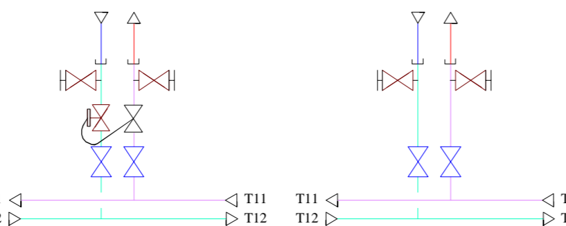
Stovų, išskyrus 29, 32, 35, 38, 41 ir 44 balansavimo uždarymo mazgas
