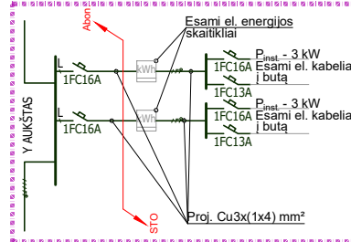
Rekonstruojami AS-2-Y el. skydai (kur Y-1...11, iš viso 11 vnt.)
