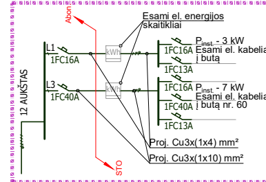
Rekonstruojami AS-2-12 el. skydas
