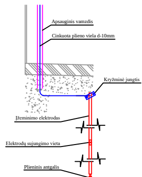
Giluminio įžemintuvo fragmentas
