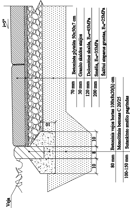
NUOGRINDOS ĮRENGIMO DETALĖ DD-5 M 1:10
