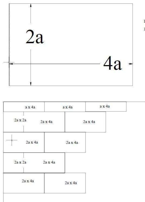
2 pav. Pirmojo termoizoliacinio sluoksnio klojimo schema
