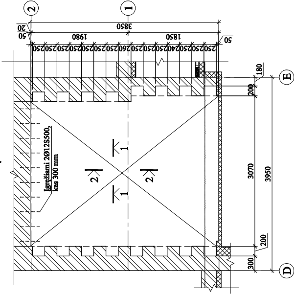
LAIPTINĖS STOGELIO TARP D-E AŠIŲ KONSTRUKCIŲ PLANAS M 1:50
