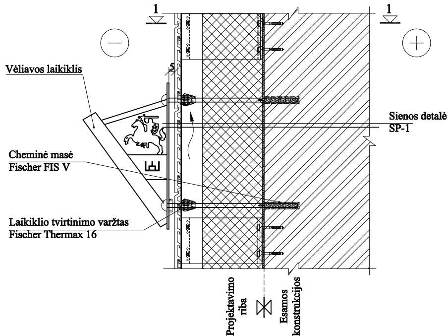
PJŪVIS 1-1 M 1:10
