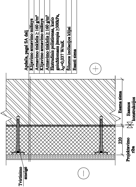
COKOLIO DETALĖ CP-1 M 1:10
