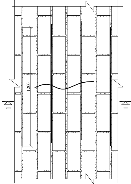
SIENOS ĮTRŪKIMŲ SUTVARKYMO ARMATŪRINIAIS STRYPAIS SCHEMA. KAI TVARKOMAS VIENAS PLYŠYS M1:10
