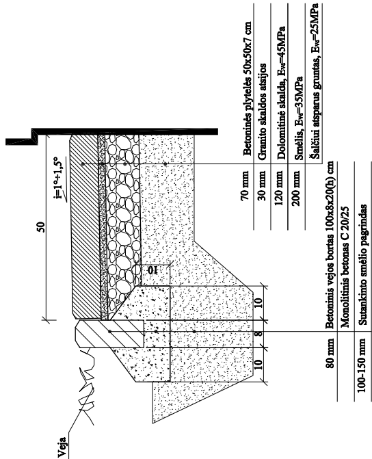
NUOGRINDOS ĮRENGIMO DETALĖ DD-1 M 1:10
