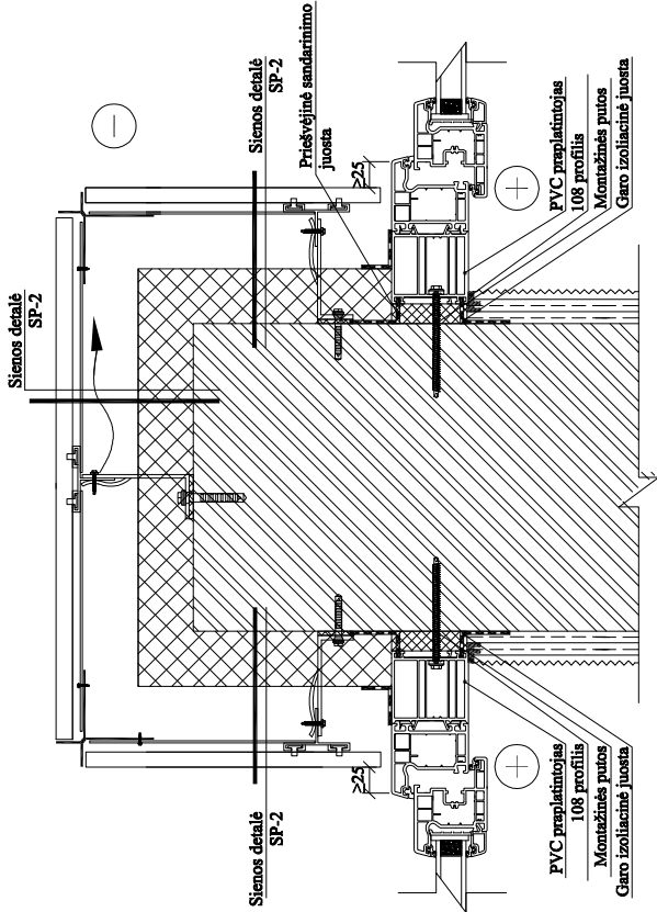
PVC LODŽIŲ STIKLINIMO ŠONINIO ANGOKRAŠČIO SU PRAPLATINTOJU ĮRENGIMO DETALĖ SM-3 M 1:5
