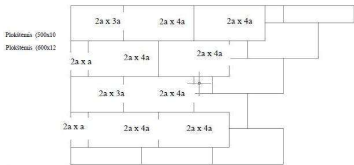
3 pav. Antrojo termoizoliacinio sluoksnio klojimo schema
