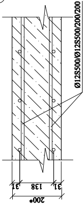
PJŪVIS 2-2 M 1:10
