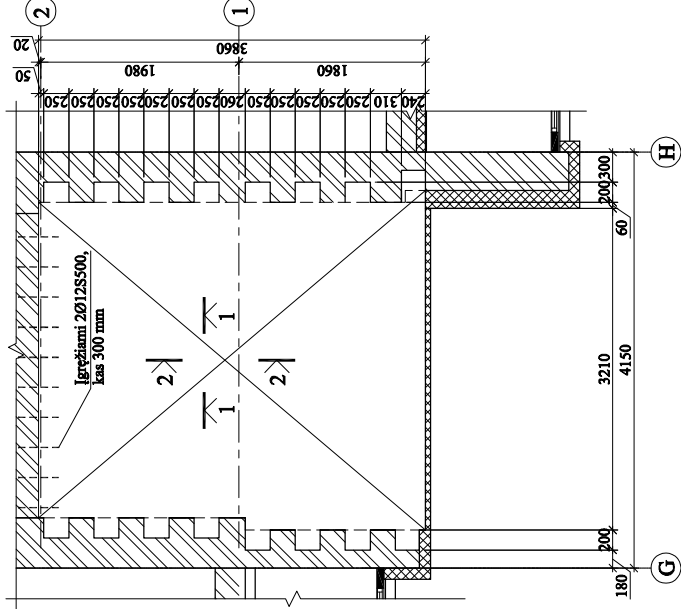
LAIPTINĖS STOGELIO TARP G-H AŠIŲ KONSTRUKCIŲ PLANAS M 1:50
