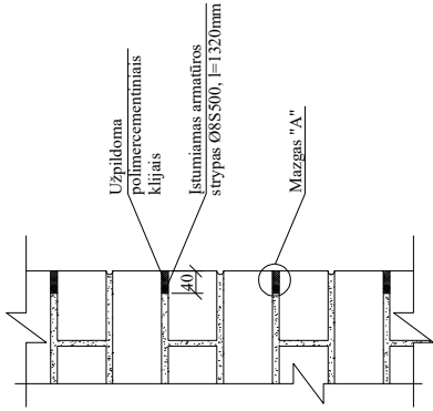
PIŪVIS 1-1 M1:10
