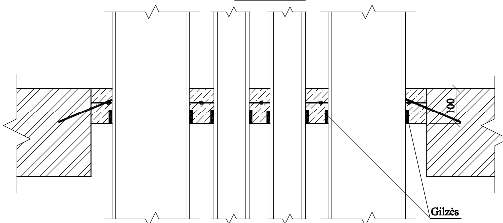
PJŪVIS 1-1
