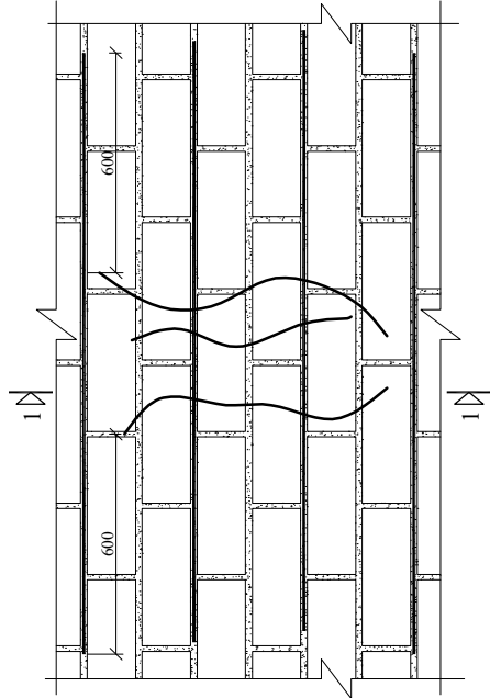
SIENOS ĮTRŪKIMŲ SUTVARKYMO ARMATŪRINIAIS STRYPAIS SCHEMA, KAI PLYŠIŲ DAUGIAU NEI VIENAS M1:10
