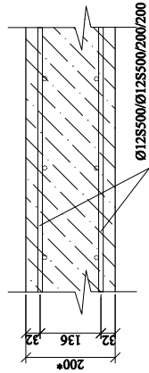
PJŪVIS 1-1 M 1:10
