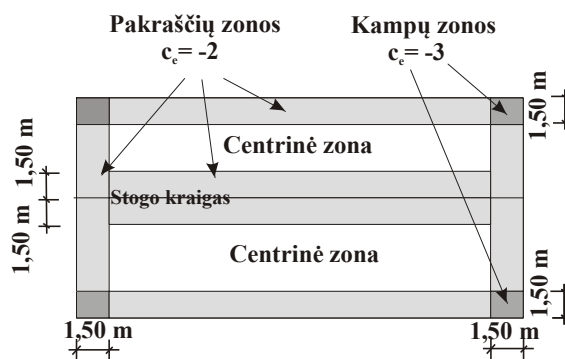
10 paveikslas. Principinė stogo suskirstymo į zonas schema
