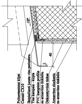
PJŪVIS "2-2" M 1:2
