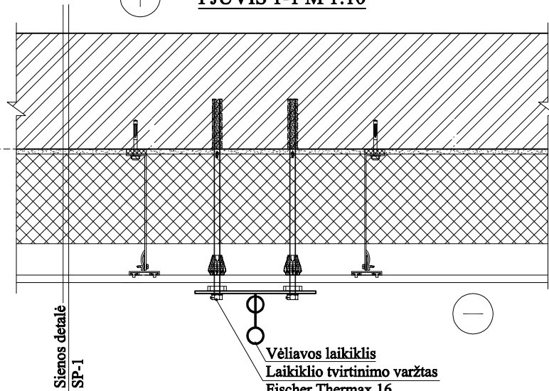
PJŪVIS 1-1 M 1:10
