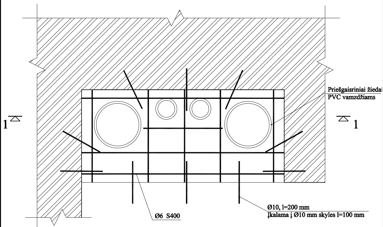
PJŪVIS 1-1
