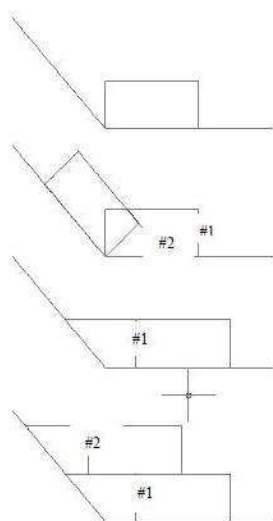
4 pav. Šilumos izoliacijos plokščių supjaustymas ir išdėstymas nelygiuose stogo kampuose
