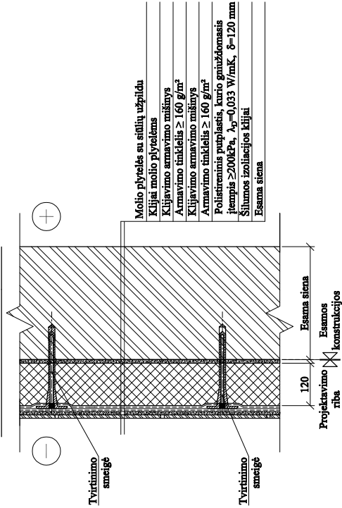
SIENOS DETALĖ SP-3 M 1:10
