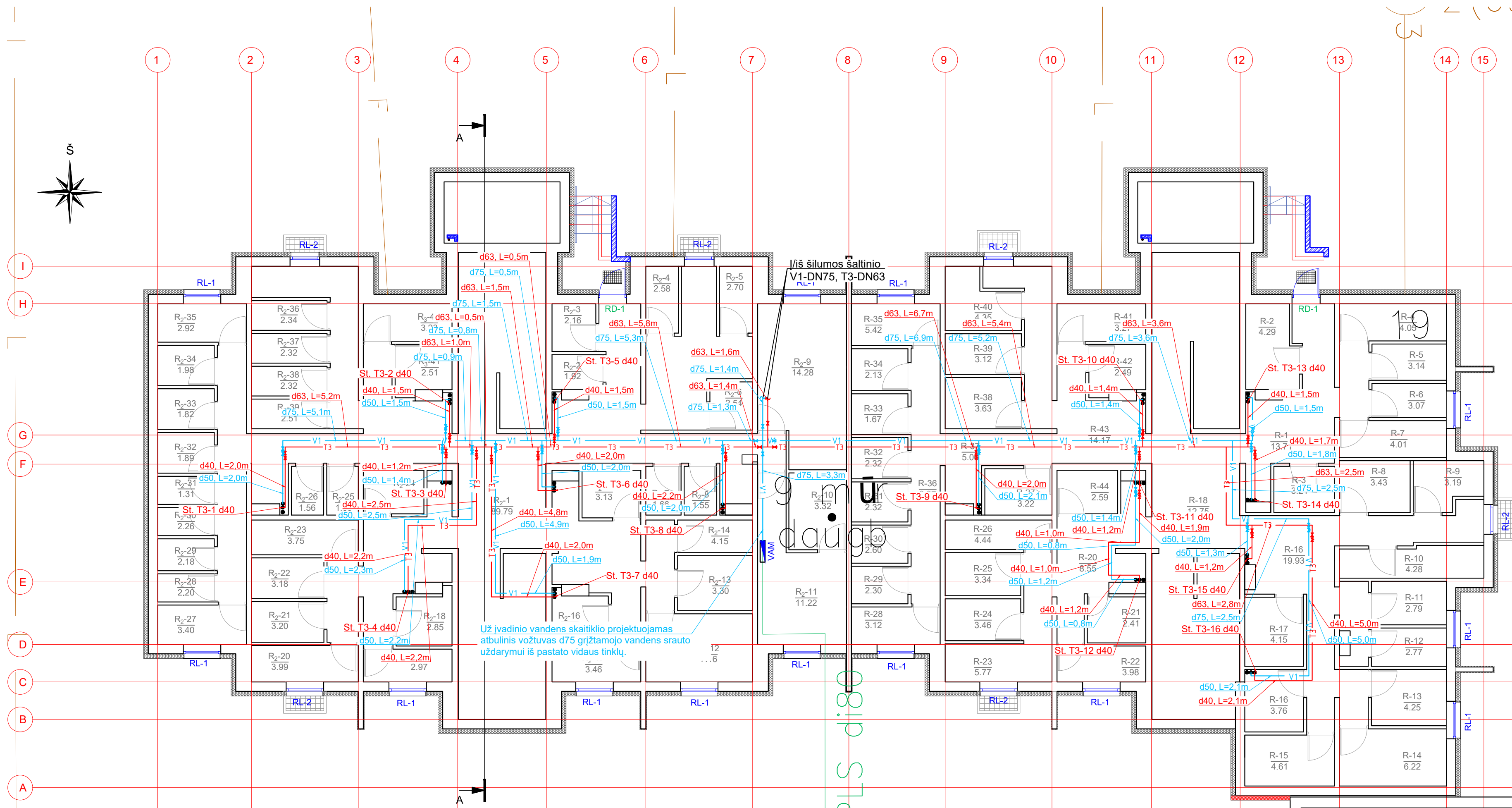
RŪSIO PLANAS M 1:100
