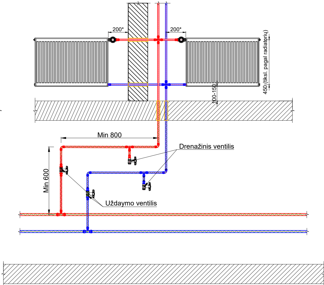
TIPINIS DVIGUBO STOVO APRIŠIMAS
