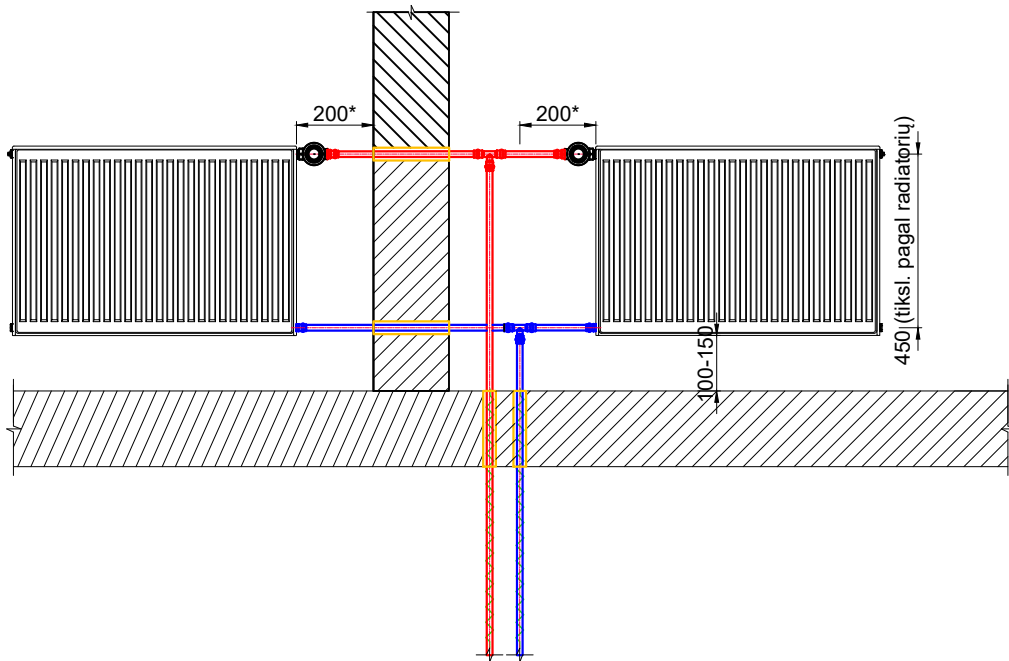
KETVIRTO AUKŠTO DVIGUBO STOVO ĮRENGIMO SCHEMA
