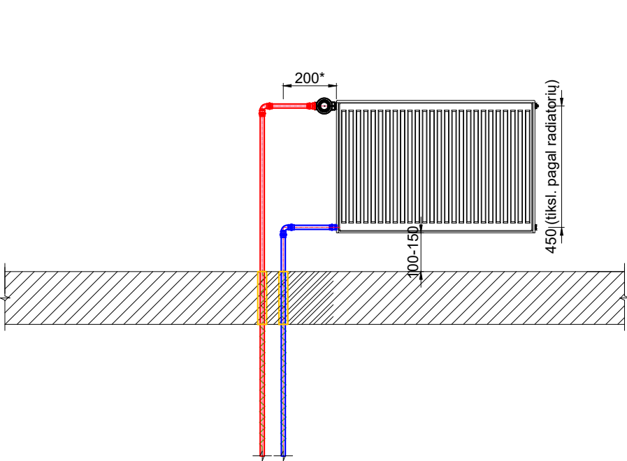
KETVIRTO AUKŠTO VIENGUBO STOVO ĮRENGIMO SCHEMA
