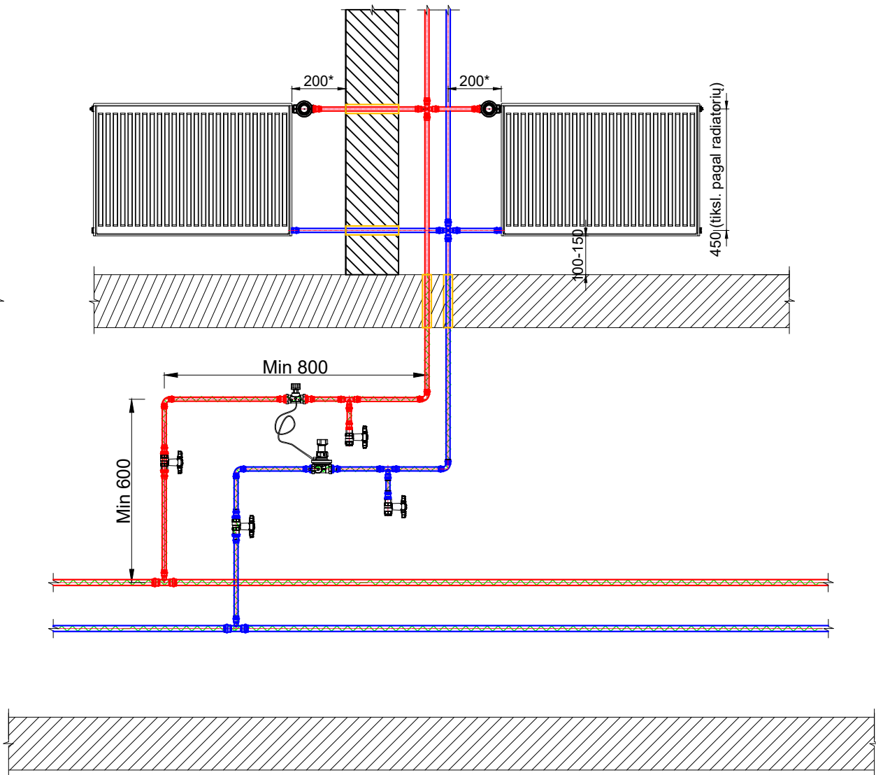
TIPINIS DVIKUBO STOVO APRIŠIMAS
