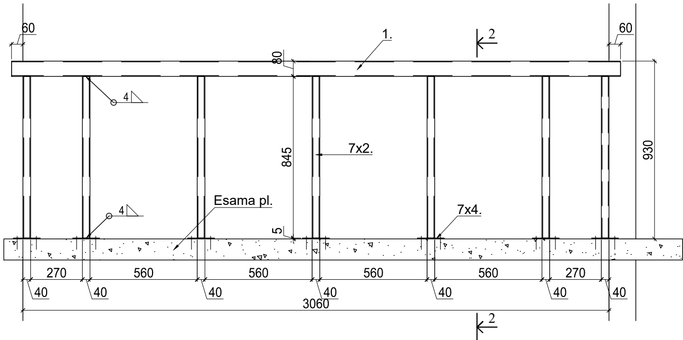
Pjūvis 1-1 M1:20
