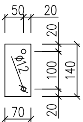
Plokštelė 5. M1:10
