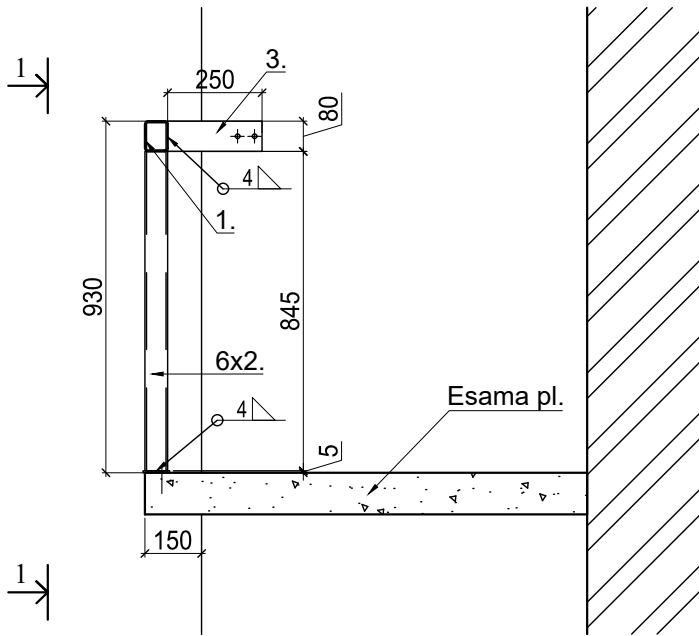
Pjūvis 2-2 M1:20
