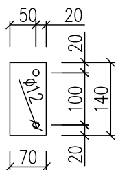
Plokštelė 5. M1:10
