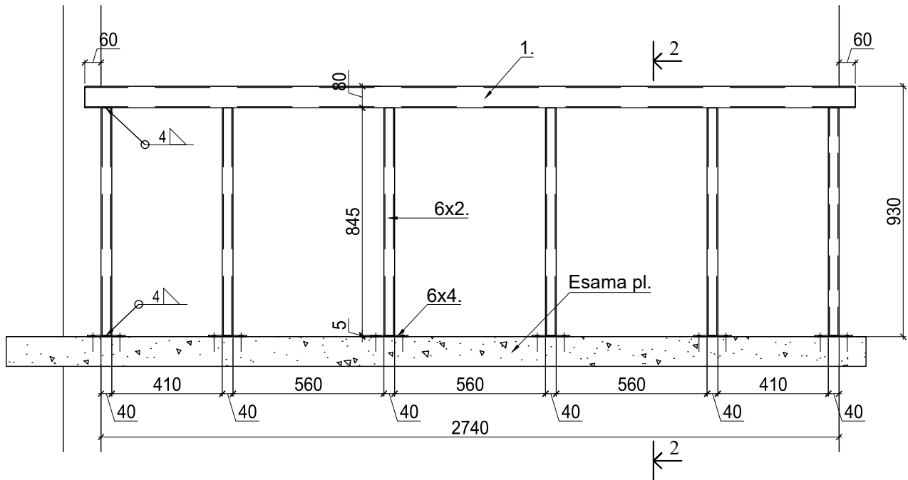
Pjūvis 1-1 M1:20
