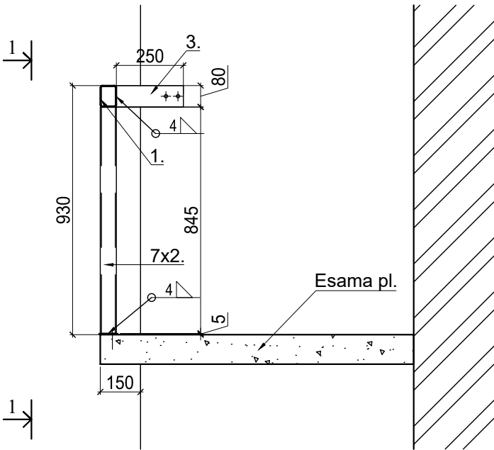
Pjūvis 2-2 M1:20
