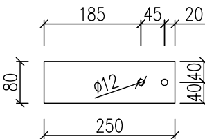
Plokštelė 4. M1:10
