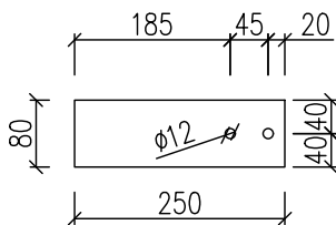
Plokštelė 4. M1:10
