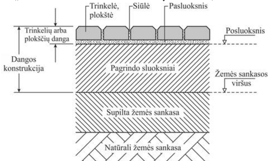
1 pav. Betoninių trinkelės konstrukcijos pavyzdinė struktūra
