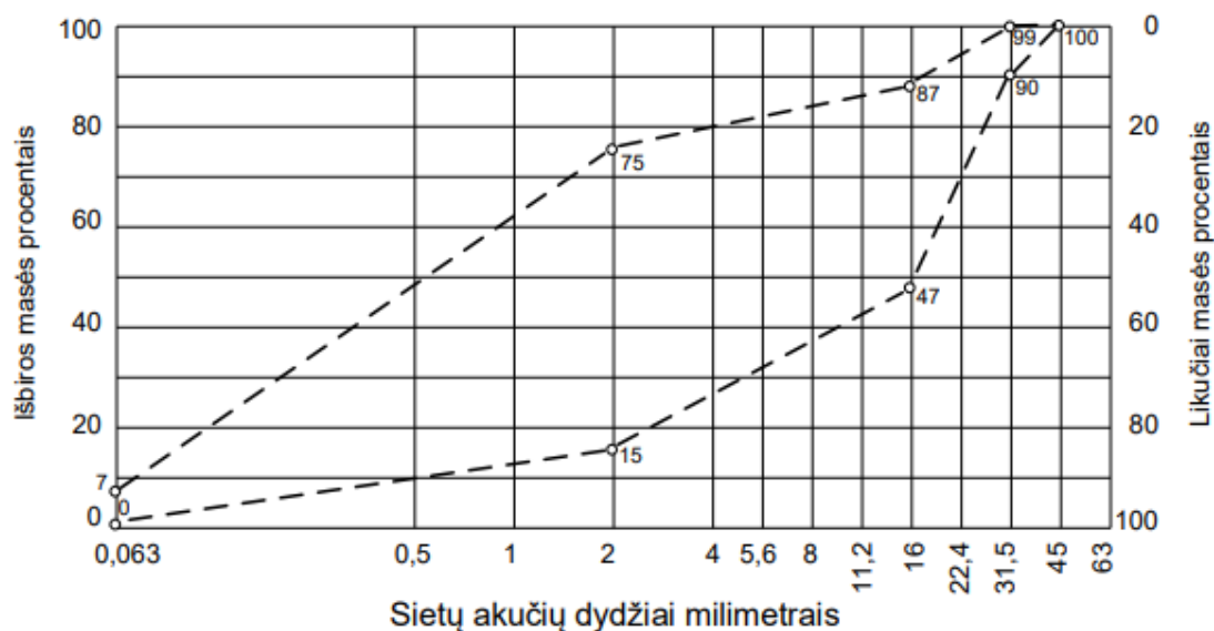
1 pav. Apsauginis šalčiui atsparus sluoksnis iš mišinio 0/32
