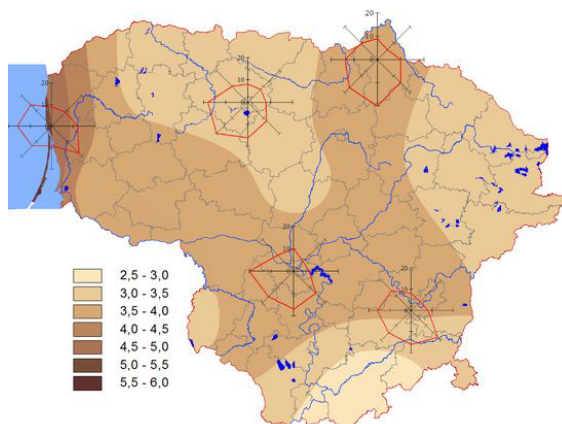
1. pav. Vėjo kryptys
