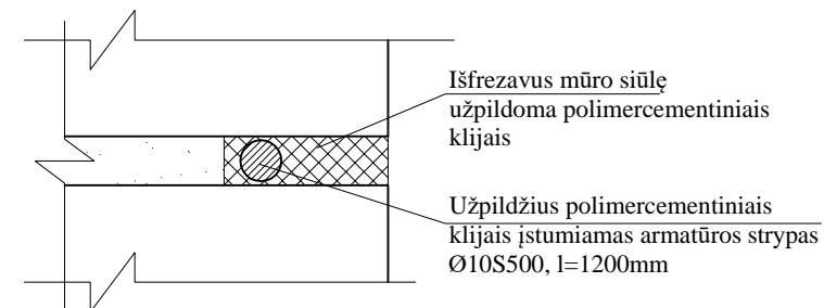
MAZGAS "A" M1:2
