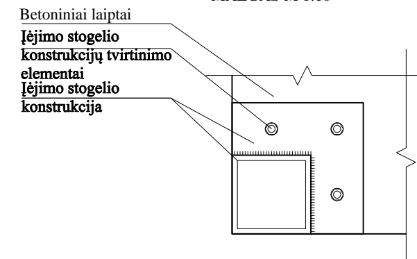
PRINCIPINIS STOGELIO GAMINIO TVIRTINIMO MAZGAS M 1:10
