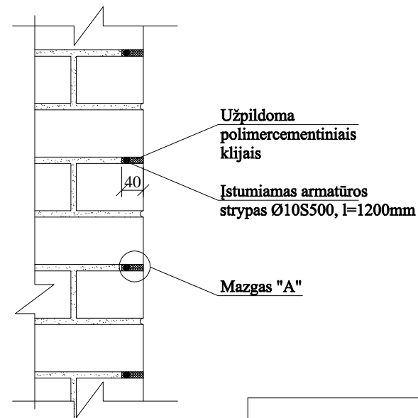
PJŪVIS 1-1 M1:10
