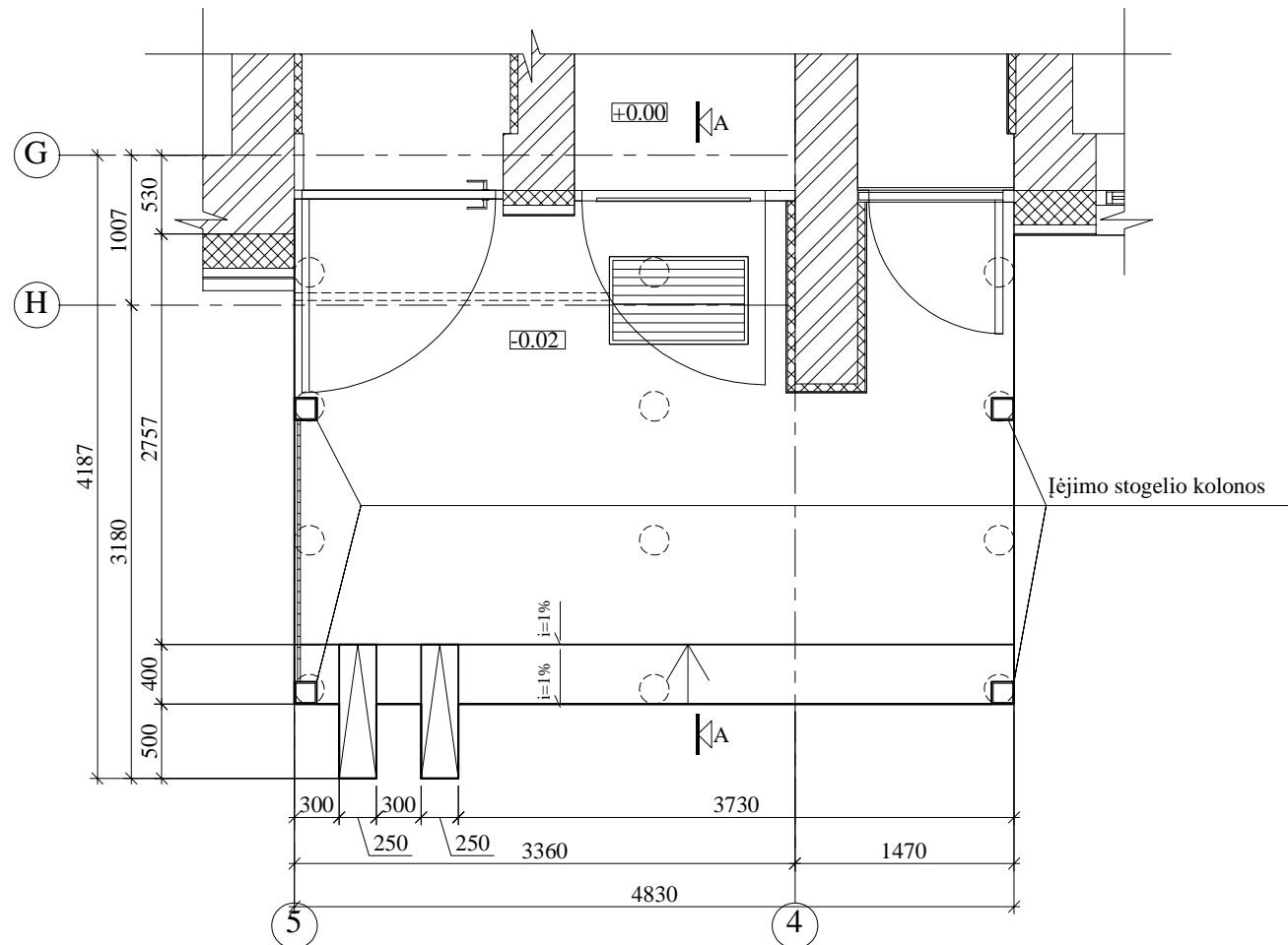
POLIŲ PLANAS M 1:50
