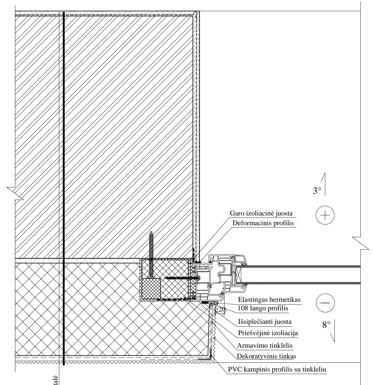
RŪSIO LANGŲ ŠONINIO ANGOKRAŠČIO ĮRENGIMO DETALĖ M 1:5
