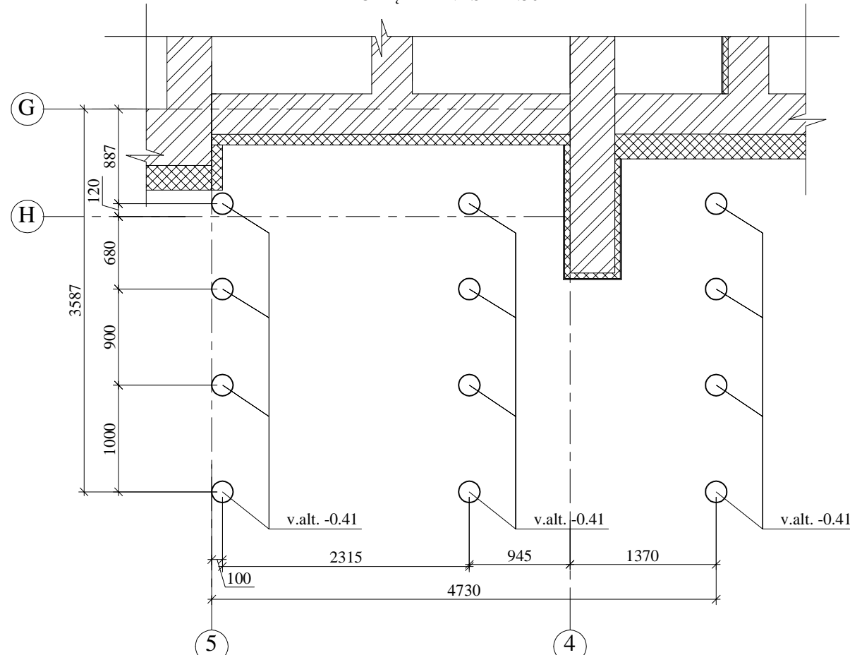
POLIŲ PLANAS M 1:50
