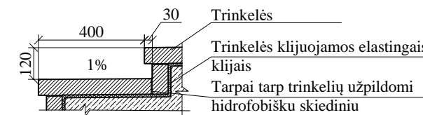
LAIPTŲ APDAILOS ĮRENGIMAS M 1:20
