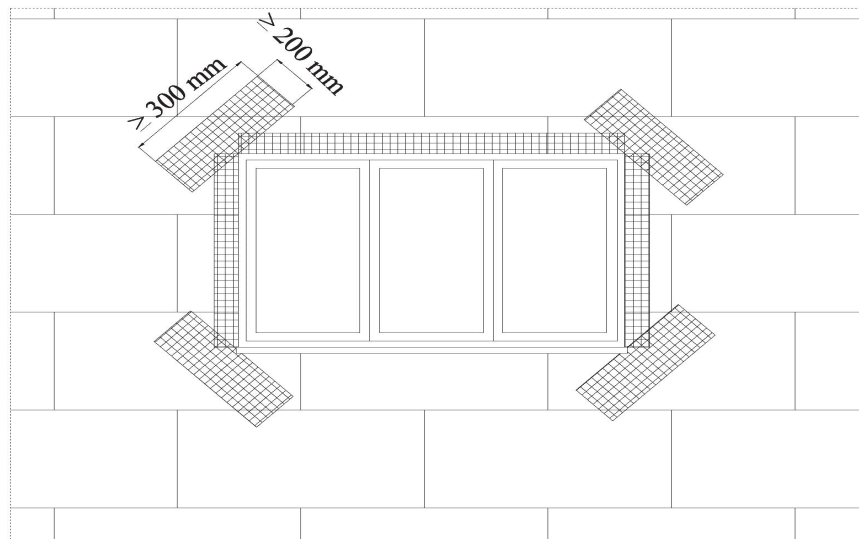
5pav. Papildomų armavimo tinklelių išdėstymas ties angukampais ir briaunomis.
