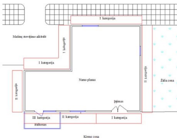
1 paveikslas. Vėdinamos sistemos naudojimo kategorijos parinkimo pastato fasade schema
