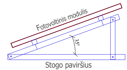
Fotovoltinių modulių laikančioji balastinė konstrukcija
