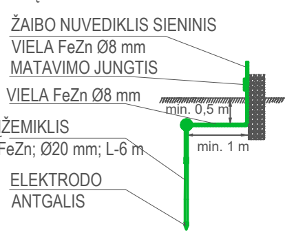
ĮŽEMIKLIO MONTAVIMO ESKIZAS:
