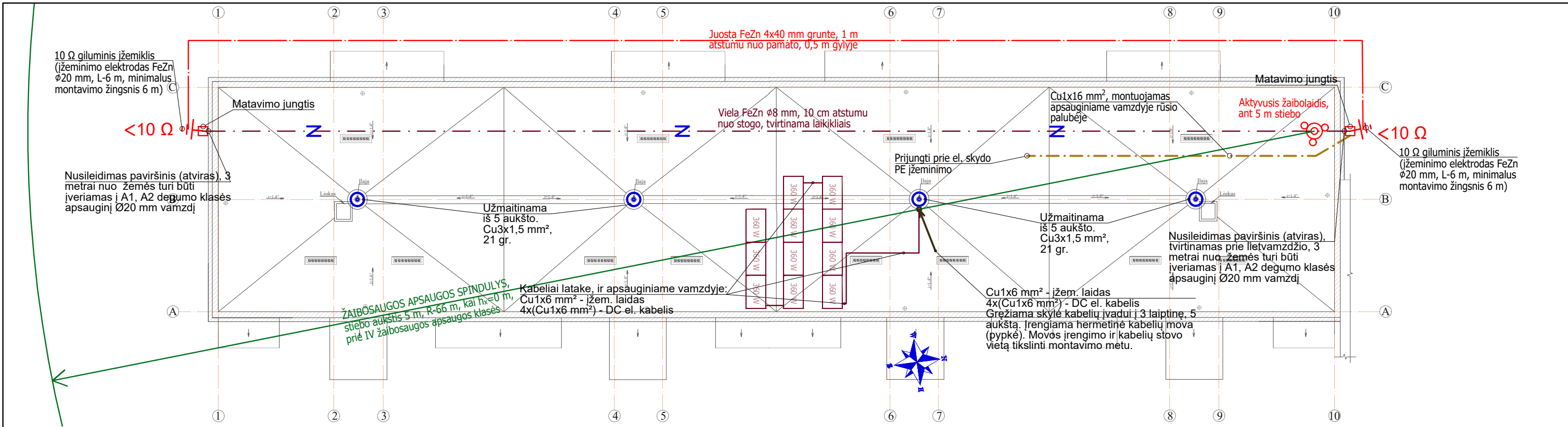
PRINCIPINĖ AKTYVINĖS ŽAIBOSAUGOS ĮRENGINIO SCHEMA
