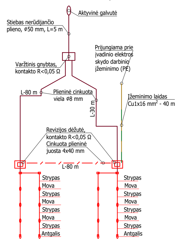
PRINCIPINĖ AKTYVINĖS ŽAIBOSAUGOS ĮRENGINIO SCHEMA
