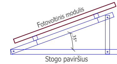
Fotovoltinių modulių laikinčioji balastinė konstrukcija
