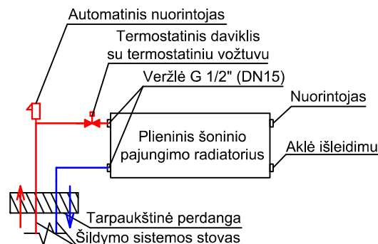
Laiptinės radiatoriaus pajungimo schema
