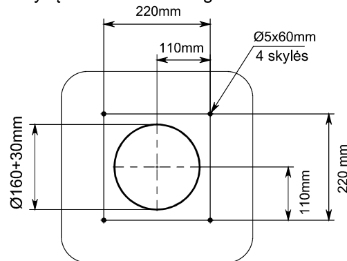
Skylių atstumai išorinio gaubto tvirtinimui
