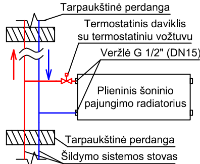
Radiatorių pajungimo schema (tarpinių aukštų)
