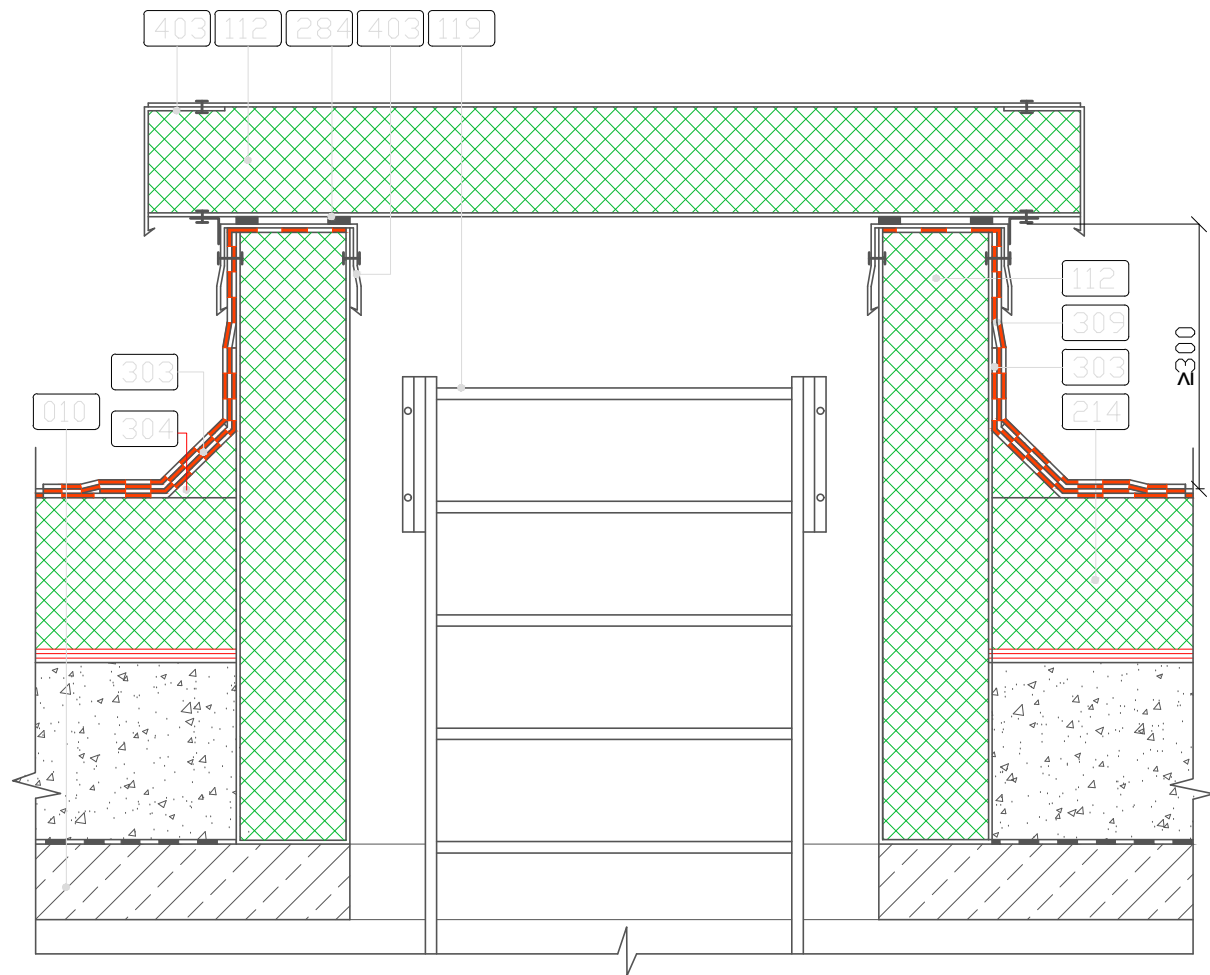
DETALĖ LK - 01
