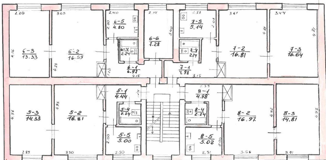
Pav. 4. 2-ojo aukšto kadastrinis planas
