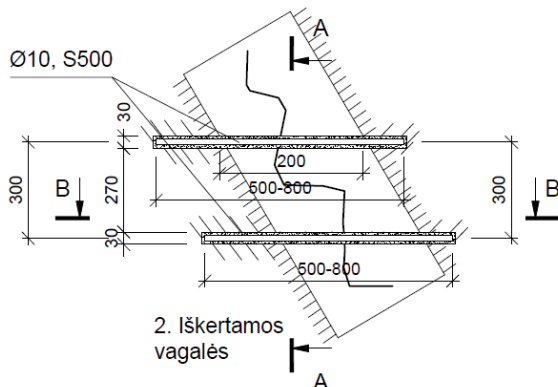
Mūro stiprinimas
