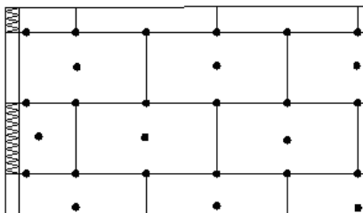
Smeigių išdėstymo schema, 1 m^2 tvirtinant 6 smeiges 6 smeiges kampuose
