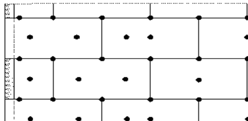
Smeigių išdėstymo schema, 1 m^2 tvirtinant 5-
