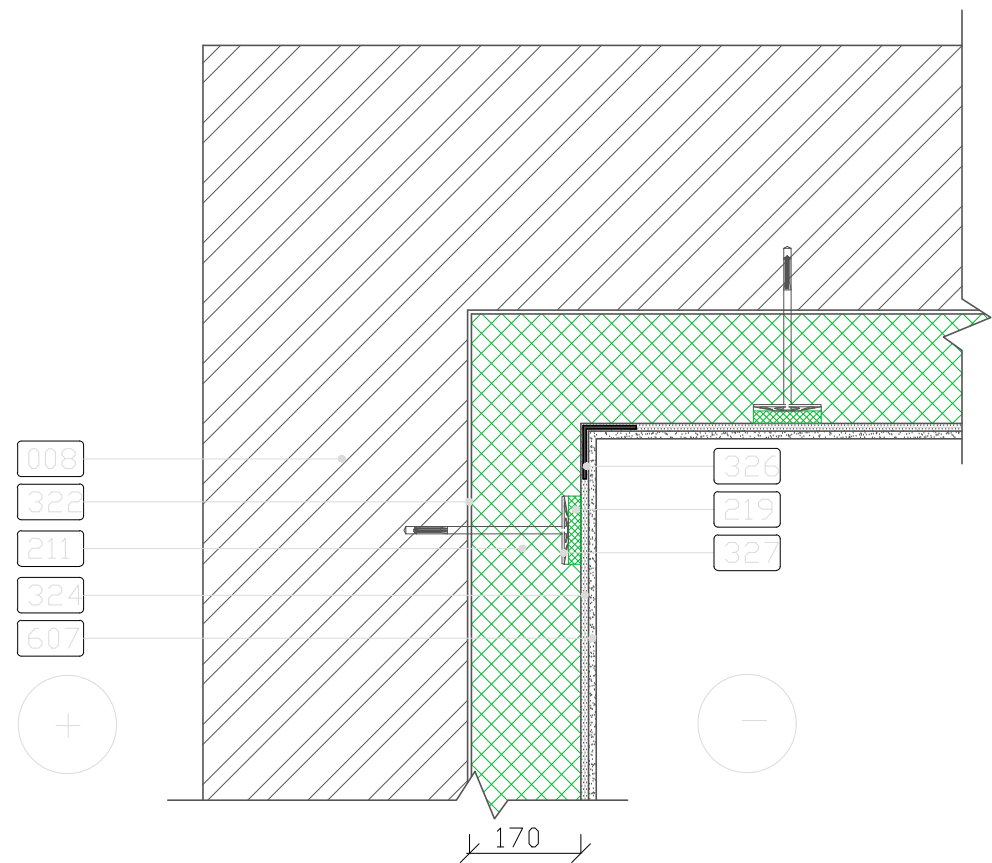
DETAL Ė SN - 02 ties vidin iu kampu
