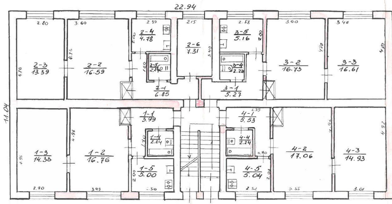
Pav. 3. 1-ojo aukšto kadastrinis planas
