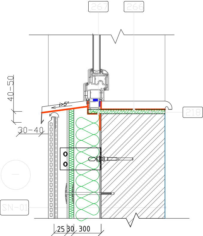
DETALĖ ANG - 01 vertikalus pjūvis
