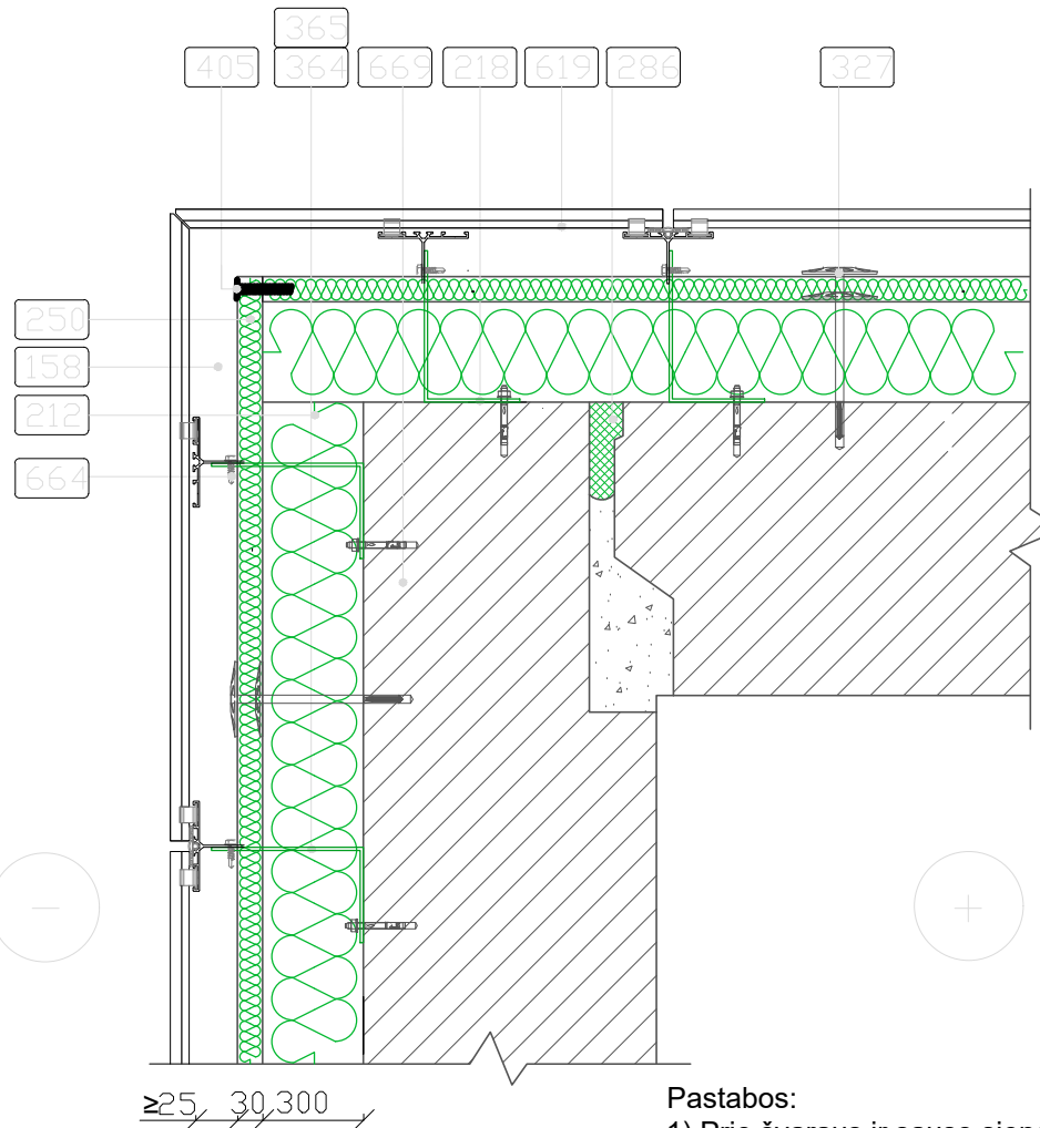
DETALĖ SN - 01
