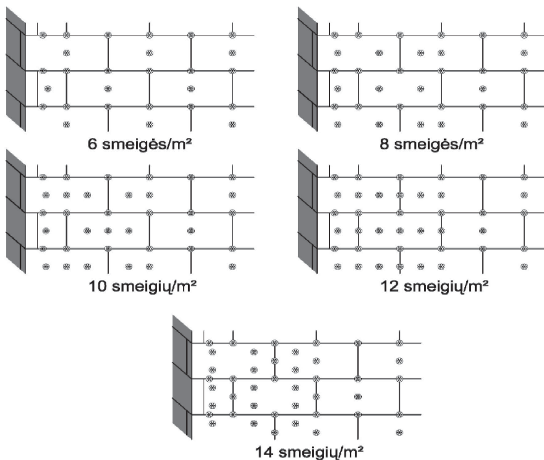
4 pav. Smeigių išdėstymo schema, kai šiltinimo plokštė tvirtinama prie pastato kampo.
