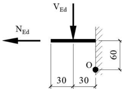
Istiklinimo tvirtinimo skaičiuojamoji schema Nr.2.
