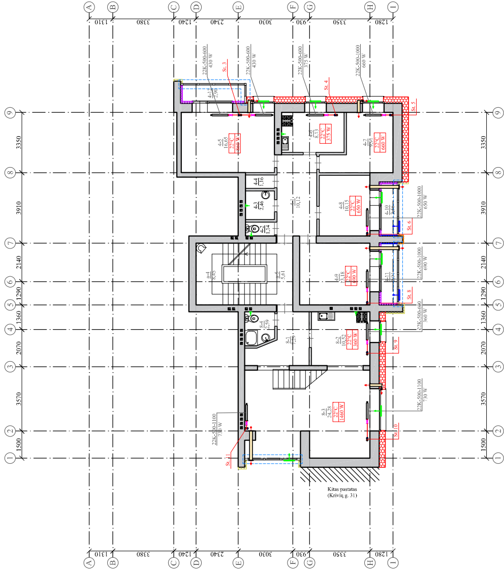
Pirmo aukšto planas M 1:150
