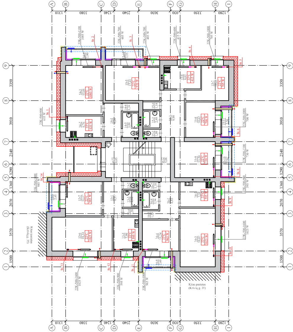
Ketvirtio aukšto planas M 1:150
