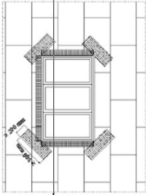
ANGOKRAŠČIŲ KAMPŲ ARMAVIMAS
