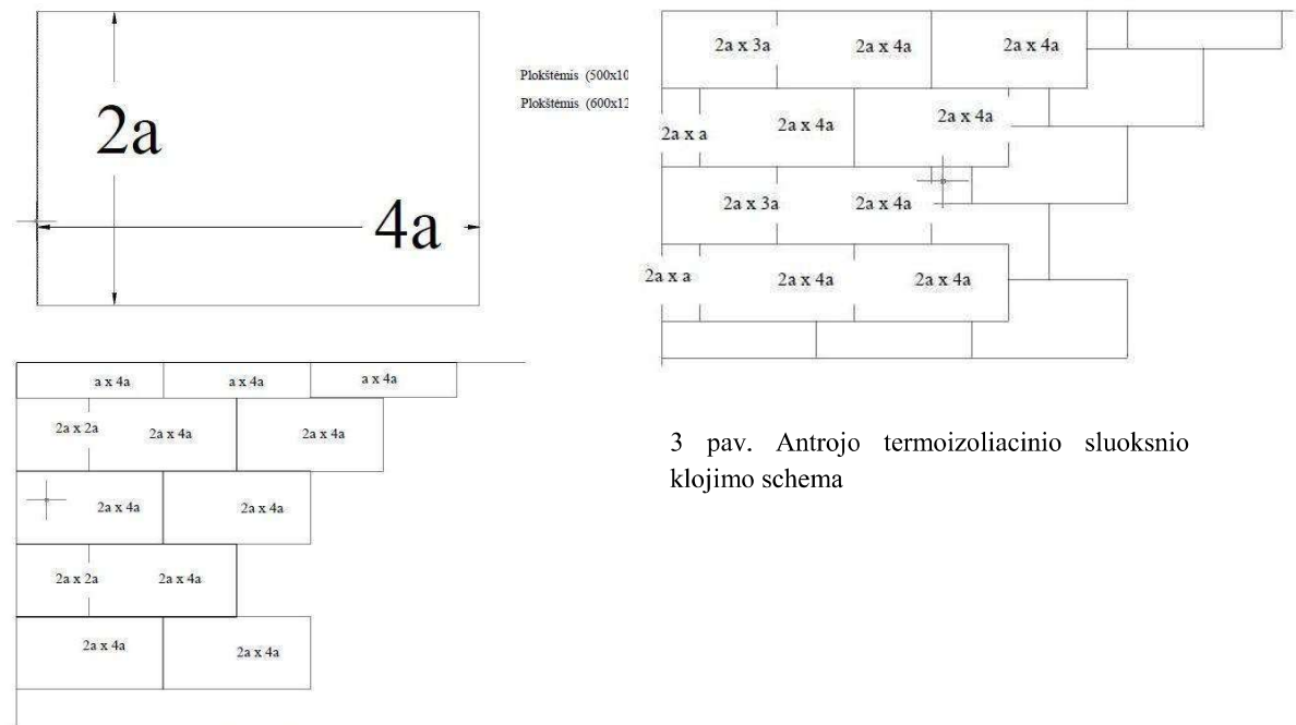
2 pav. Pirmojo termoizoliacinio sluoksnio klojimo schema
