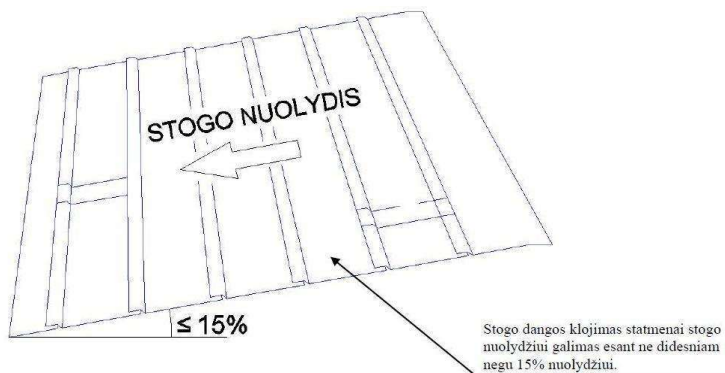
6 pav. Dengimas danga ant šlaito
