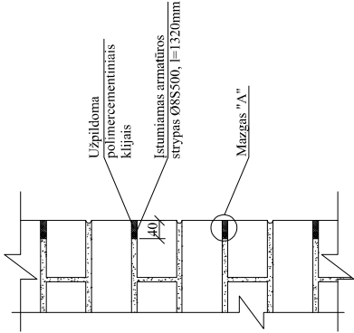
PIŪVIS I-I M1:10
