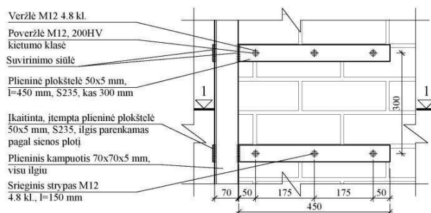
SIENOS KRAŠTO SUSTIPRINIMO DETALĖ M1:10
