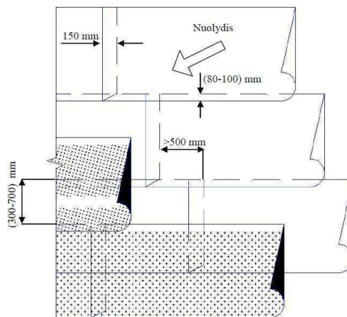
8 pav. Poslinkis sutampančiuose stogo dangų sluoksniuose
