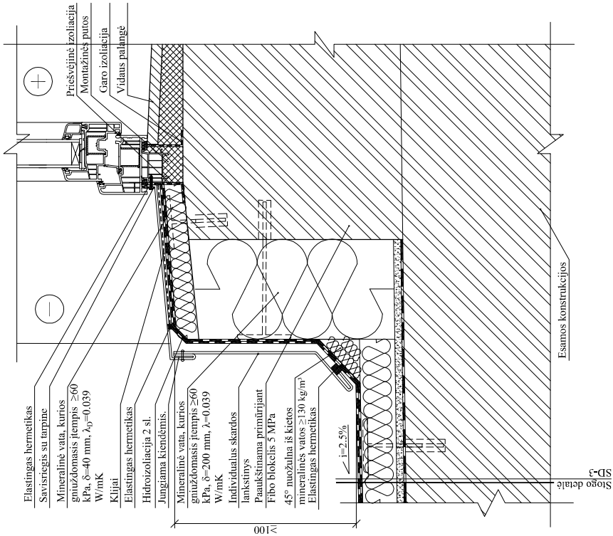
STOGELIO SU LAIPTINĖS LANGO ANGOKRAŠČIU SUJUNGIMO DETALĖ M 1:5
