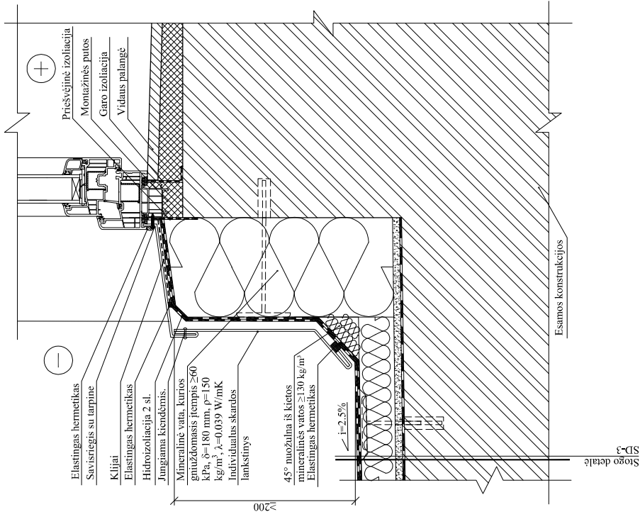
STOGELIO SU LAIPTINĖS LANGO ANGOKRAŠČIU SUJUNGIMO DETALĖ M 1:5
