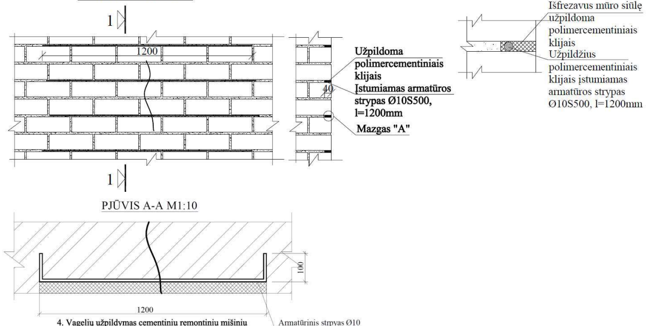
SIENOS TVIRTINIMO ARMATŪRINIAIS STRYPAIS SCHEMA, KAI TVIRTINAMAS VIENAS PLYŠYS M1:10
