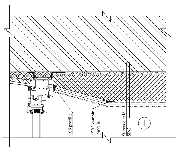
BALKONŲ VIDAUS STIKLINIMŲ ANGOKRŠČIŲ APŠILTINIMO DETALĖ M 1:5
