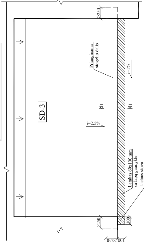
IĖJIMO STOGELIO PLANAS M 1:20
