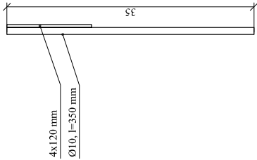
METALO JUOSTA POZ.1 M1:5
