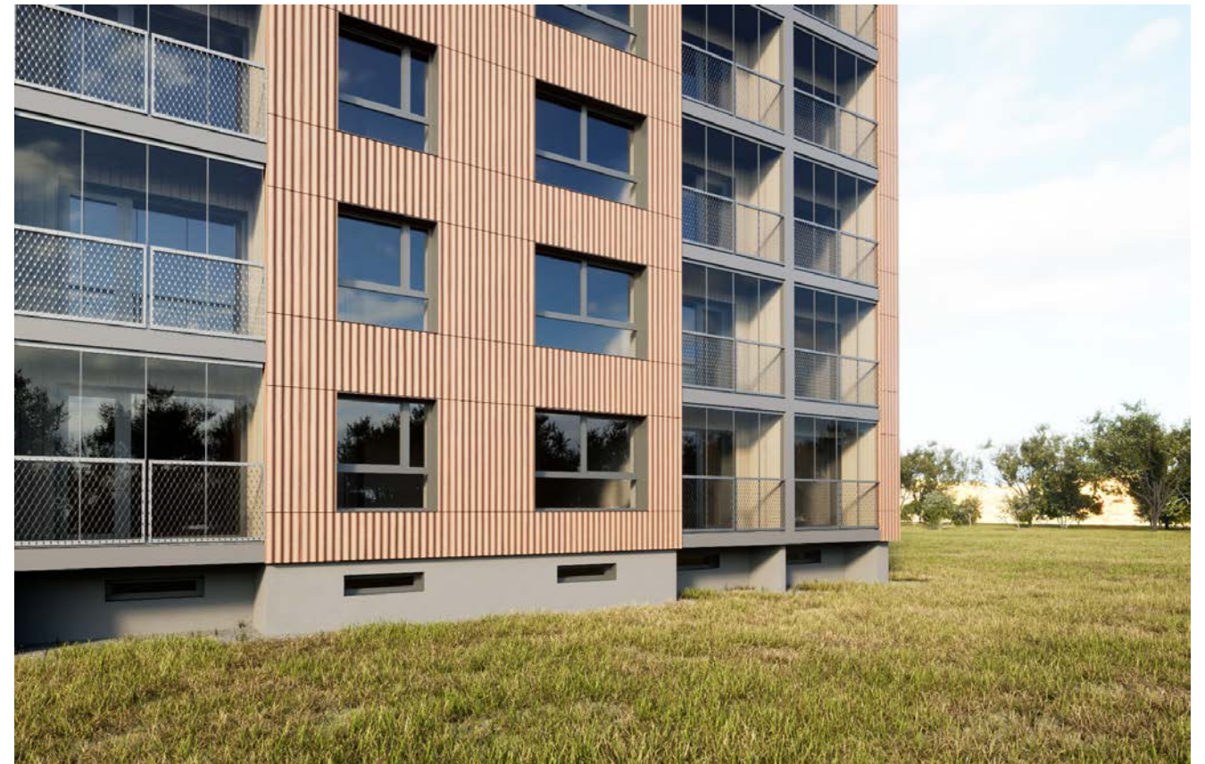
Vizualizacija: lodžių stiklinimas „šalta“ berėmė sistema
