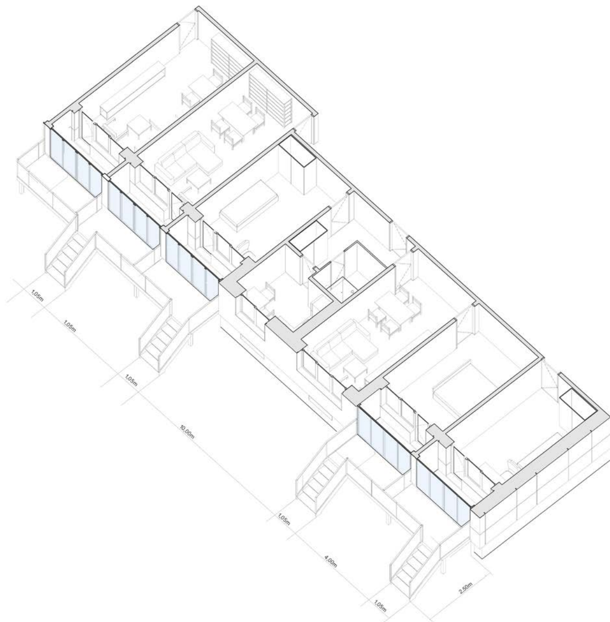
Variantas 2: terasa ir laipteliai
