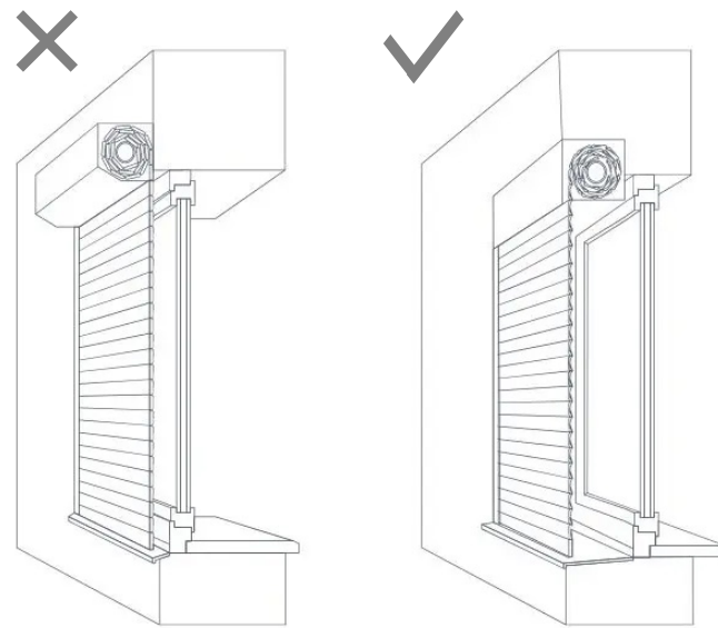
Apsauginių žaliuzių montavimo angokraštyje pavyzdys
