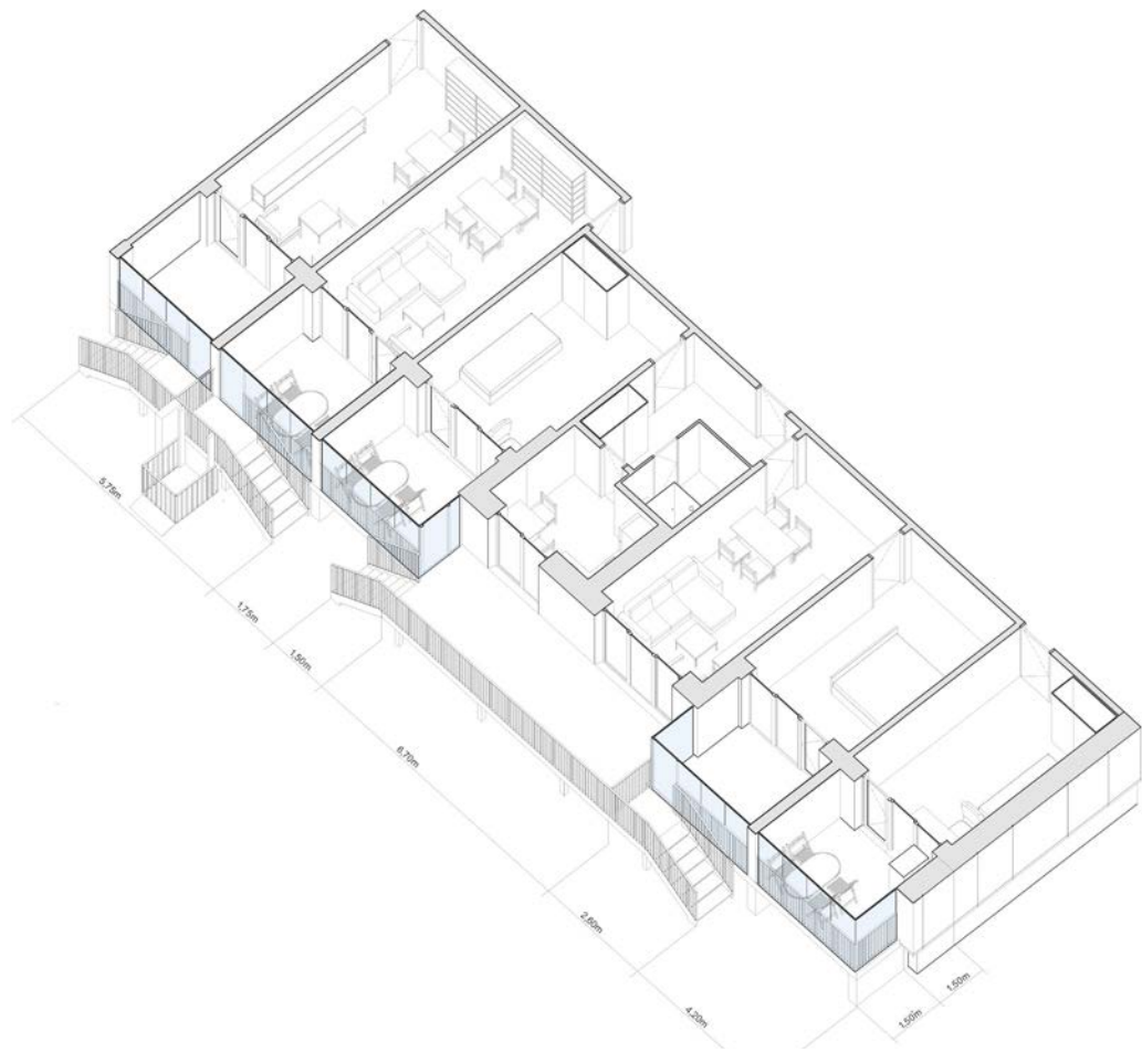
Terasų ir keltuvų išdėstymo schema pirmame aukšte
