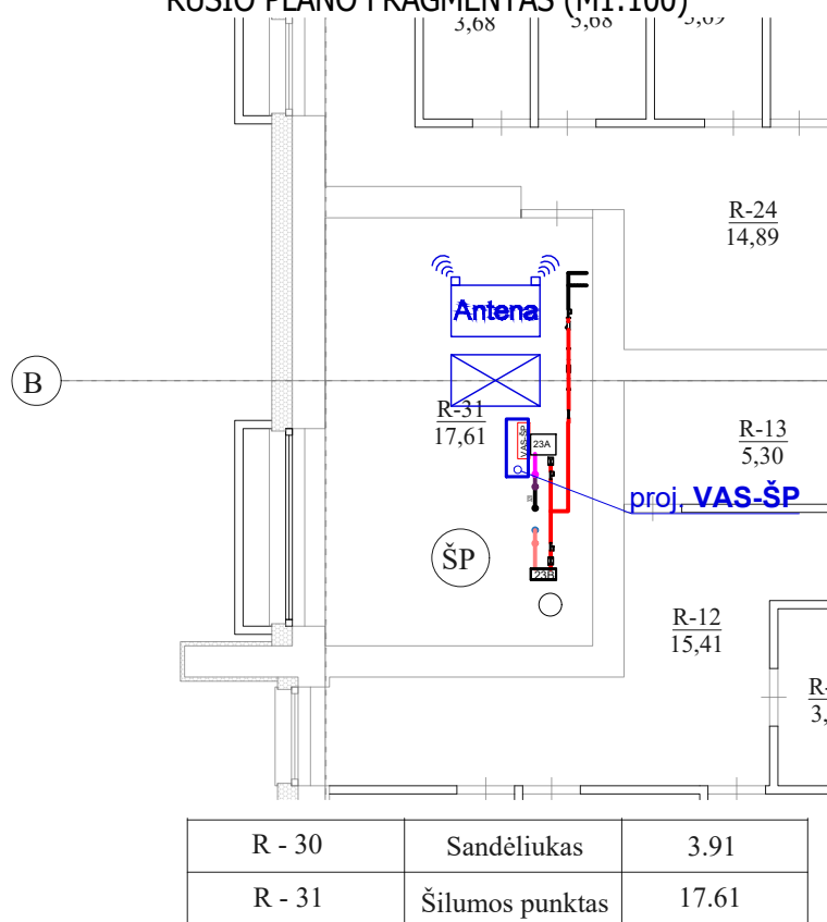
RŪSIO PLANO FRAGMENTAS (M1:100)
