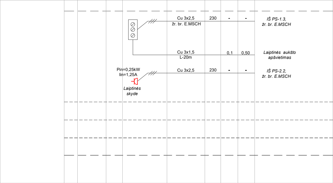
Skyde montuojama papildoma bendrųjų reikiųjų el. tinklo paskirstymo įranga:
