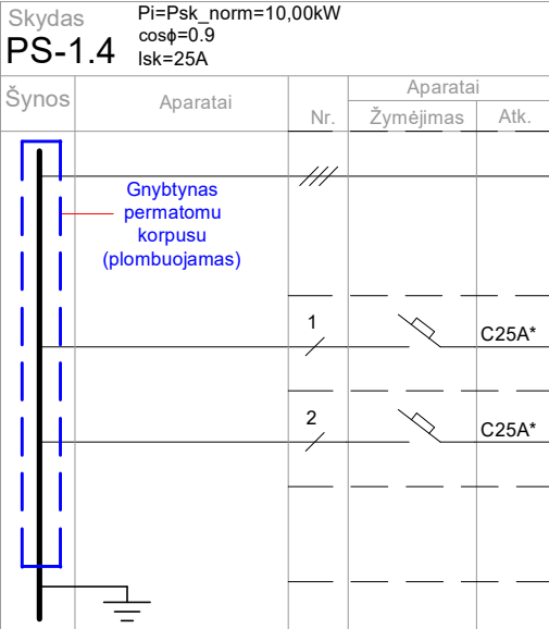
Skyde montuojama papildoma bendrųjų reikiųjų el. tinklo paskirstymo įranga:
