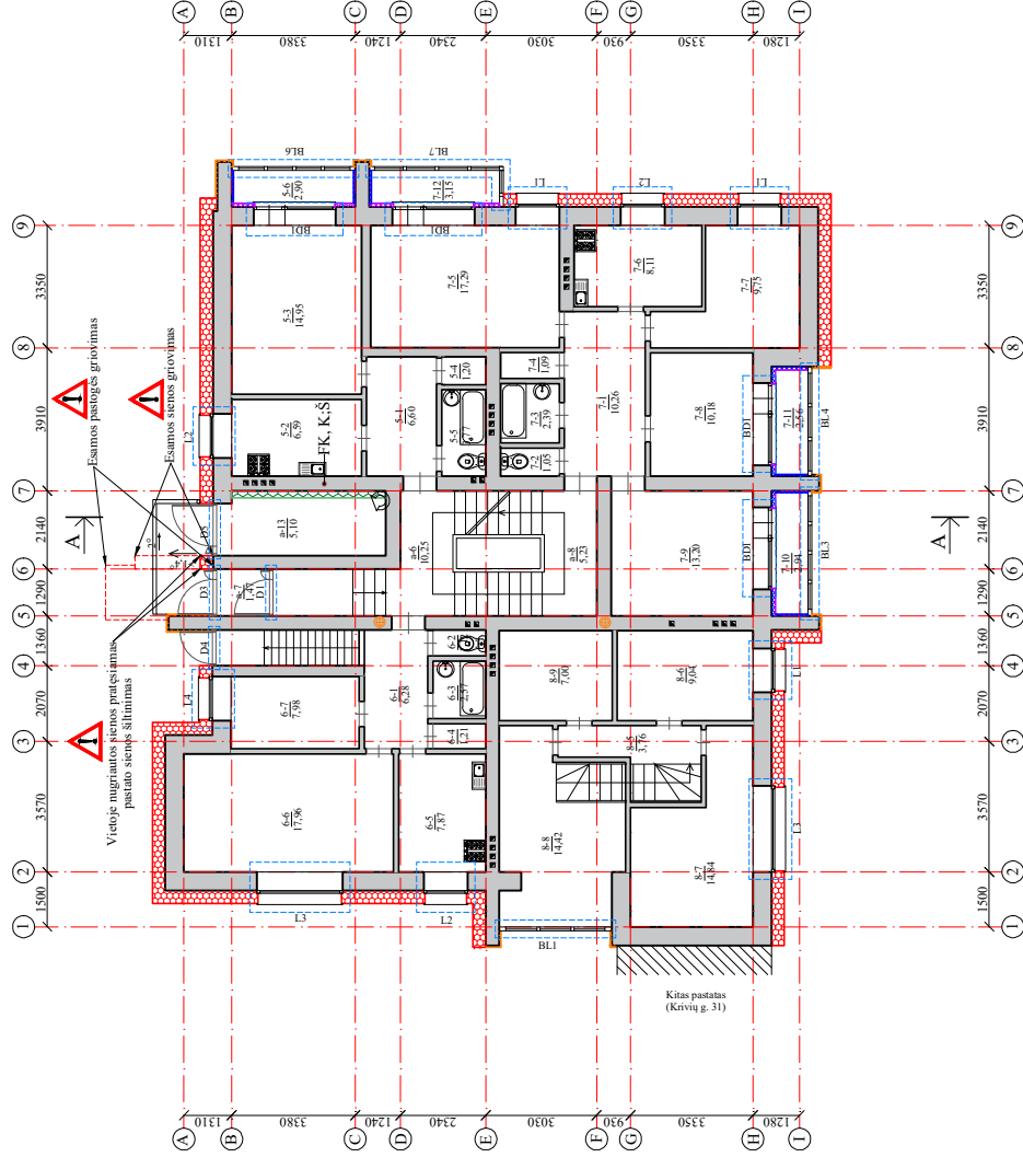
Antro aukšto planas M 1:100
