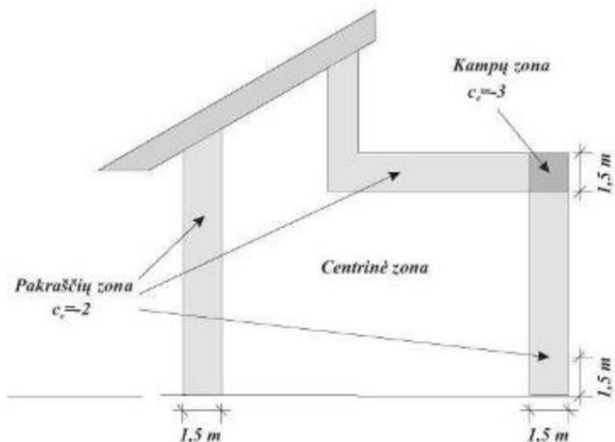
1 pav. Pastato aerodinaminių koeficientų nustatymo schema.
