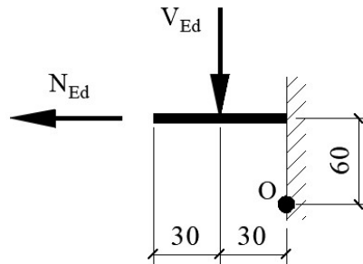
Įstiklinimo tvirtinimo skaičiuojamoji schema Nr.2.
