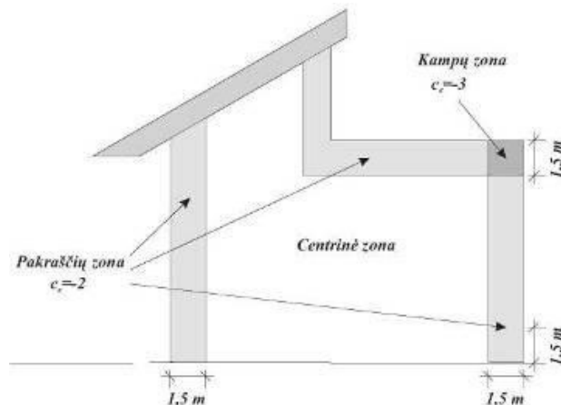
1 pav. Pastato aerodinaminio koeficientų nustatymo schema.
