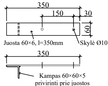
Detalė A1 plienas S275
