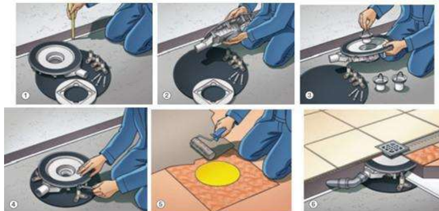
10 pav. Trapo montavimo pavyzdžiai
