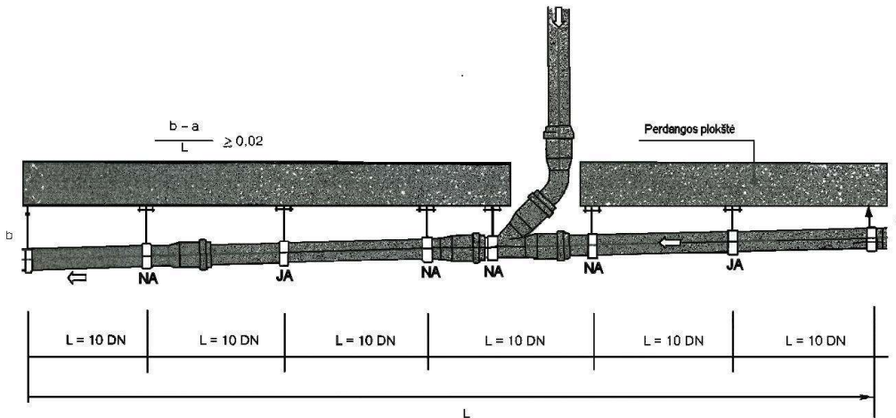
5 pav. Pakabinto vamzdyno tvirtinimas
