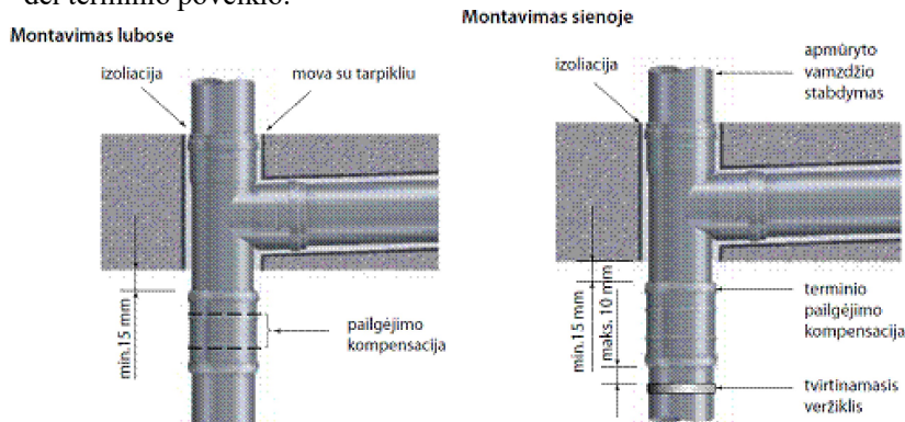
8 pav. Dalinis kanalizacijos vamzdžių apmūrijimas
