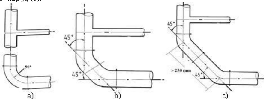
1 pav. Stovų jungimas prie išvadų
