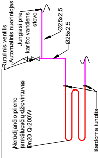
RANKŠUOSIŲ DŽIOVINTUVŲ PALUNGIMO PRINCIPINE SCHEMA
