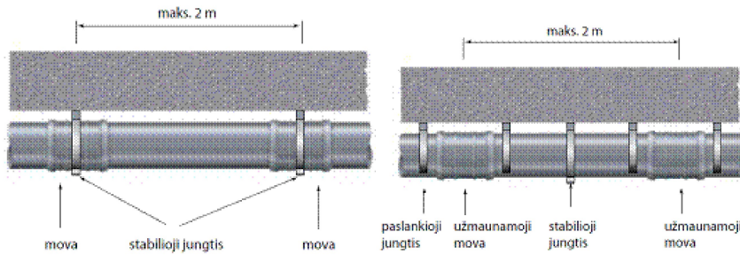
9 pav. Vamzdyno montavimas naudojant movas
