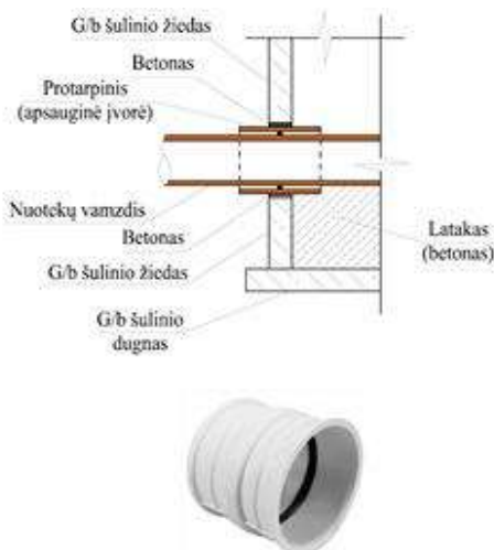
11 pav. Vamzdžio pajungimas G/B šuliniuose
