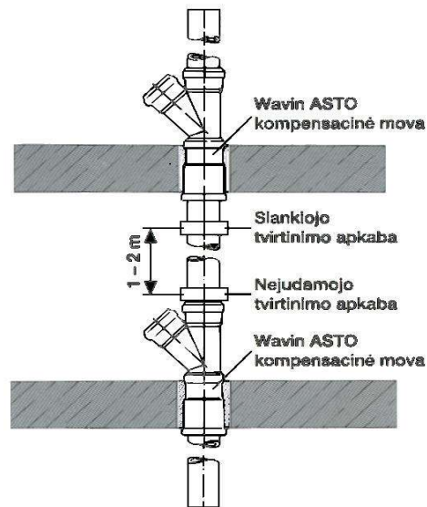
4 pav. Vertikalaus stovo tvirtinimas
