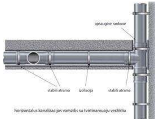
7 pav. Iš dalies įmūrijamo vamzdyno montavimas
