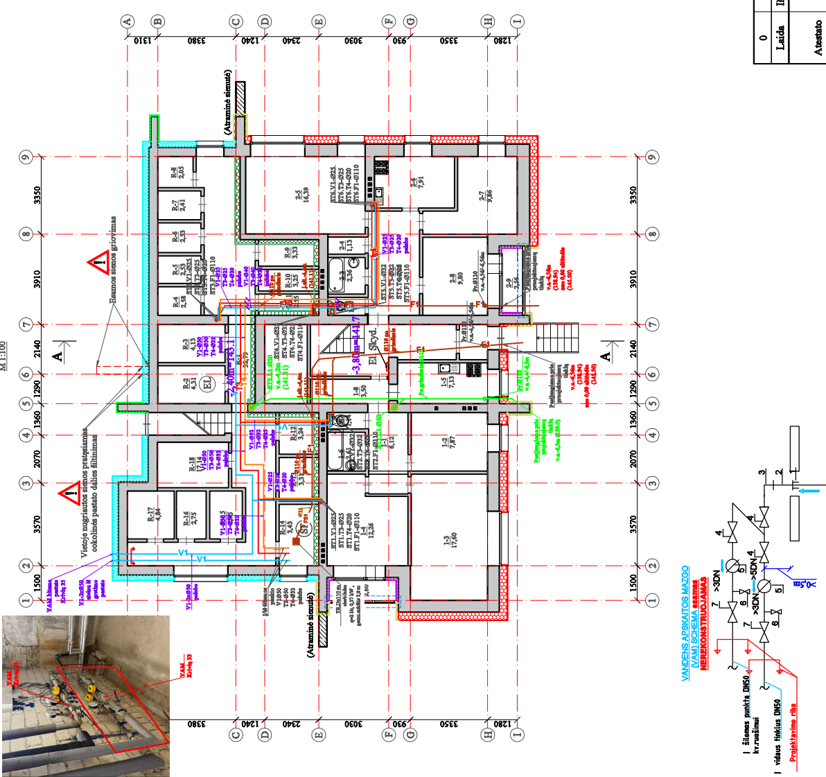
Rūsiu ir cokolinio ankšto planas M 1:100
