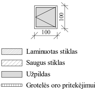
KEIČIAMO LIUKO SCHEMA:
