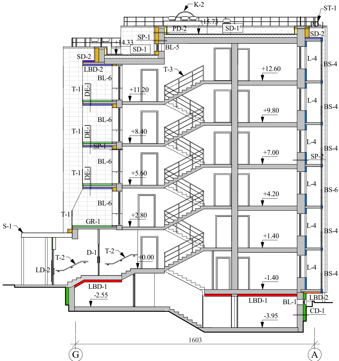
PJŪVIS A-A M 1:150
