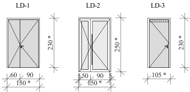
KEIČIAMŲ LAUKO DURŲ SCHEMAS:
