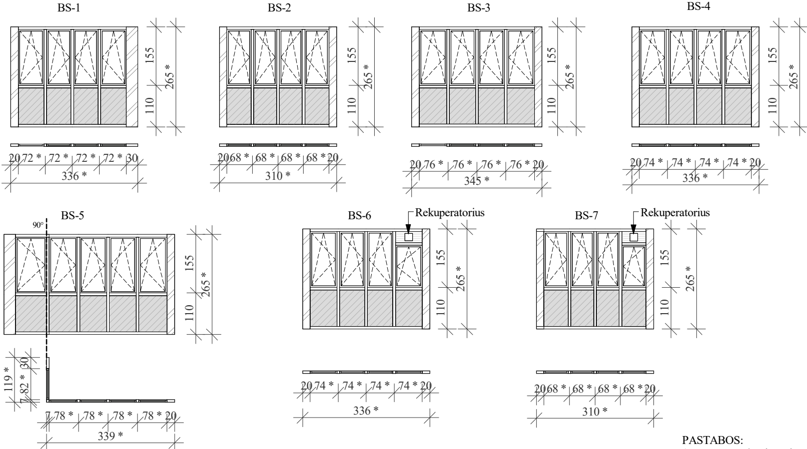
LODŽŲ STIKLINIMŲ SCHEMOS:
