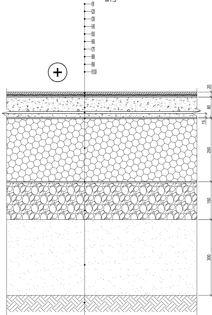
Grindų GR-1.4 detalė M1:5
