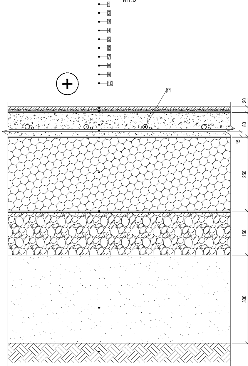
Grindų GR-1.2 detalė M1:5
