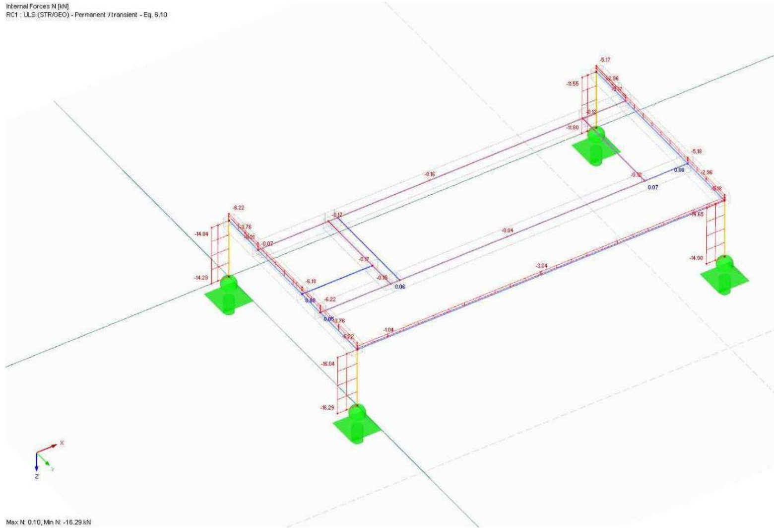
4.14 pav. Konstrukcijų ašinės jėgos N (ULS)
