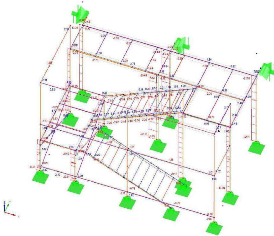
4.34 pav. Konstrukcijos ašinės jėgos N (ULS)
