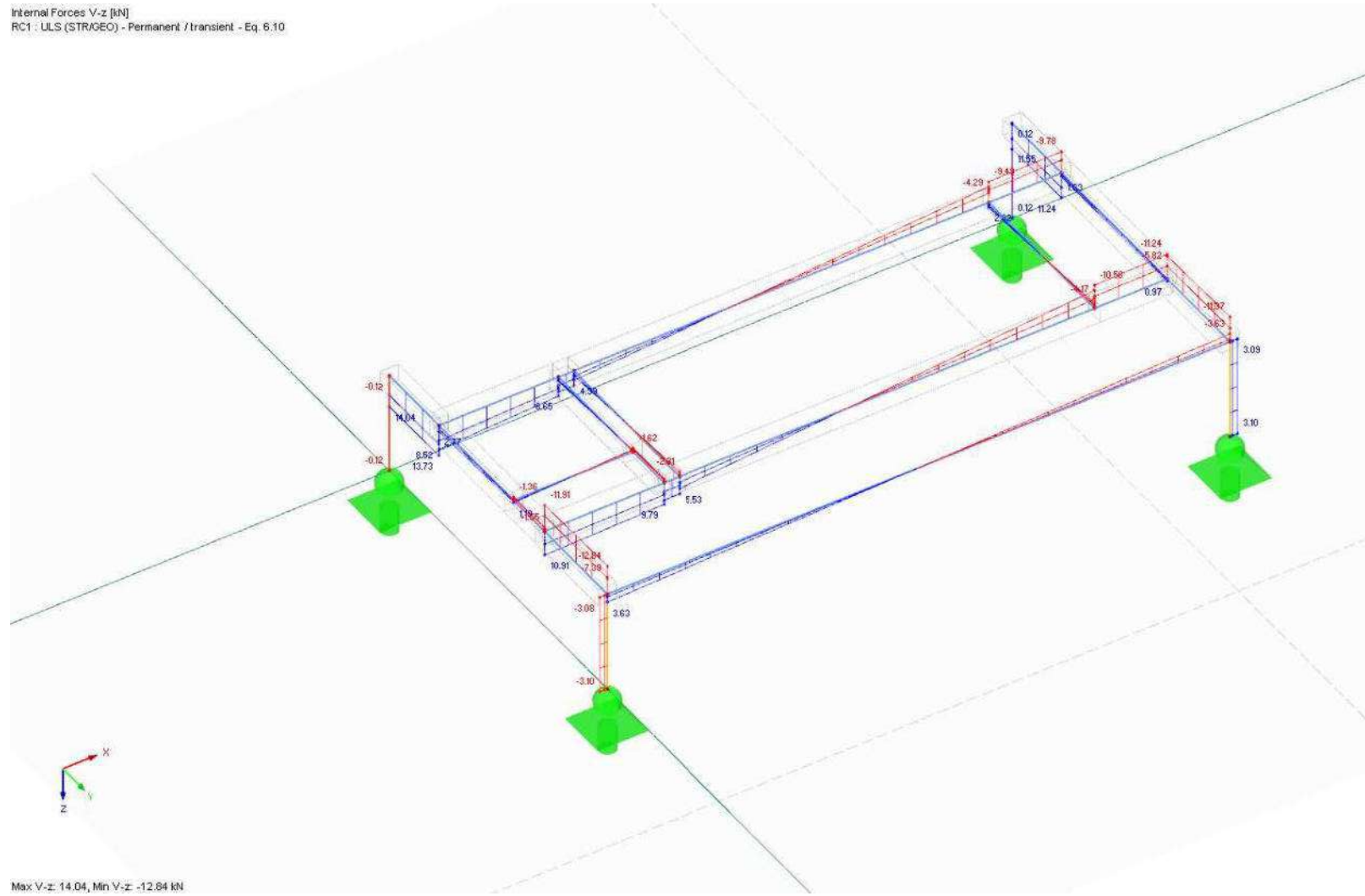
4.12 pav. Konstrukcijų skersinės jėgos Vz (ULS)
