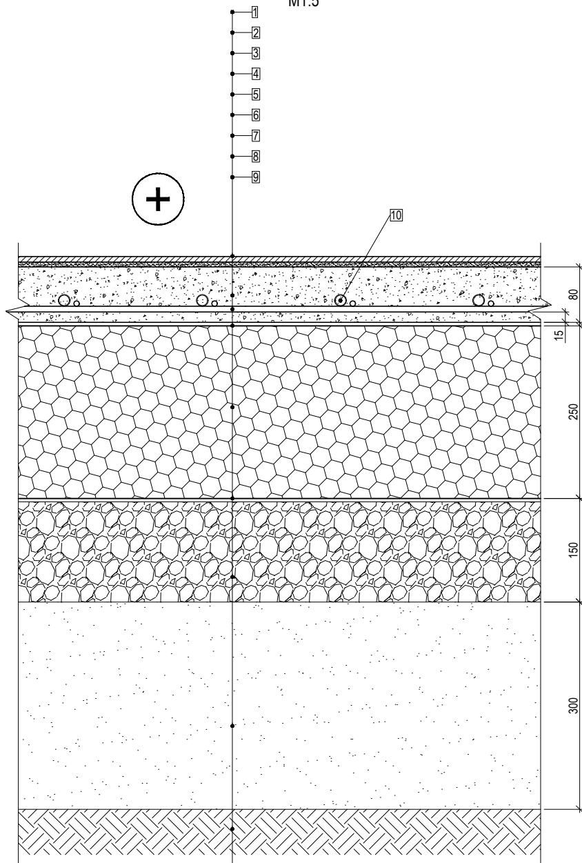
Grindų GR-1.1 detalė M1:5
