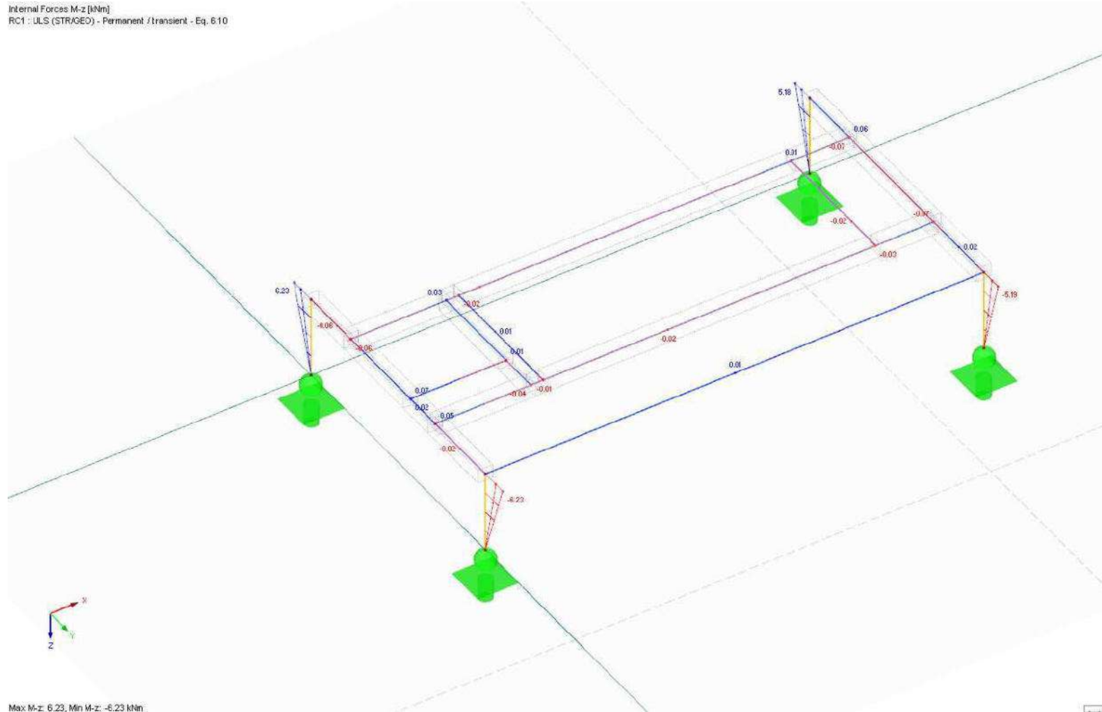
4.11 pav. Konstrukcijų lenkimo momentai Mz (ULS)
