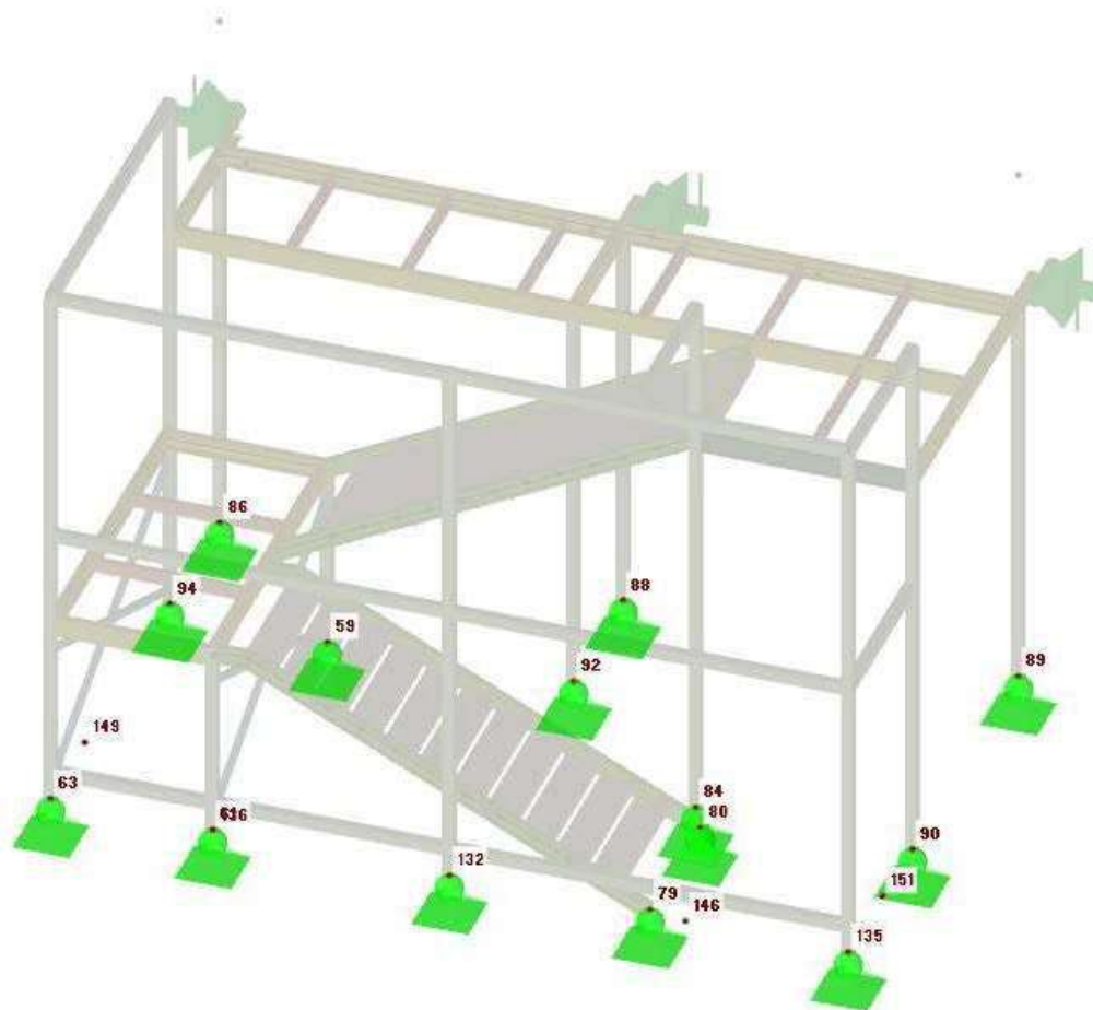
4.35 pav. Atraminių taškų schema
