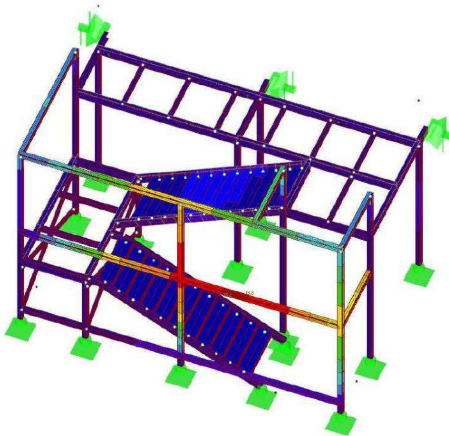
4.29 pav. Konstrukcijos įlinkiai (SLS)
