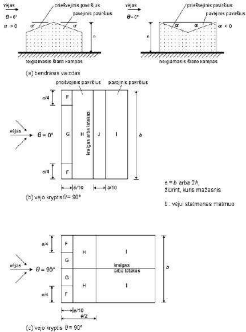
3.7 pav. Vėjo krypties veikimo ir stogo paviršių pasiskirstymo schema
