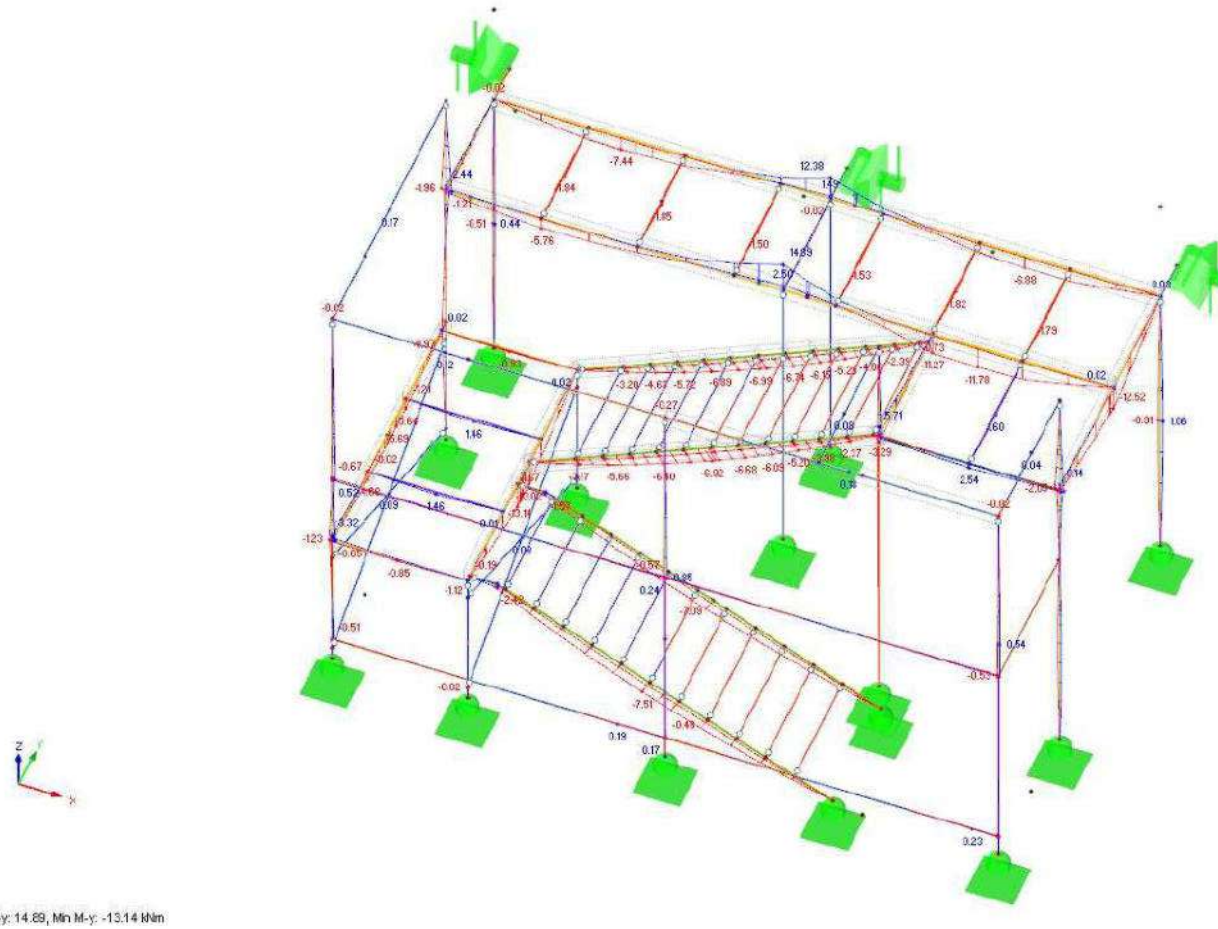
4.31 pav. Konstrukcijos lenkimo momentai My (ULS)
