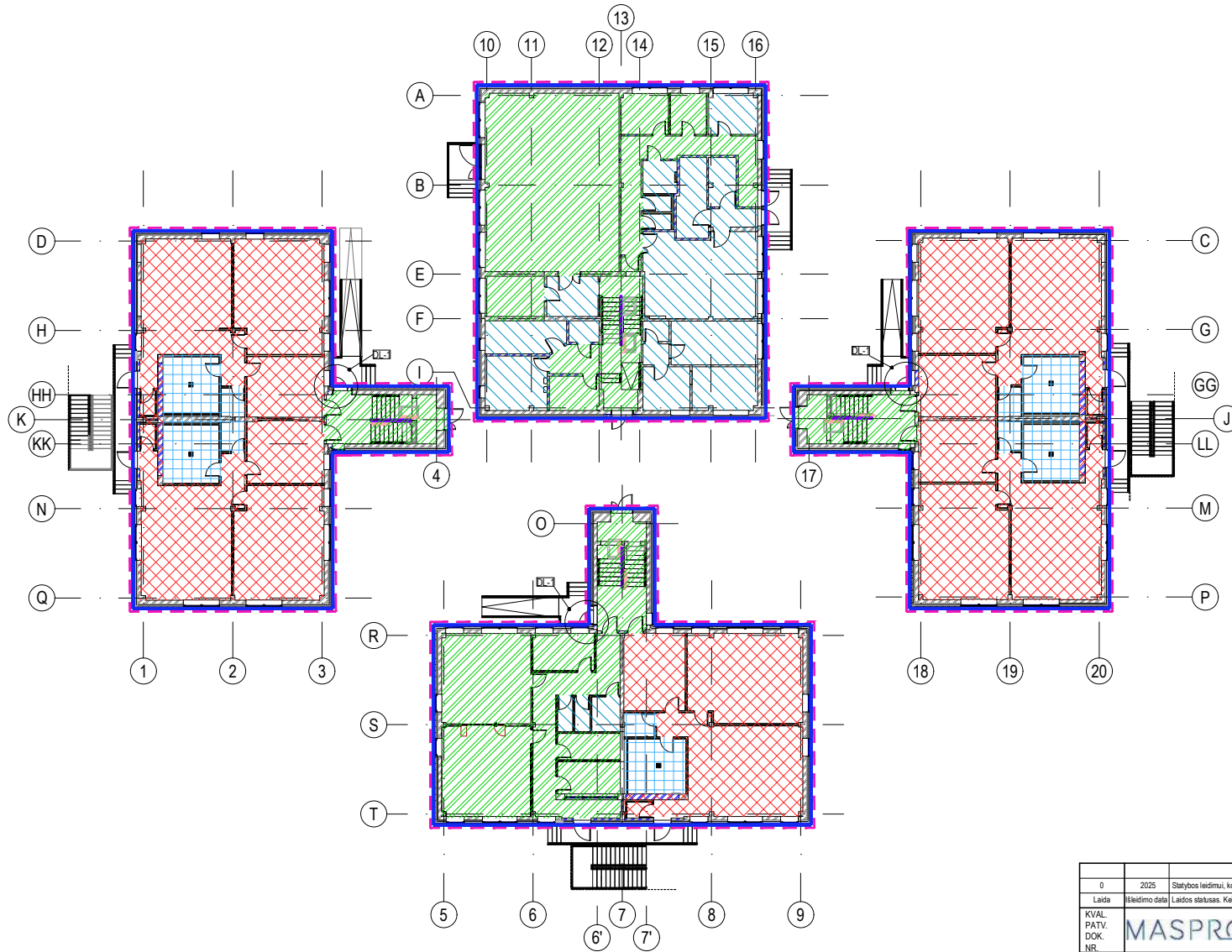
Pirmo aukšto planas su mazgų ir detalių nužymėjimu M1:200
