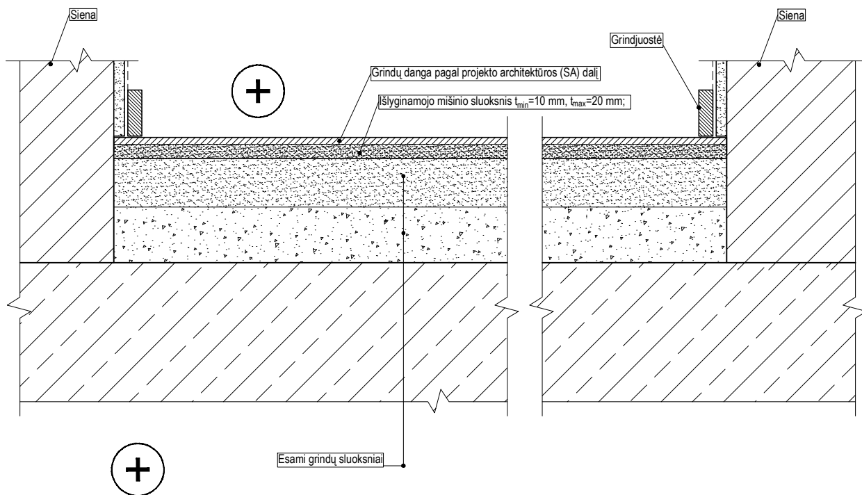
Grindų GR-2.1 detalė M1:5
