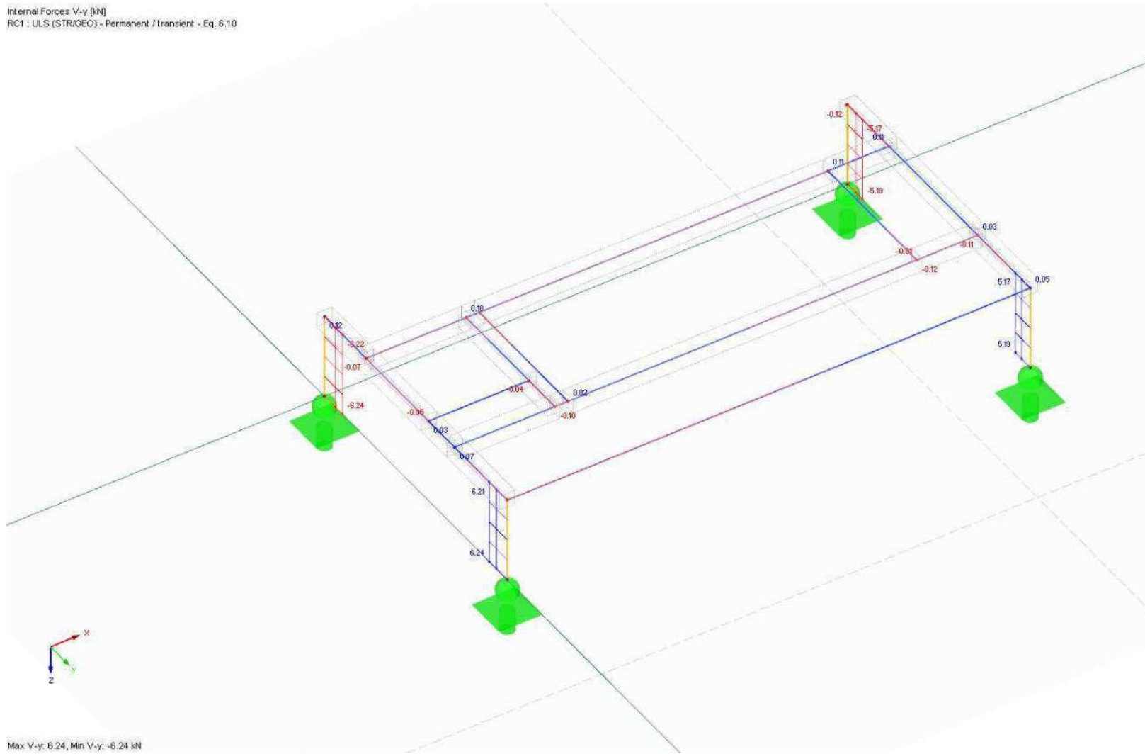
4.13 pav. Konstrukcijų skersinės jėgos V_y (ULS)
