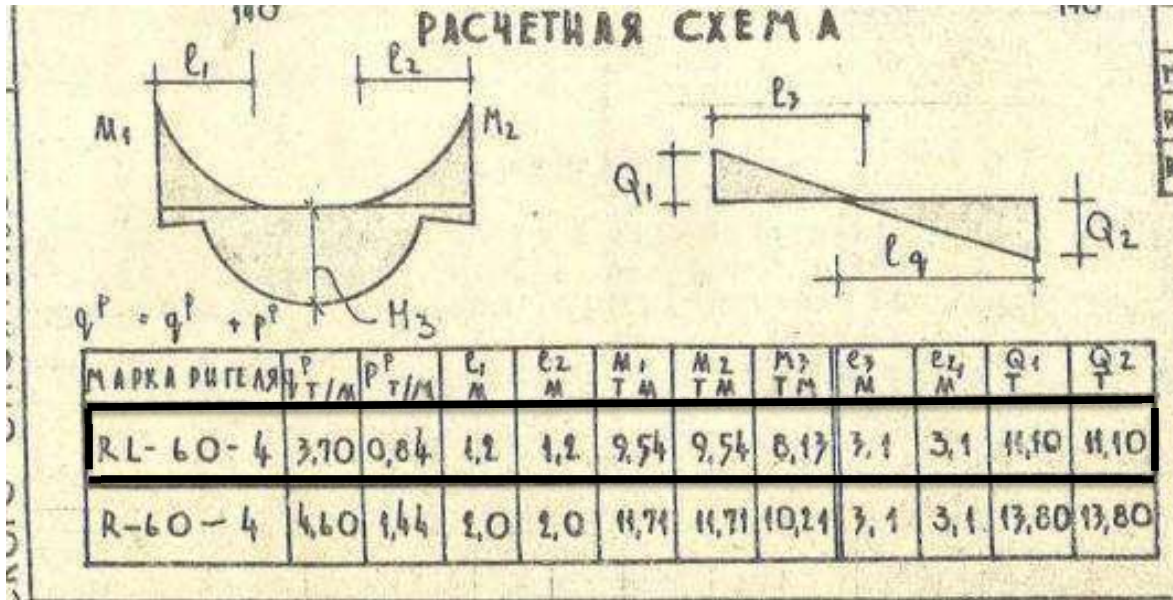
Rygių (rėmsijų) RL-60-4 skaičiuojamoji schema ir skaičiuotinė laikomoji galia pagal [3.1.9] katalogą
