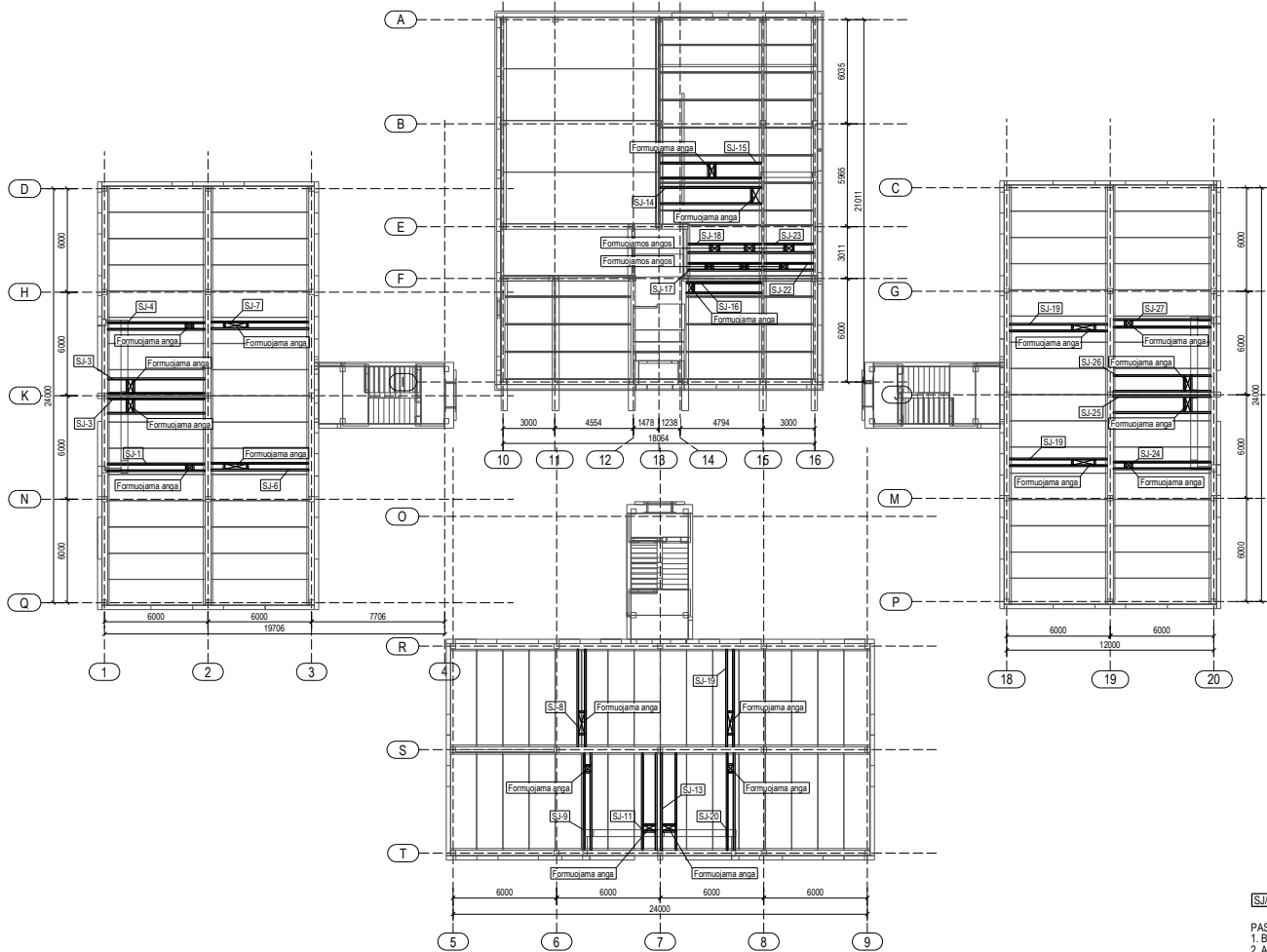
Perdangos planas 1a. 1:200
