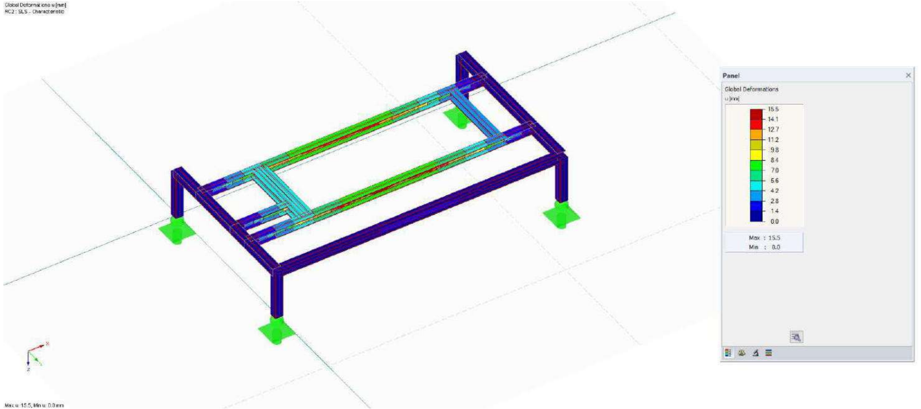
4.9 pav. Konstrukcijų įlinkiai (SLS)
