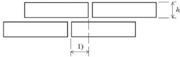
3.1 Paveikslas. Mūro gaminių užlaidos
