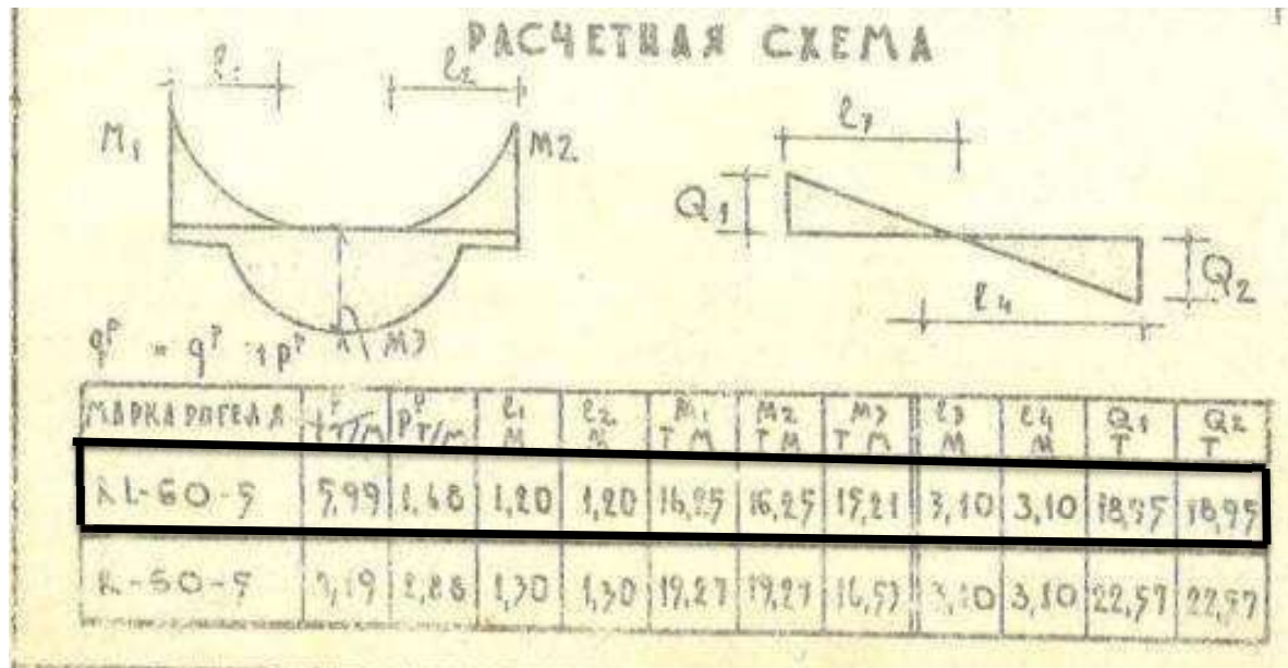
Rygių (rėmsijų) RL-60-5 skaičiuojamoji schema ir skaičiuotinė laikomoji galia pagal [3.1.9] katalogą
