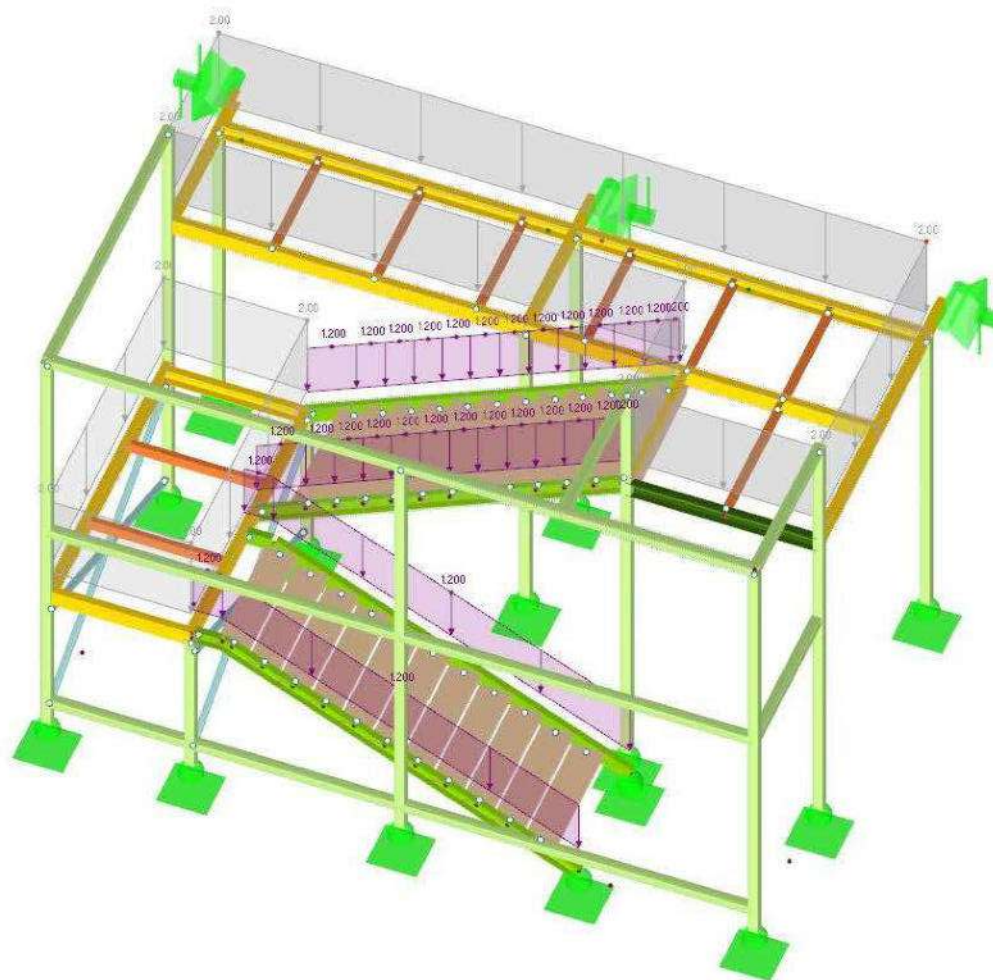
4.27 pav. Naudojimo aprova (LC3)
