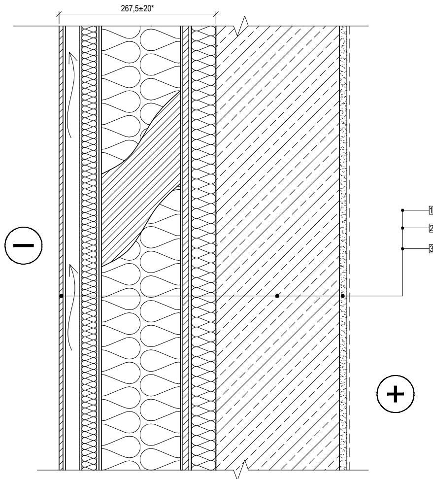
Sienos detalė SN-1 M1:5
