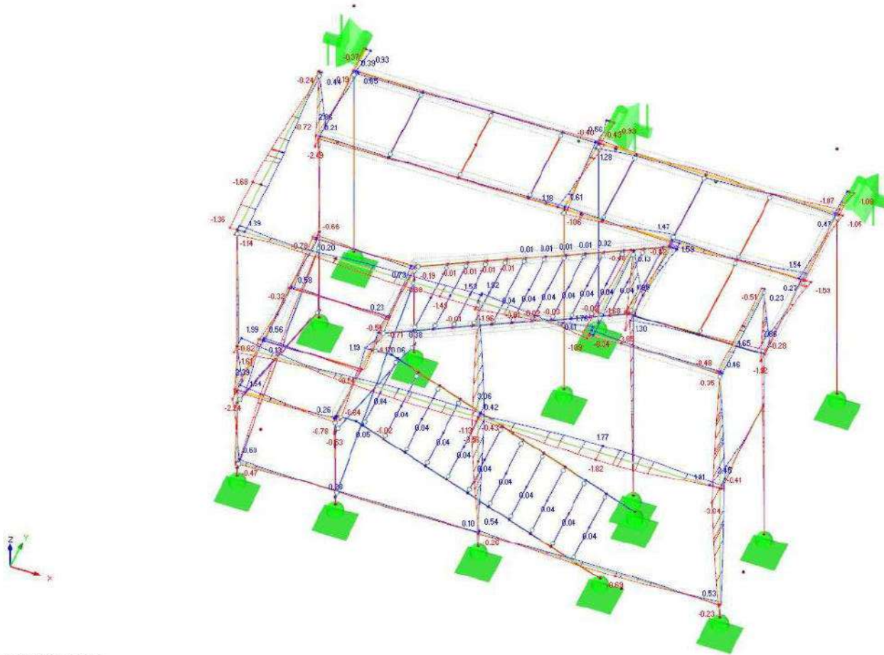
4.32 pav. Konstrukcijos lenkimo momentai Mz (ULS)
