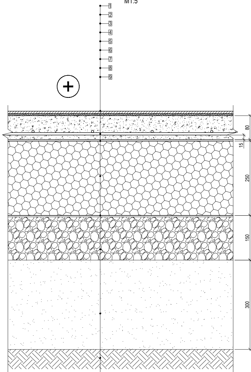
Grindų GR-1.3 detalė M1:5
