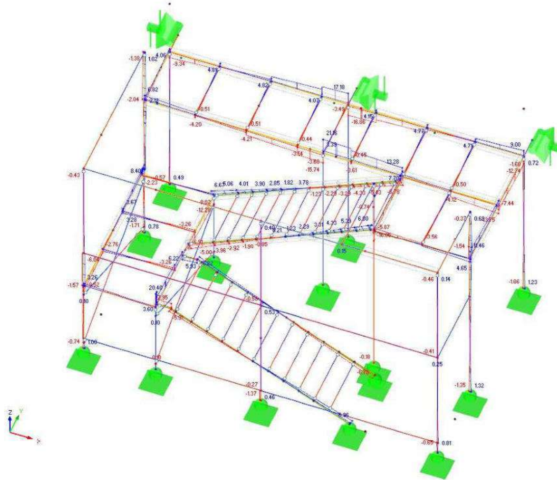
4.33 pav. Konstrukcijos skersinės jėgos Vz (ULS)
