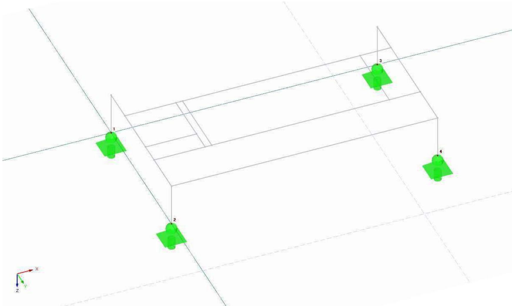
4.15 pav. Atraminių taškų schema
