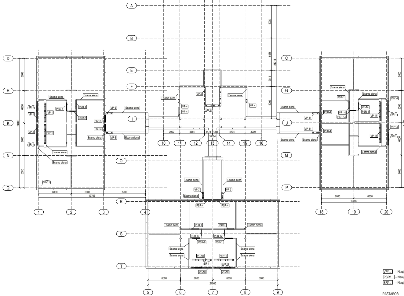
PSR sių planas 2a. 1:200
