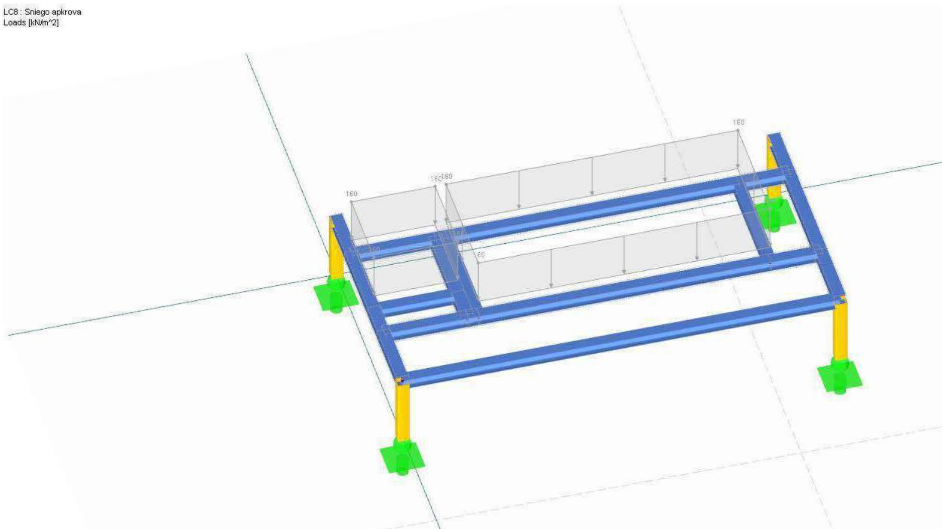
4.6 pav. Sniego apkrova ant ŠVOK įrenginių (LC3)
