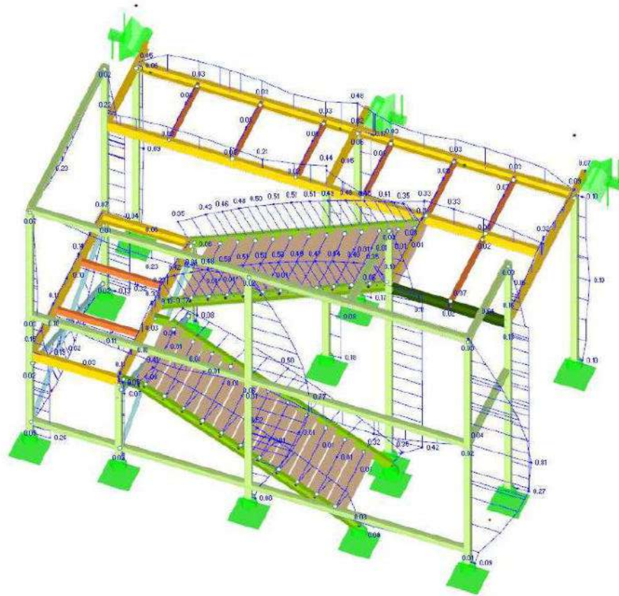
4.28 pav. Konstrukcijos išnaudojimo koeficientai (ULS)
