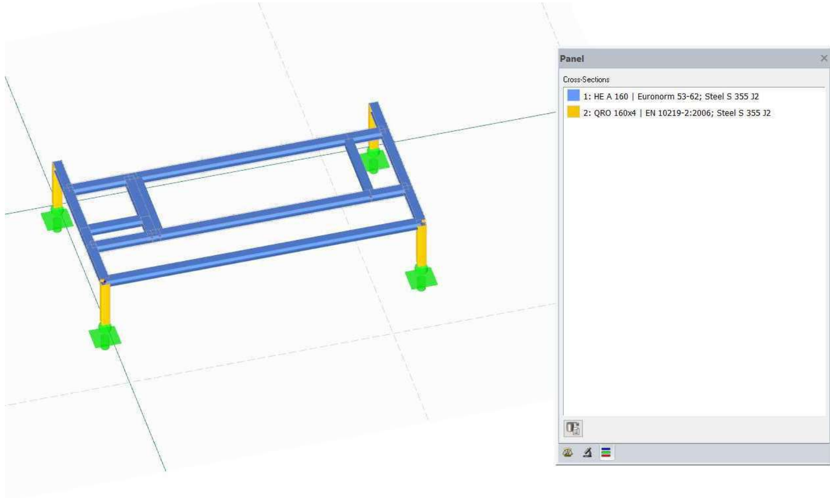
4.4 pav. Skaičiuojamoji schema ir profiliai
