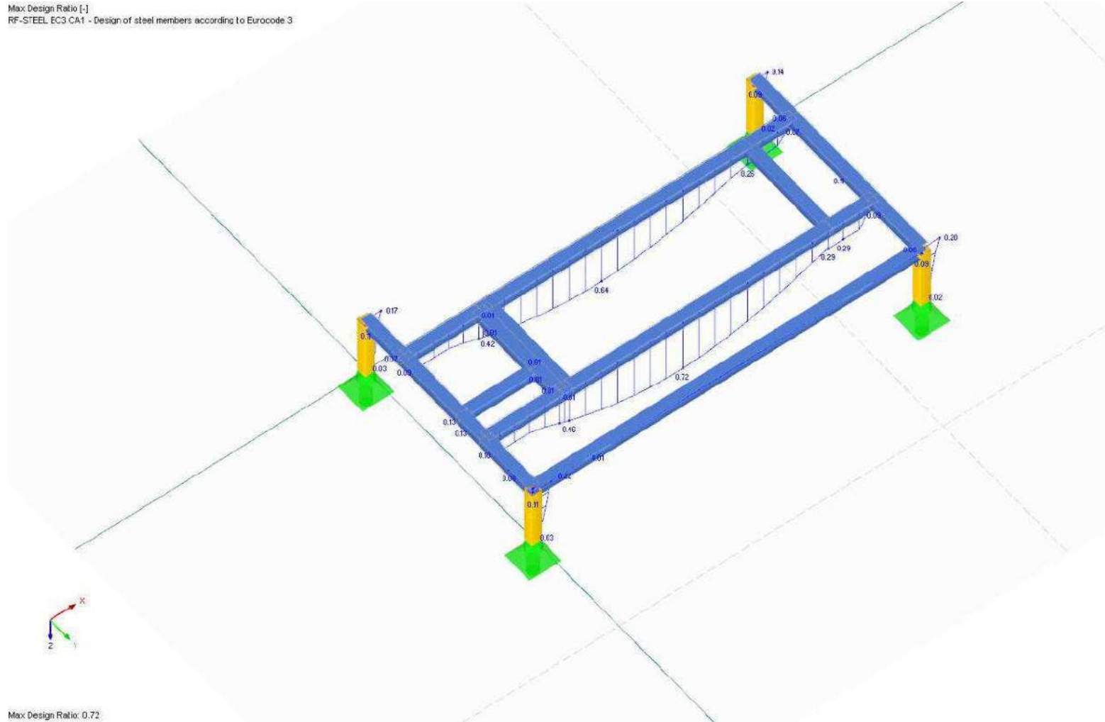
4.8 pav. Konstrukcijų išnaudojimo koeficientai
