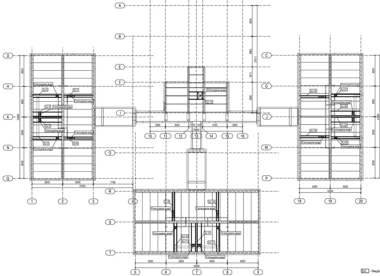
Perdangos planas 2a. 1:200
