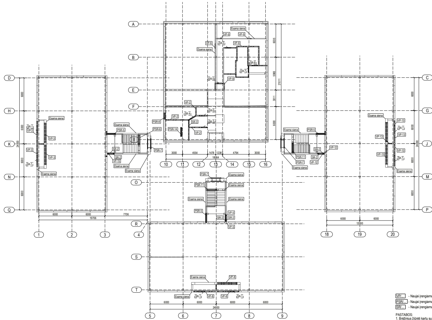
PSR sijų planas 1a. 1:200
