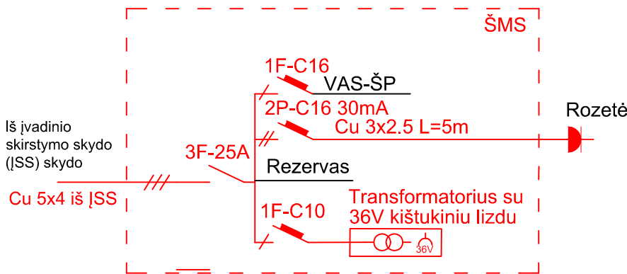
Šilumos mazgo skydo funkcinė schema
