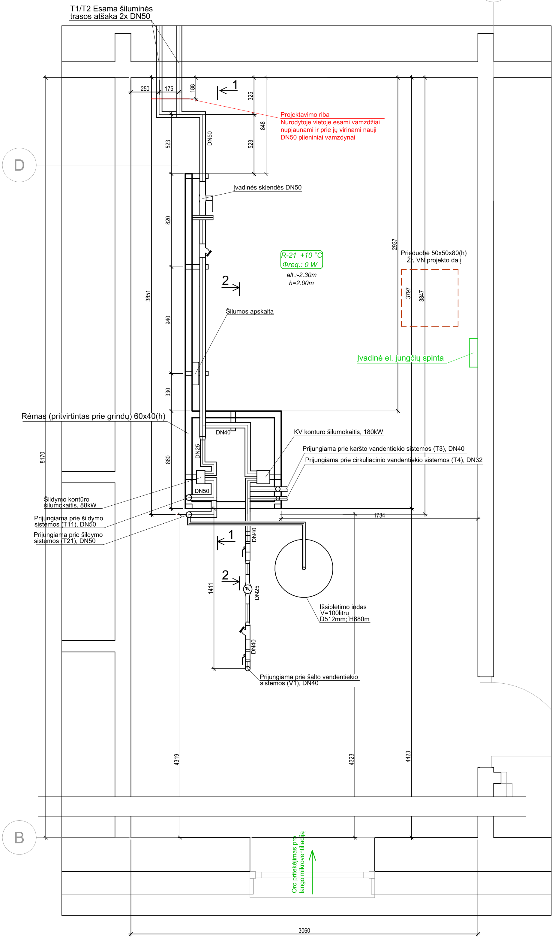
Šilumos punkto (Nr.2) planas, M1:20
