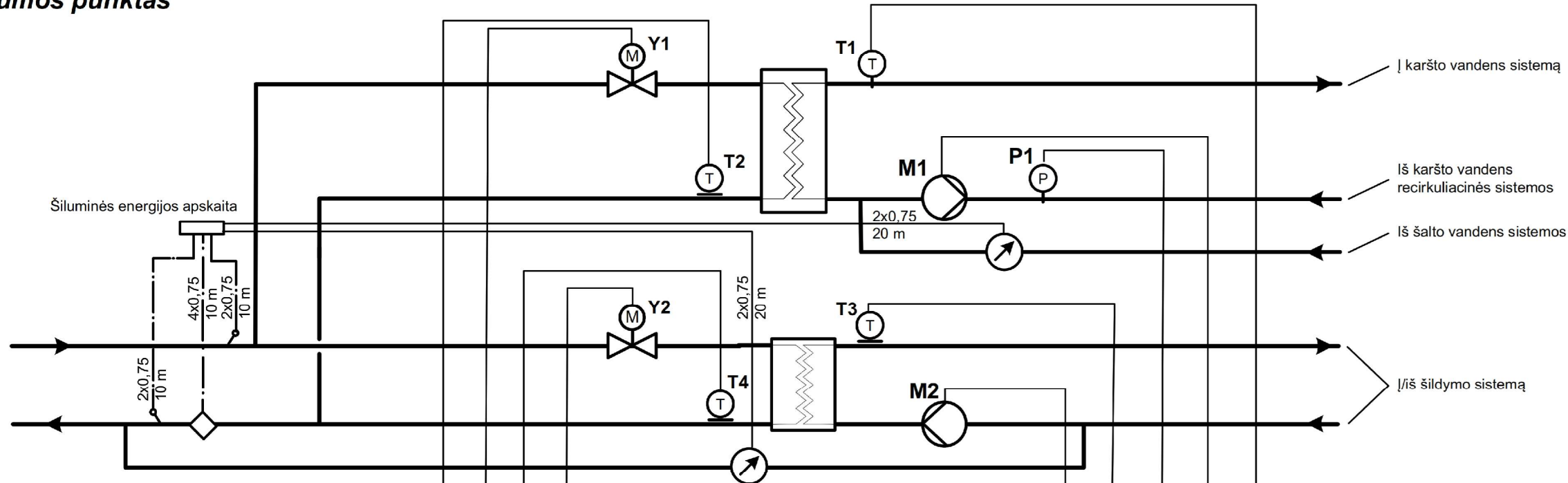
Šilumos punkto automatizavimo funkcinė schema
