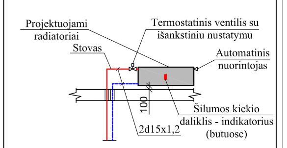
PROJEKTUOJAMA LAIPTINIŲ RADIATORIŲ PAJUNGIMO PRIE STOVŲ PRINCIPINĖ SCHEMA
