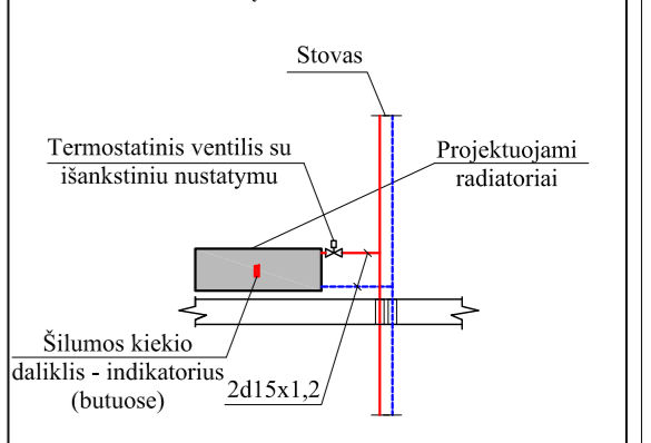
PROJEKTUOJAMA 5 AUKŠTO RADIATORIŲ PAJUNGIMO PRIE STOVŲ PRINCIPINĖ SCHEMA
