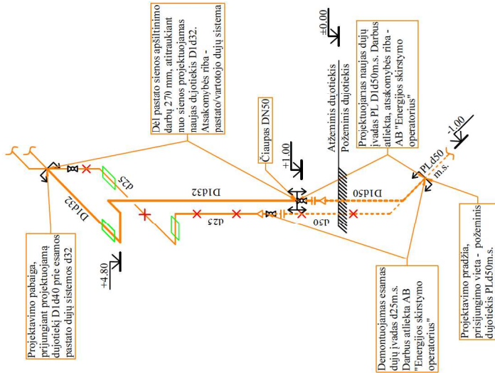
AKSONOMETRINĖ SCHEMA
