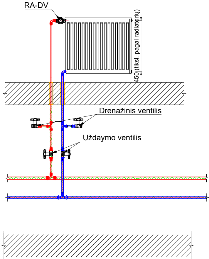
LAIPTINĖS STOVO APRIŠIMAS
