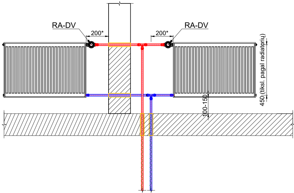
KETVIRTO AUKŠTO DVIGUBO STOVO ĮRENGIMO SCHEMA
