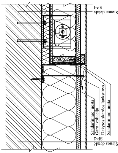
SP-1 IR SP-2 JUNGIMAS M 1:10
