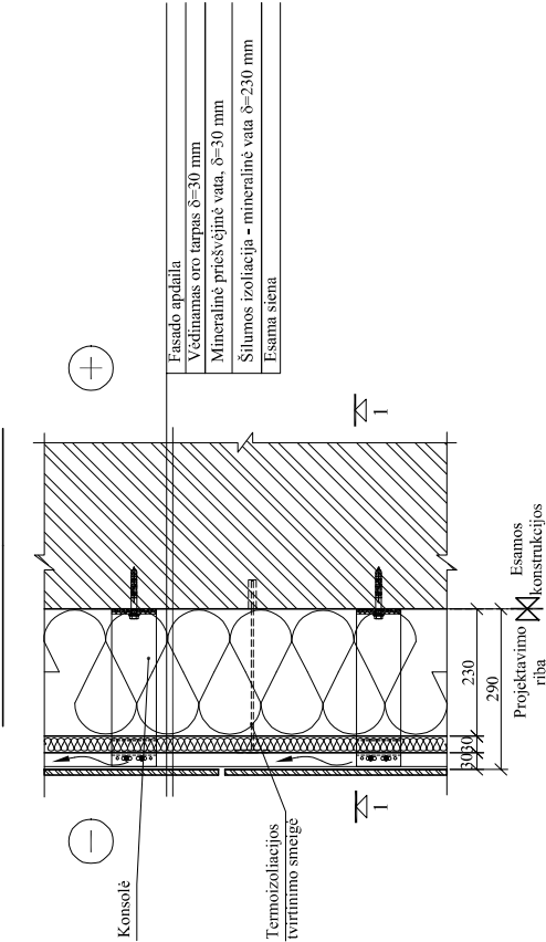
SIENOS DETALĖ SP-2 M 1:10
