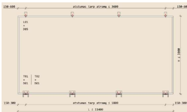
Pav. A Principinė skydo atrėmimo/ tvirtinimo schema
