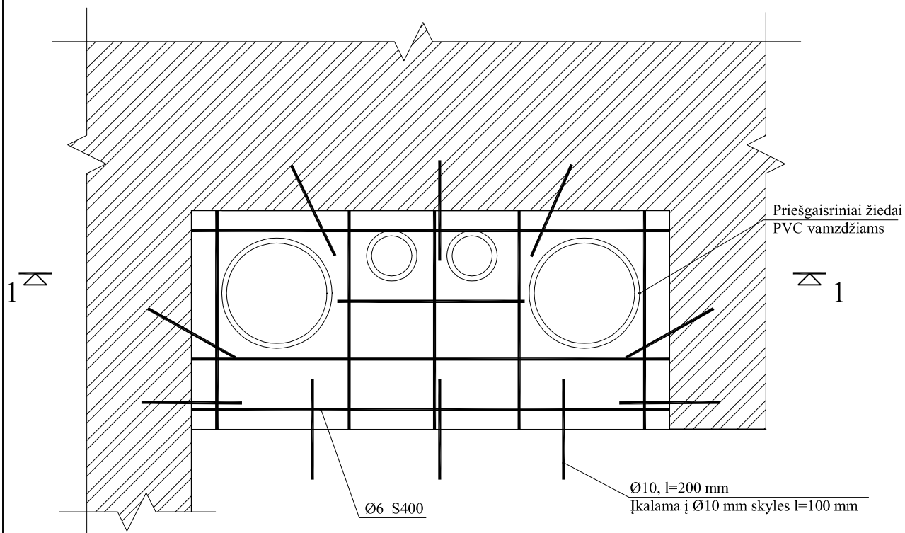
PJŪVIS 1-1
