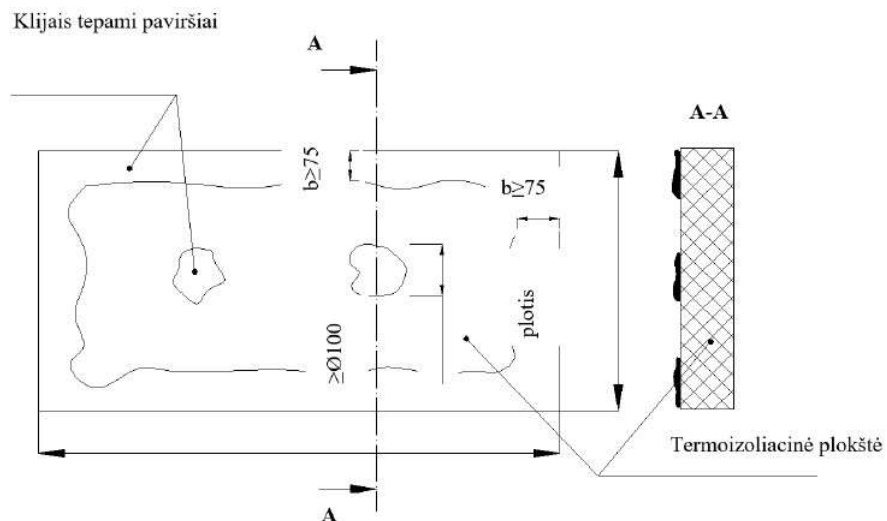
5 pav. Termoizoliacinės plokštės padengimas klizais (klizų kiekis - padengiama ne mažiau 40% plokštės ploto)
