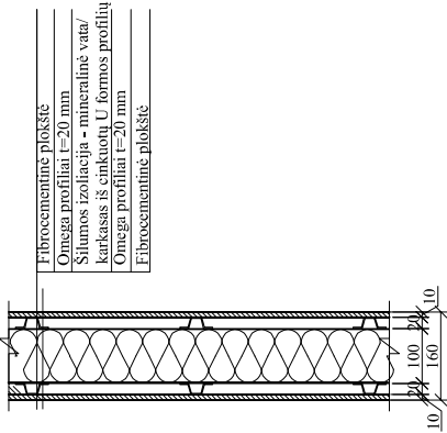
SIENOS DETALĖ SP-6 M 1:10
