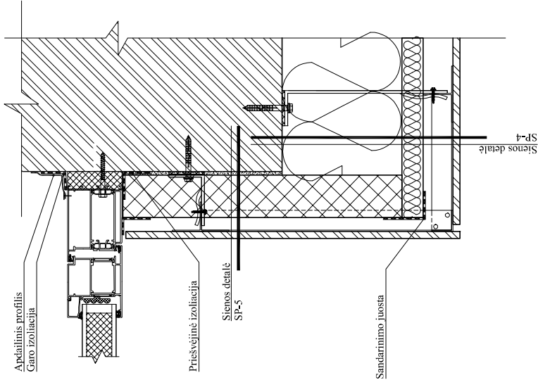
PRINCIPINĖ LAUKO DURŲ ŠONINIO ANGOKRAŠČIO ĮRENGIMO DETALĖ M 1:5
