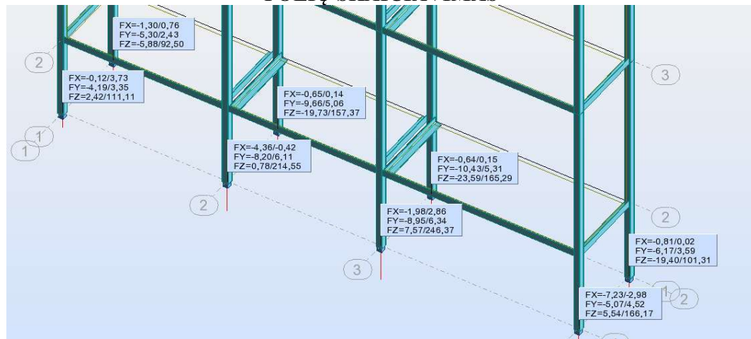
Pav.4 Atraminēs reakcijas
