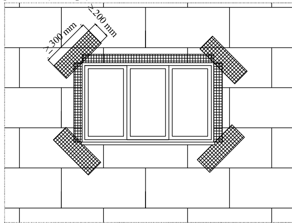
5 pav. Termoizoliacinės plokštės padengimas klizais (klizų kiekis - padengiama ne mažiau 40% plokštės ploto)
