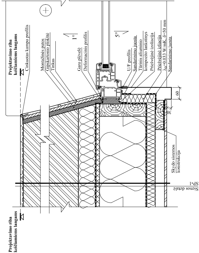
BUTŲ LANGŲ ŠONINIO ANGOKRAŠČIO ĮRENGIMO DETALĖ M 1:5
