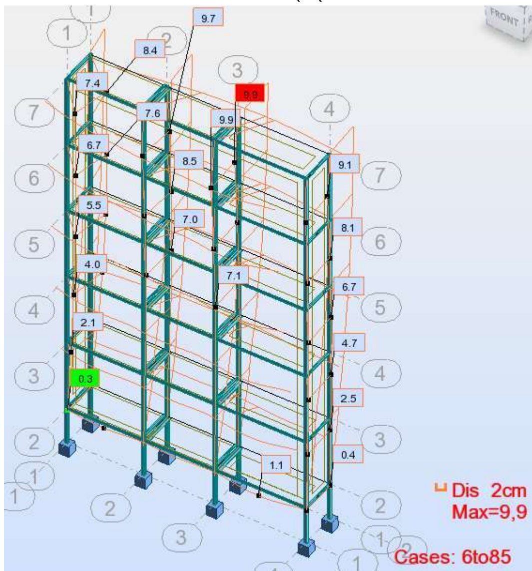
Pav. 2 konstrukcijų deformacijos.
