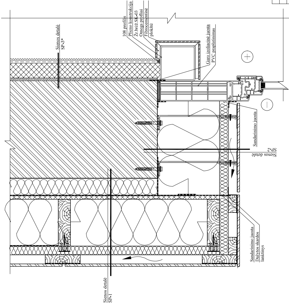
BALKONŲ STIKLINIMO ŠONINIO ANGOKRAŠČIO ĮRENGIMO DETALĖ M-1 M 1:5
