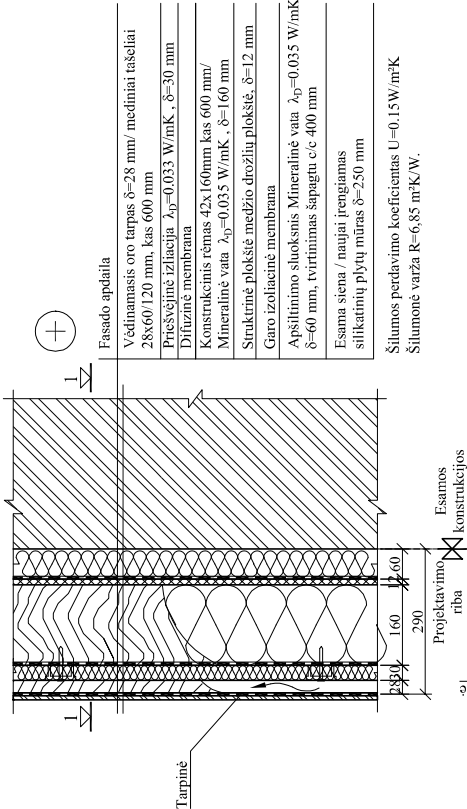
SIENOS DETALĖS SP-1 M 1:10
