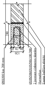
PIŪVIS D-D M 1:10
