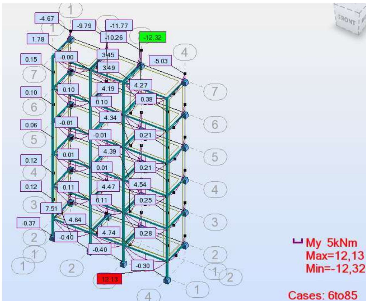
Pav. 3 Konstrukcijų lenkimo momentų diagramos
