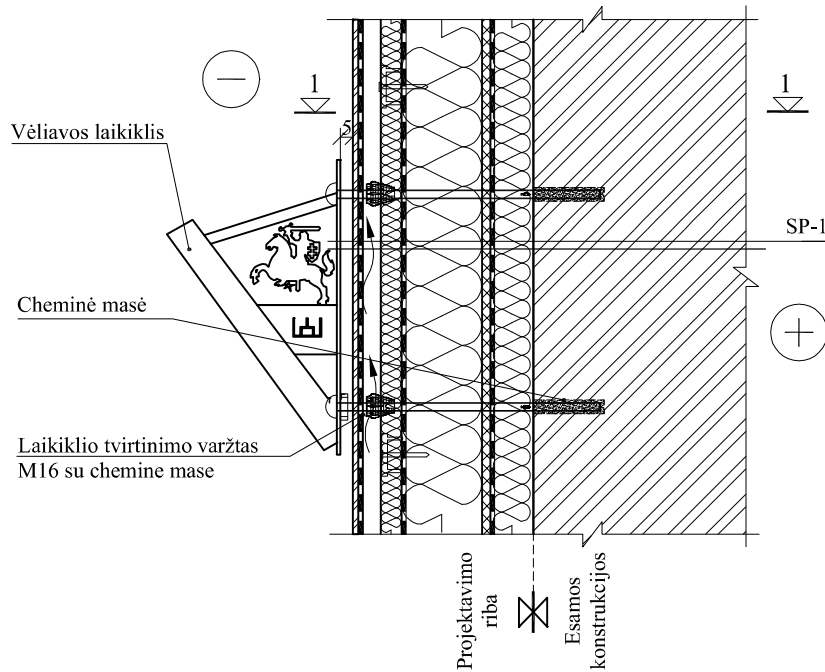
PJŪVIS 1-1 M 1:10
