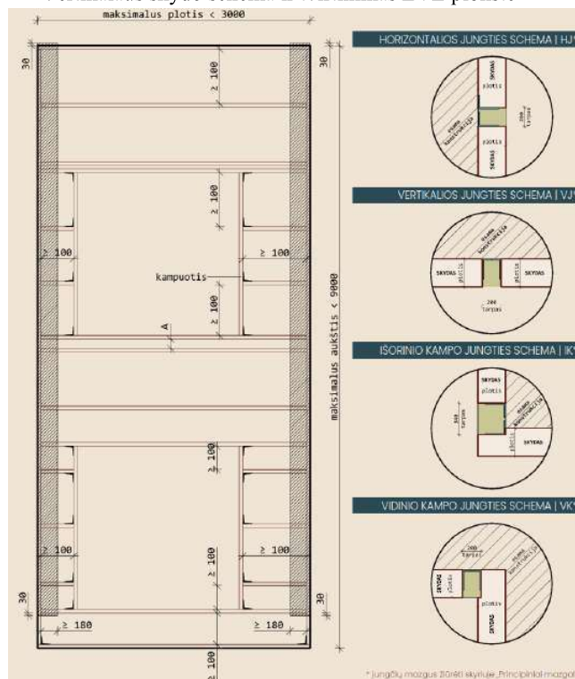
Vertikalaus skydo schema ir tvirtinimas LVL plokštė
