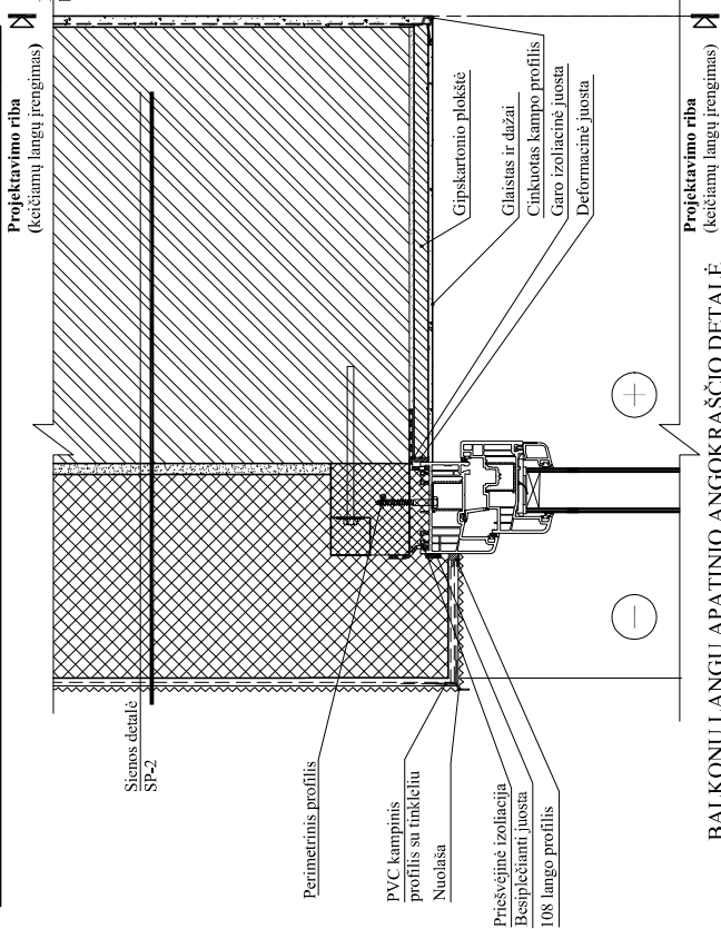
LANGŲ BALKONŲ VIDUJE VIRŠUTINIO ANGOKRAŠČIO ĮRENGIMO DETALĖ M 1:5
