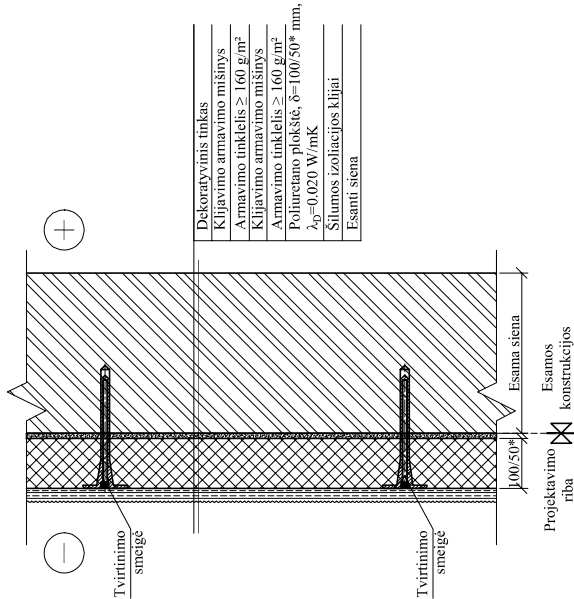
SIENŲ DETALĖ SP-3/SP-3* M 1:10
