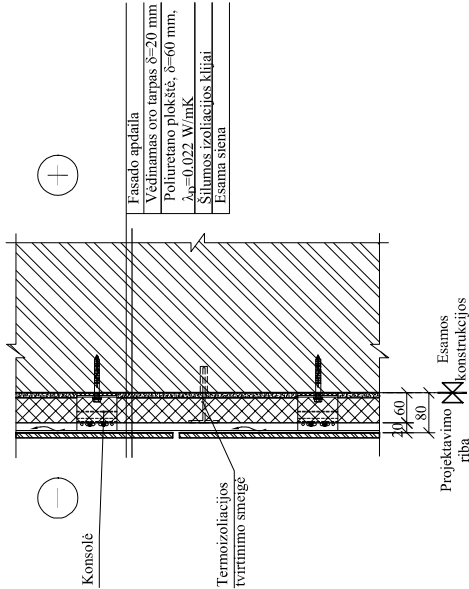
SIENOS DETALĖ SP-5 M 1:10
