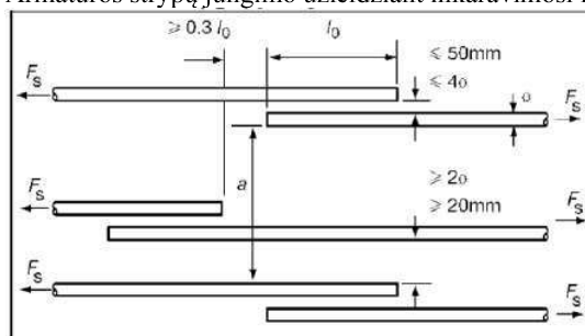
1 pav. Armatūros strypai jungiami užleidžiant
