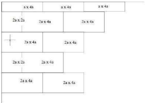
3 pav. Antrojo termoizoliacinio sluoksnio klojimo schema
