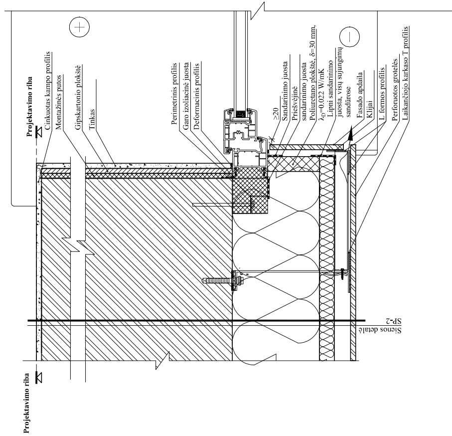
LAIPTINĖS LANGŲ ANGOKRAŠČIO ĮRENGIMO DETALĖ M 1:5
