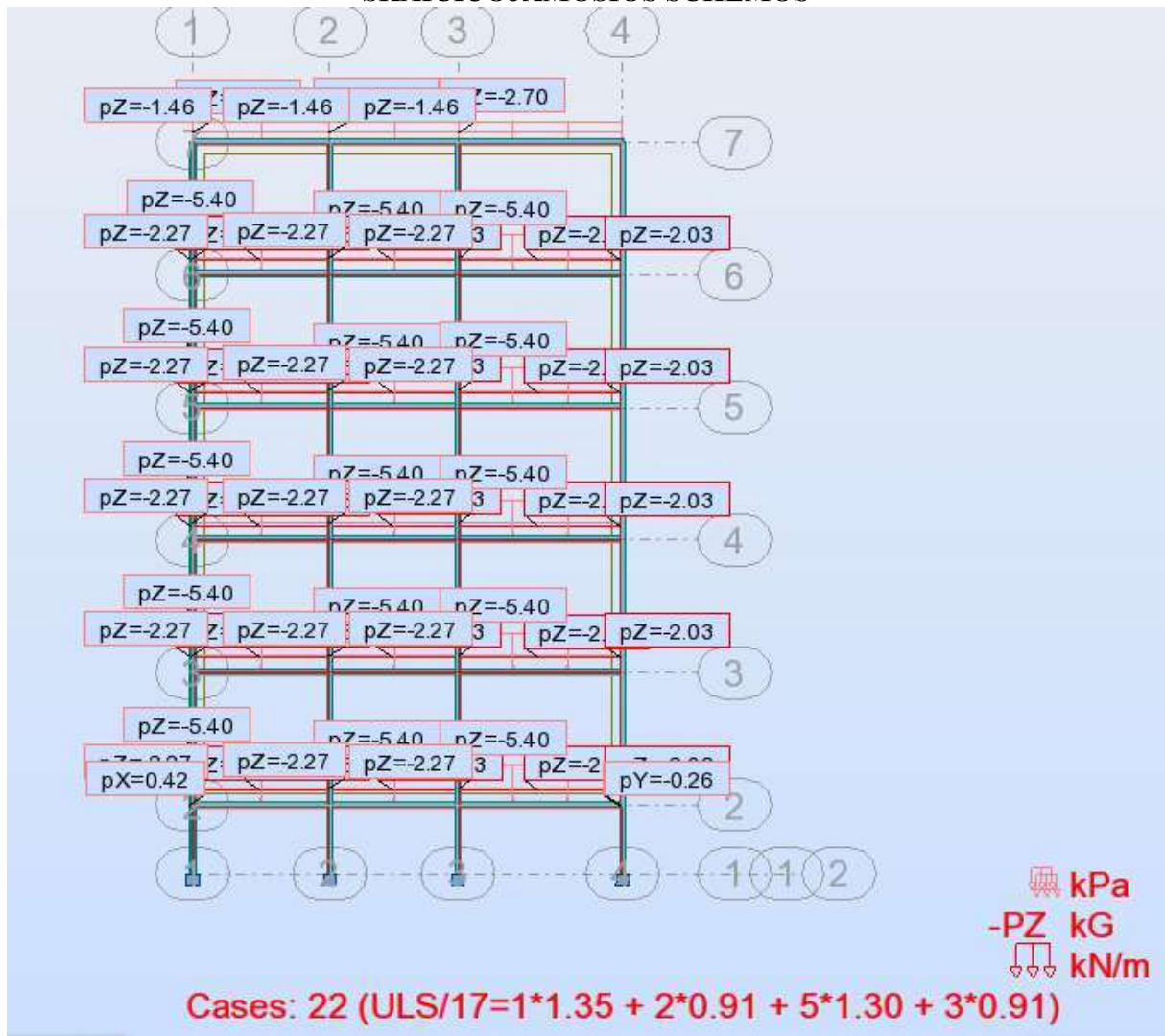
Pav. 1 balkonų konstrukcijų skaičiuojamoji schema
