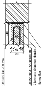
PIŪVIS E-E M 1:10
