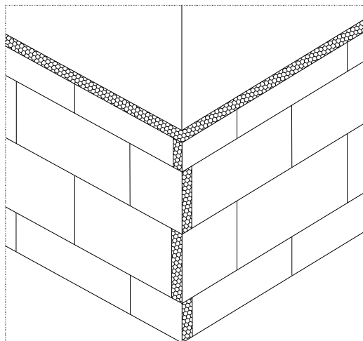
1 pav. Termoizoliacinių plokščių išdėstymas pastato kampuose.
