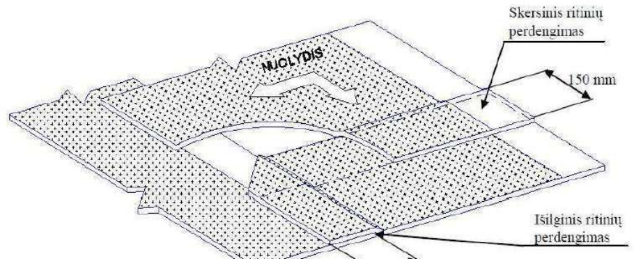
7 pav. Ritinių dangų perdengimas
