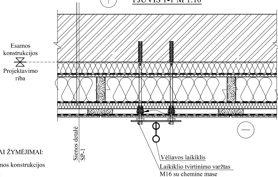
PJŪVIS 1-1 M 1:10
