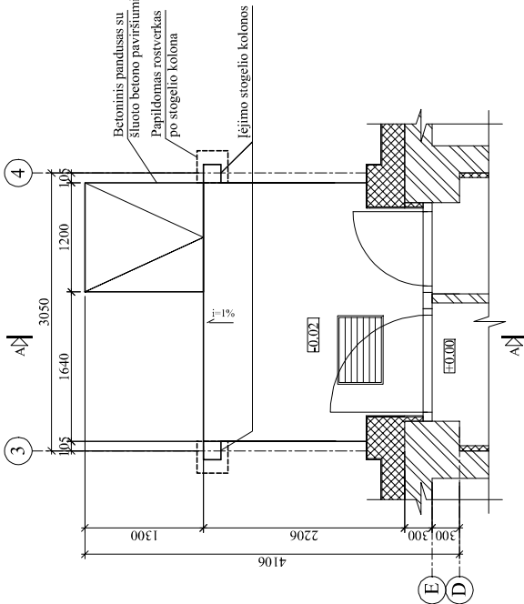
I LAIPTINĖS ĮĖJIMO AIKŠTELĖS PLANAS M 1:50
