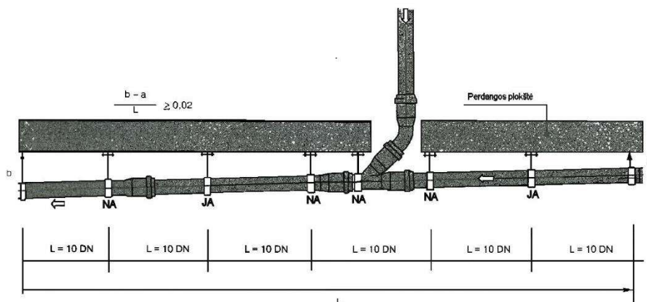
7 pav. Pakabinto vamzdyno tvirtinimas
