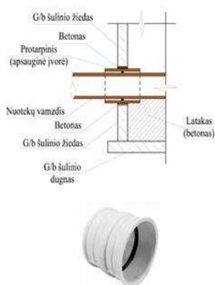
14 pav. Vamzdžio pajungimas G/B šuliniuose
