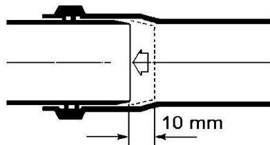
5 pav. Vamzdžių sujungimas
