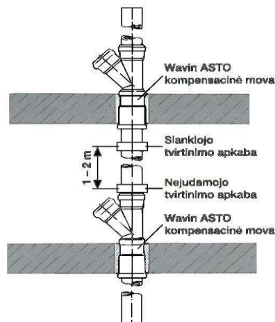
6 pav. Vertikalaus stovo tvirtinimas
