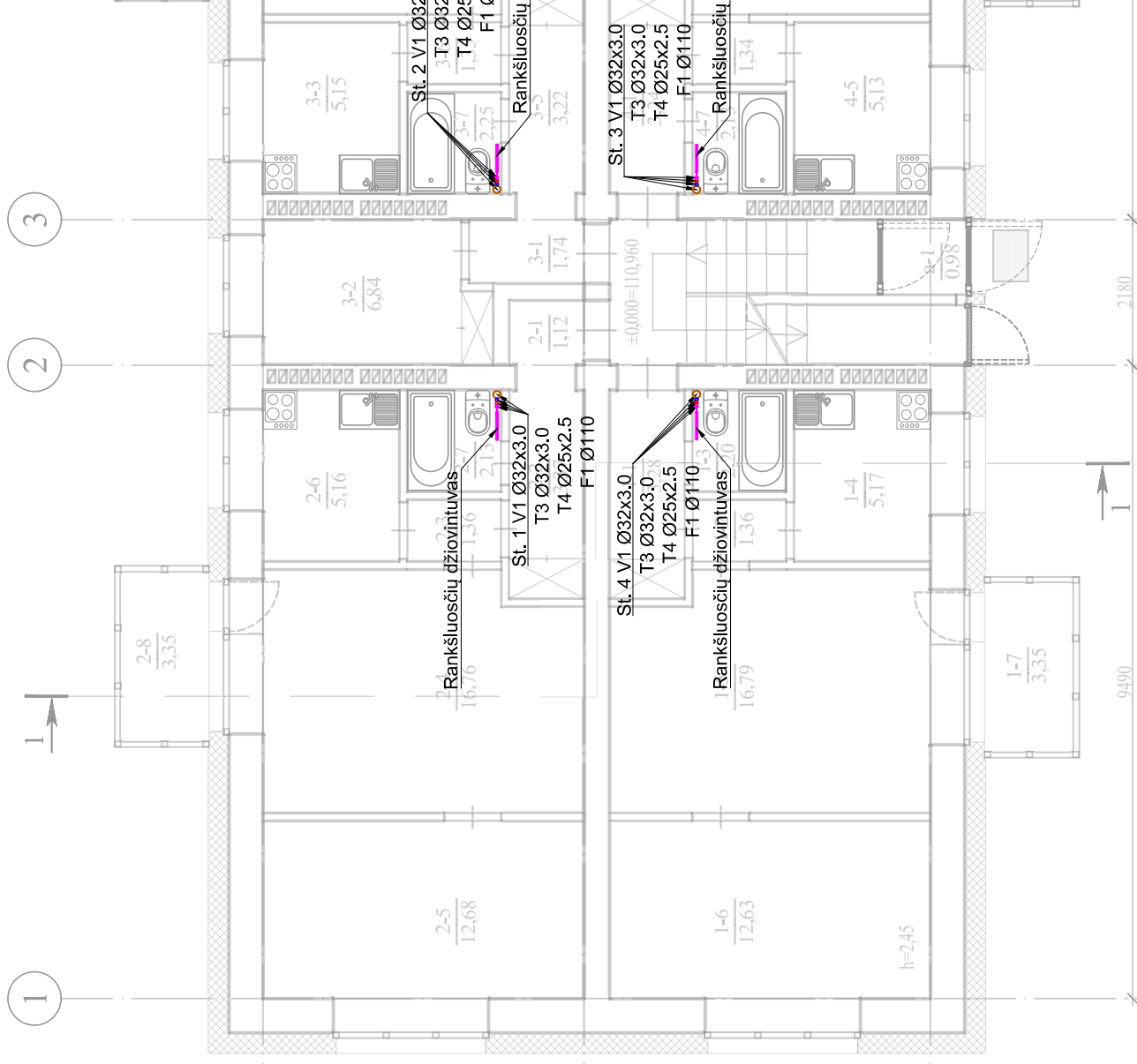
RANKŠLUOSČIŲ DŽIOVINTUVO PAJUNGIMO PRINCIPINĖ SCHEMA
