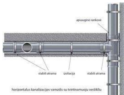
10 pav. Iš dalies įmūrijamo vamzdyno montavimas
